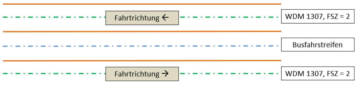
Abbildung 35: Modellierung eines durch Leitplanke getrennten Busfahrstreifens
