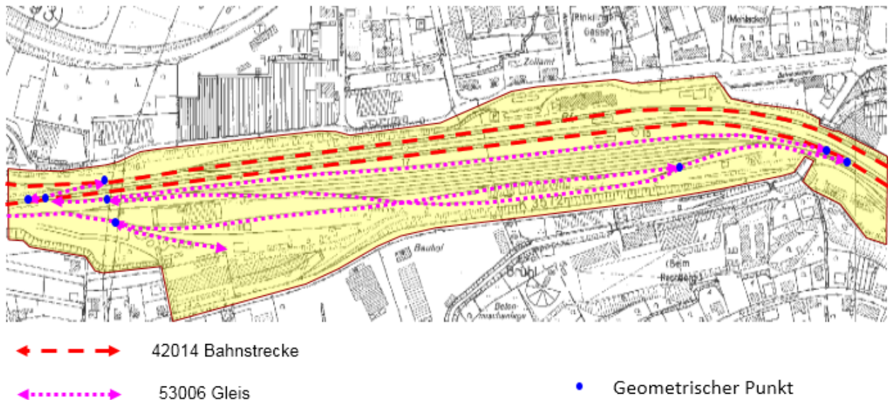
Abbildung 54: Modellierung von Gleisen
