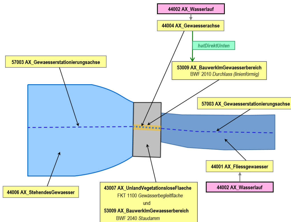
Abbildung 57: Modellierung von Wasserlauf unter Staudamm in linienförmigem Durchlass
