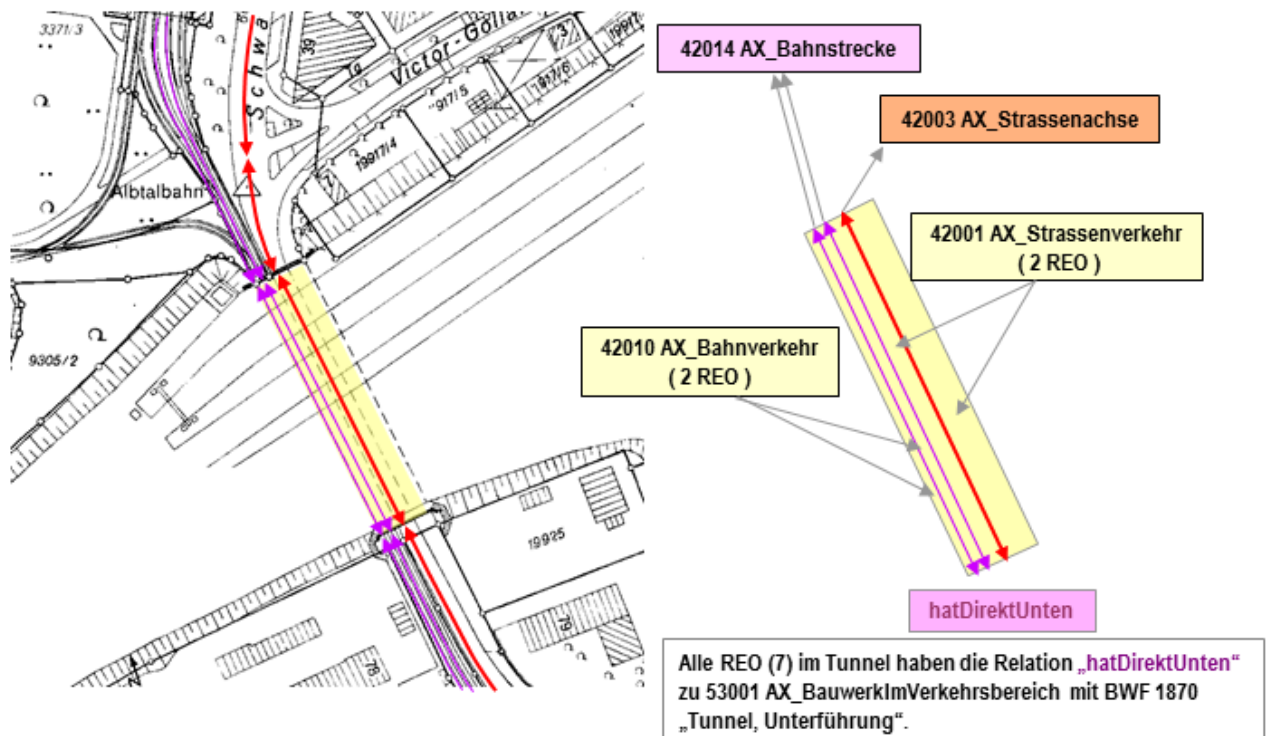
Abbildung 52: Modellierung eines flächenförmigen Tunnels mit mehreren Objekten
