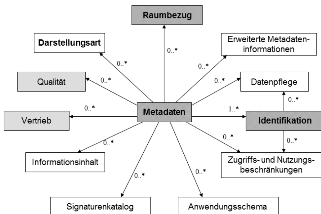
Abbildung 70: ISO-Hauptklassen
