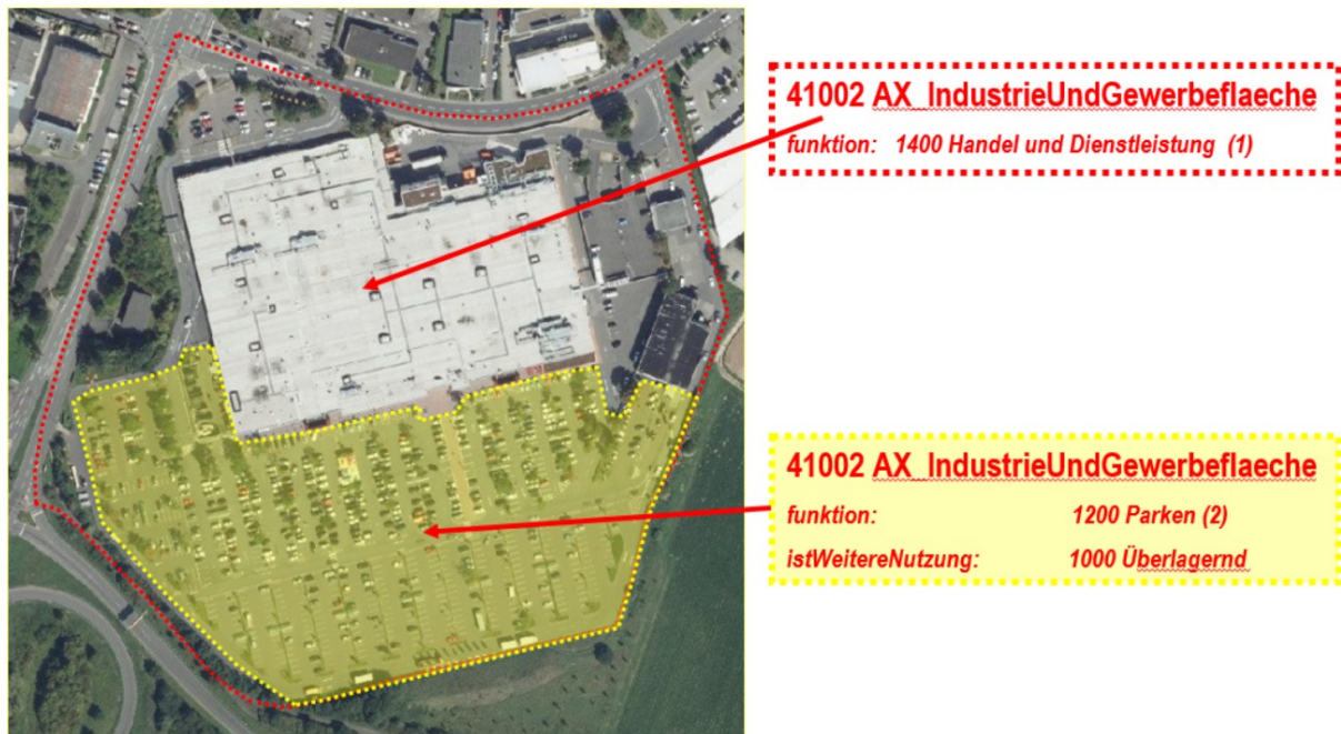
Abbildung 16 Anwendung des Attributes „istWeitereNutzung“ bei einem Kundenparkplatz
