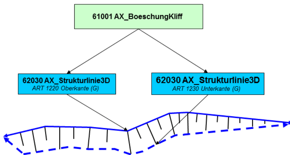
Abbildung 60: Modellierung einer Böschung mit Strukturlinien3D
