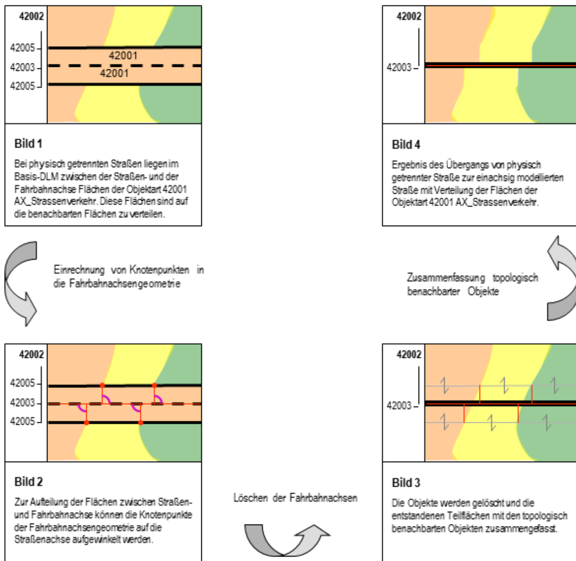
Abbildung 22: Flächenaufteilung beim Übergang von physisch getrennten zu einfach modellierten Straßen
