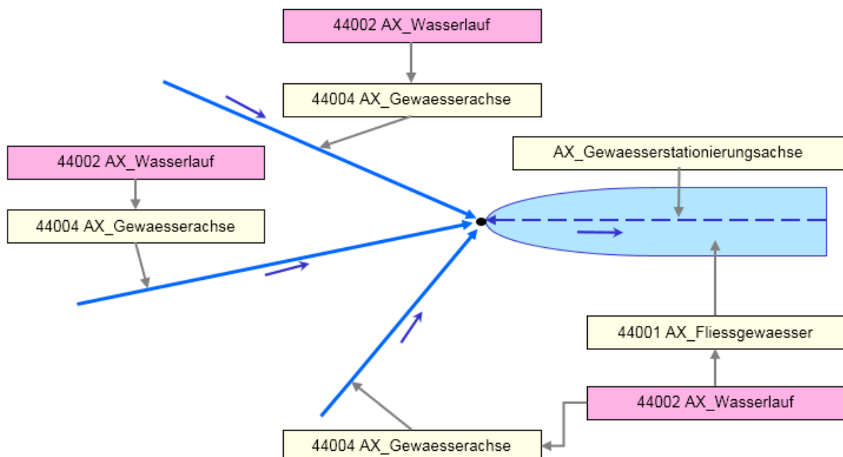
Abbildung 44: Modellierung von Wasserläufen unter Beachtung der Fließrichtung
