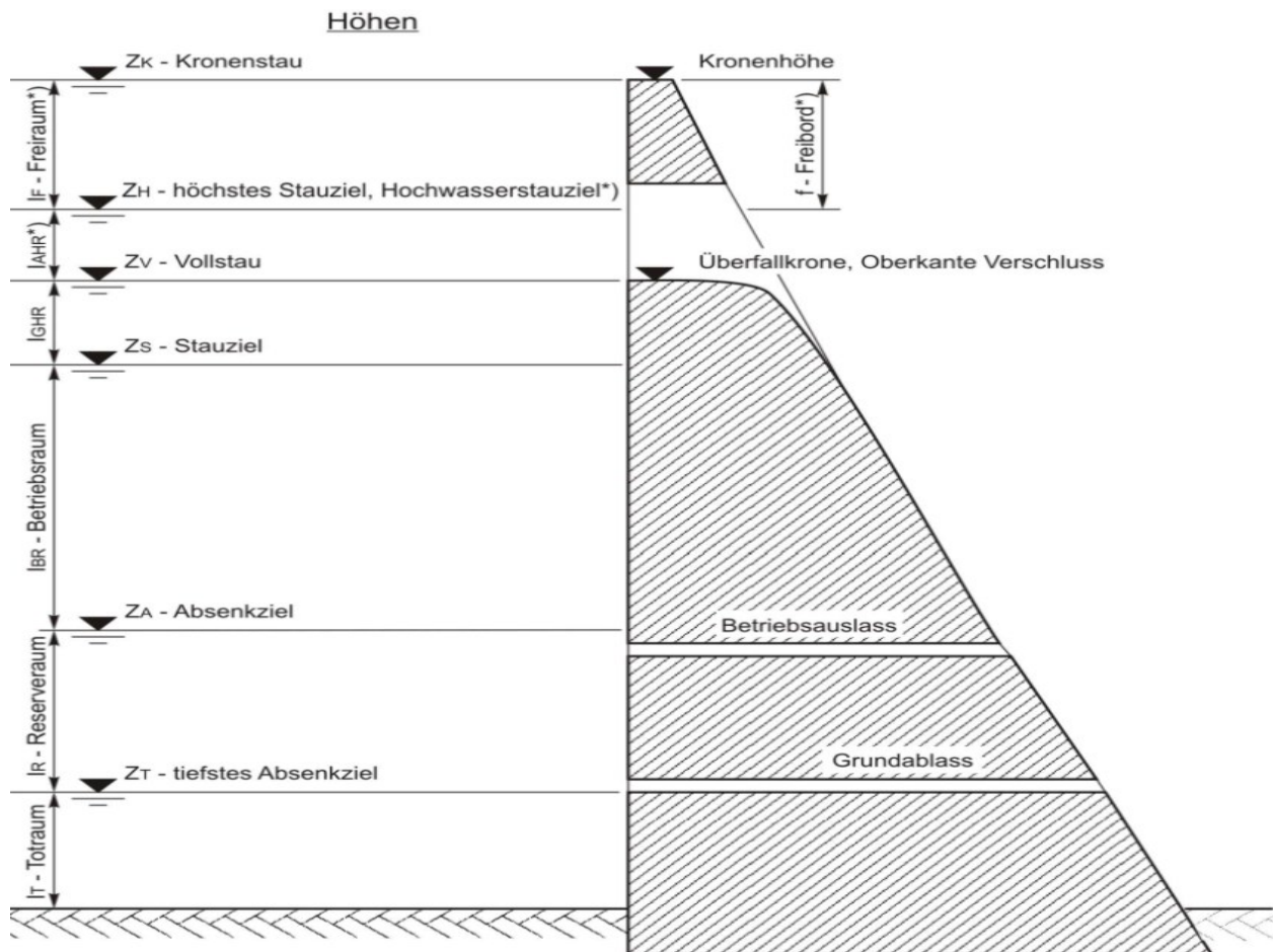
Abbildung 43: Schematische Darstellung der Stau- und Absenkziele bei einem Stausee
