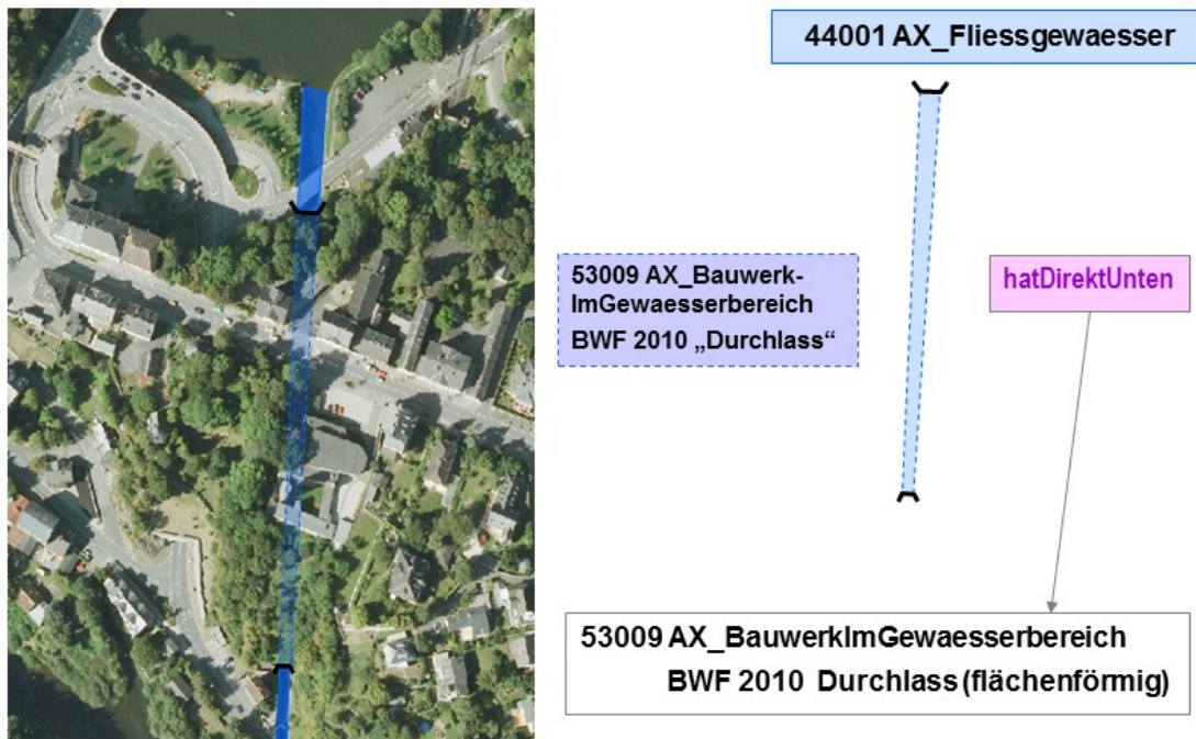
Abbildung 56: Modellierung eines flächenförmigen Durchlasses mit einem flächenförmigen Objekt
