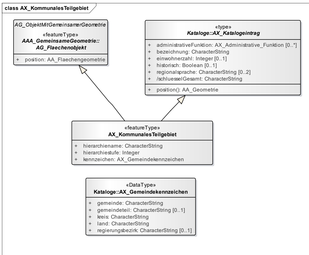
Abbildung 68: Klassendiagramm AX_KommunalesTeilgebiet
