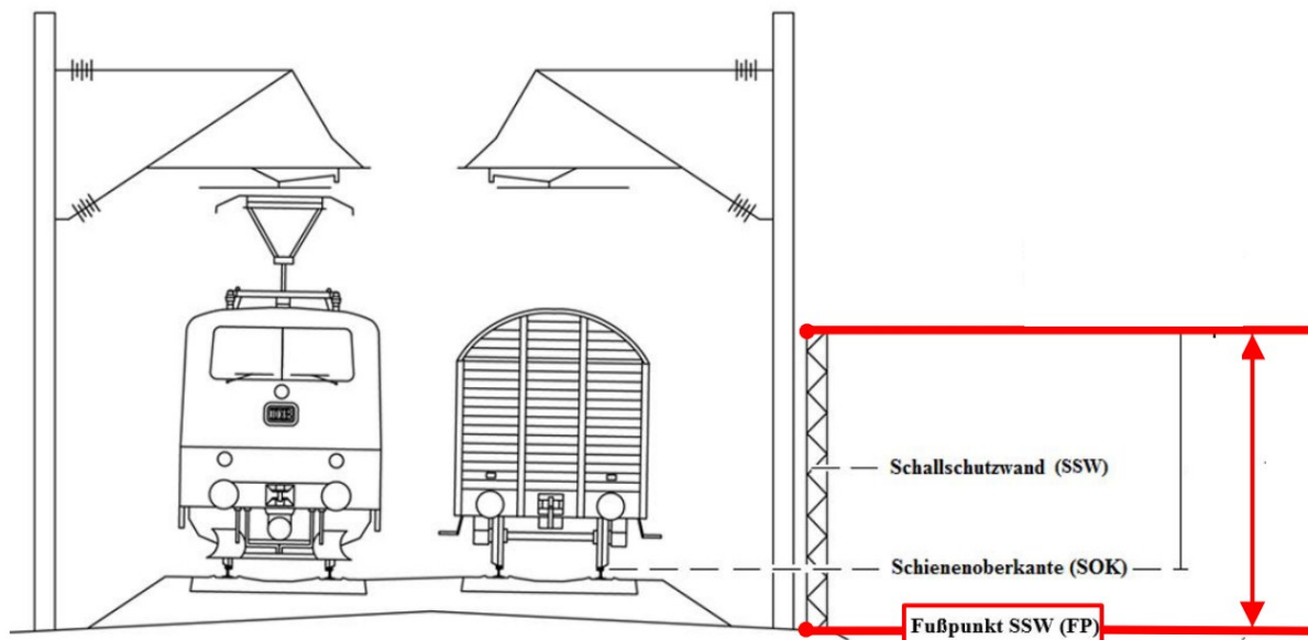
Abbildung 47: Höhenbezugspunkte für die Erhebung von Lärmschutzwänden)
