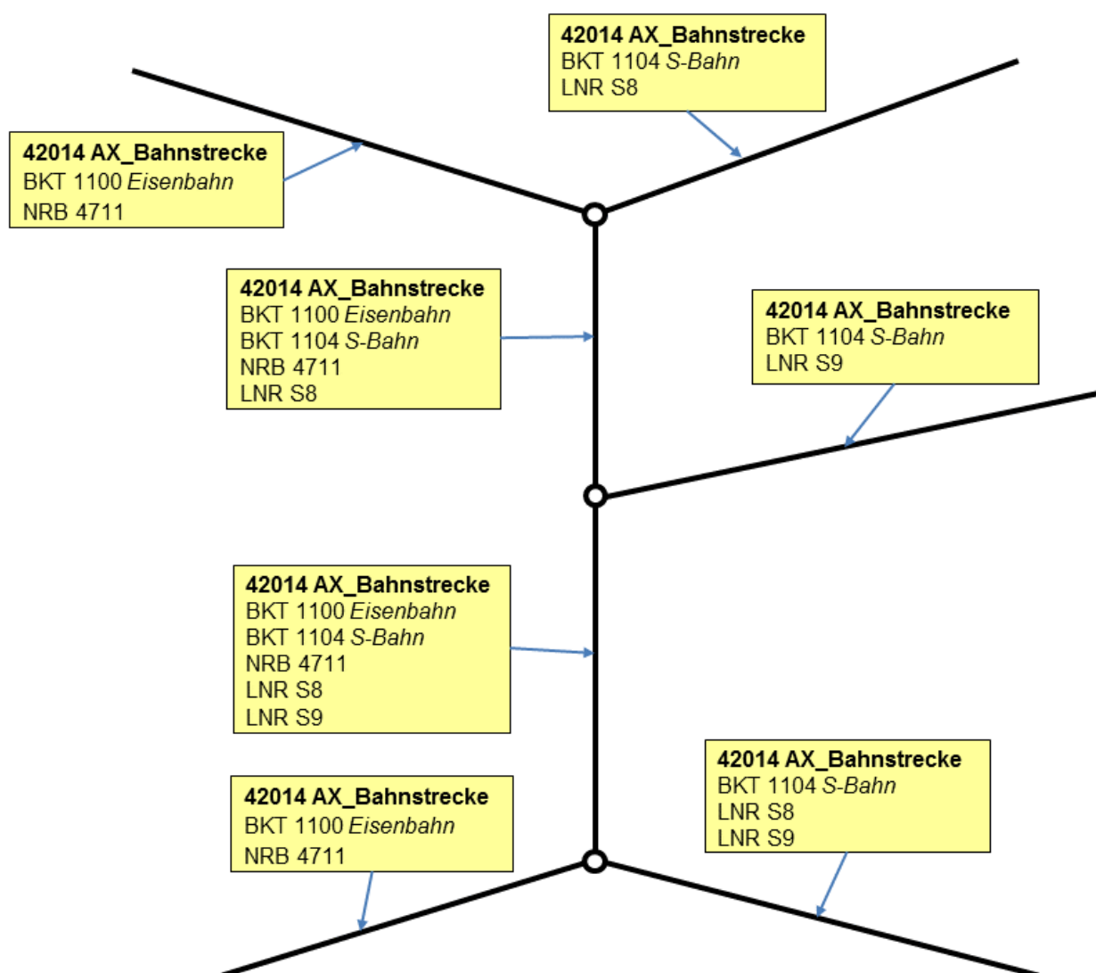
Abbildung 41: Modellierung von Bahnstrecken mit Strecken- und Liniennummern
