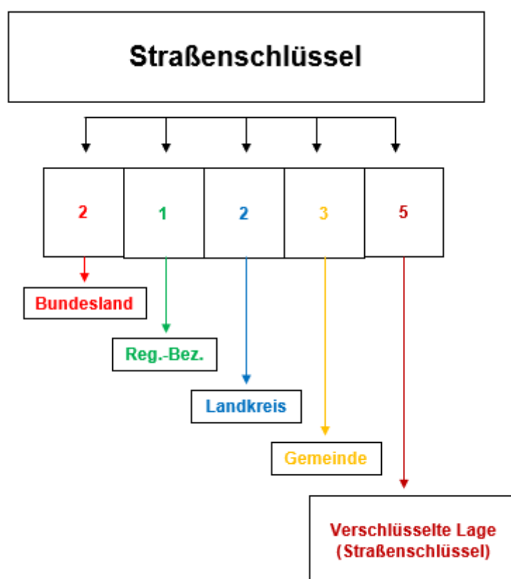
Abbildung 36: Zusammensetzung des 13-stelligen Straßenschlüssels (STS)
