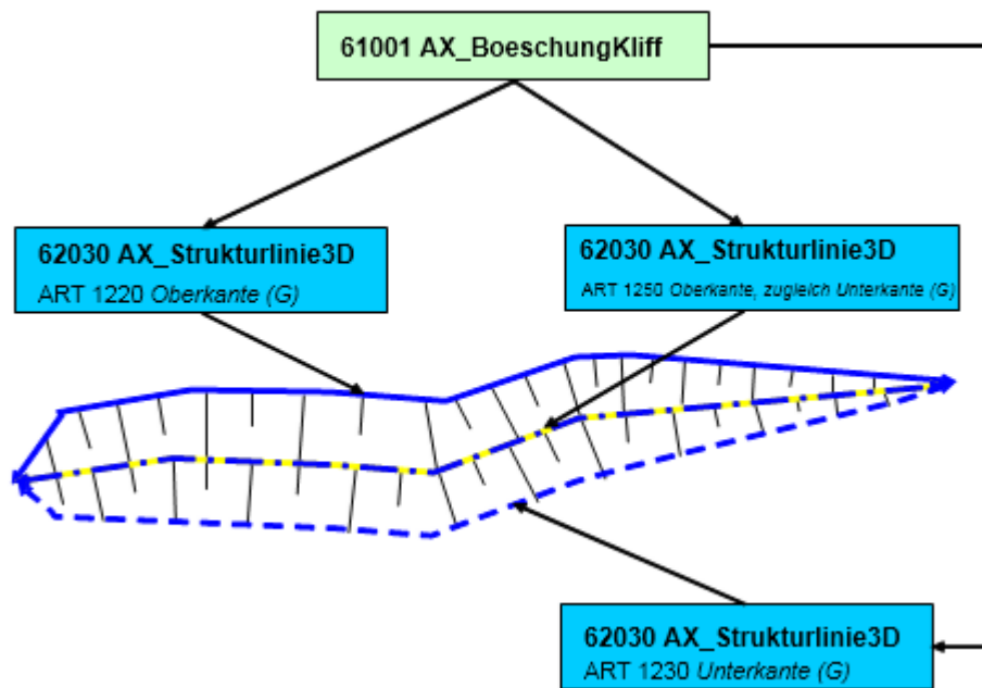
Abbildung 61: Modellierung einer Böschung mit Strukturlinien3D und Gefällewechsel
