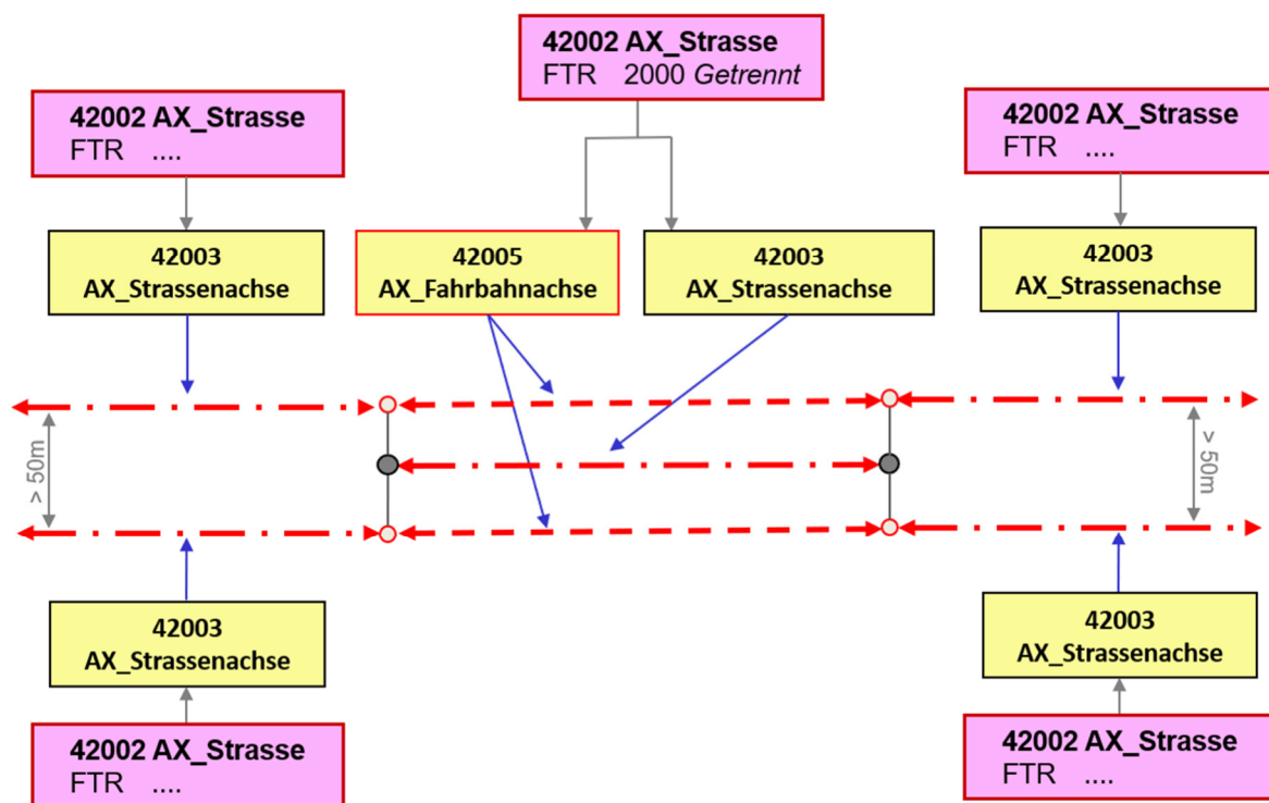
Abbildung 45: Modellierung eines „Wechsels“ physische Trennung in nicht-physische Trennung
