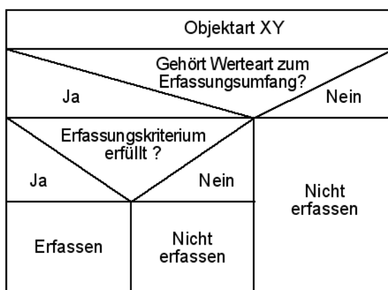
Abbildung 16: Objekterfassung bei Attributarten mit Multiplizität 1 bzw. 1..*
