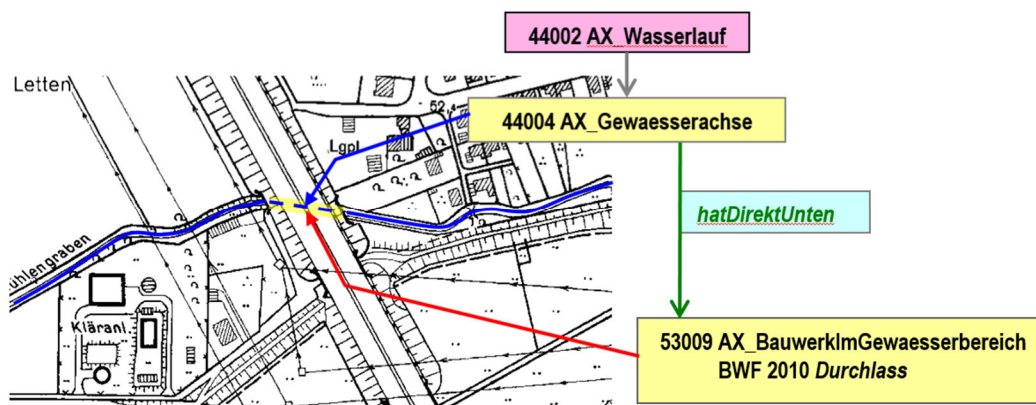
Abbildung 20: Beispiel für die Modellierung eines Durchlasses
