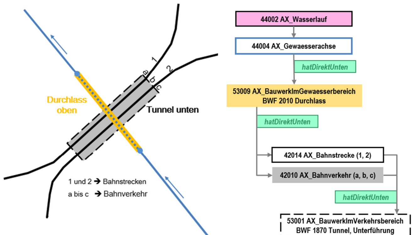
Abbildung 24: Vergabe der Relation „hatDirektUnten“ bei Durchlass über Tunnel
