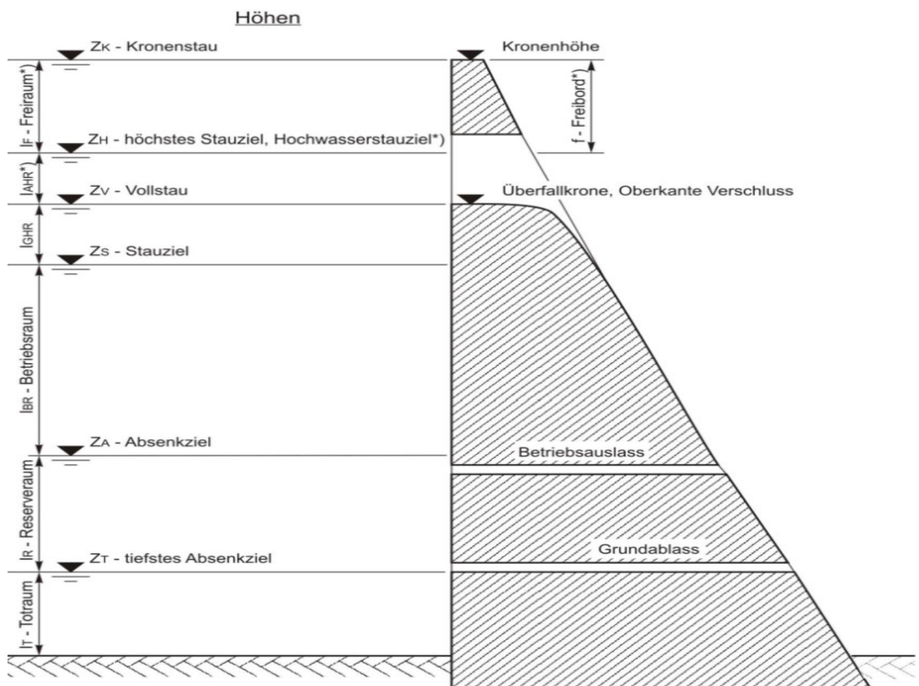
Abbildung 52: Schematische Darstellung der Stau- und Absenkziele bei einem Stausee
