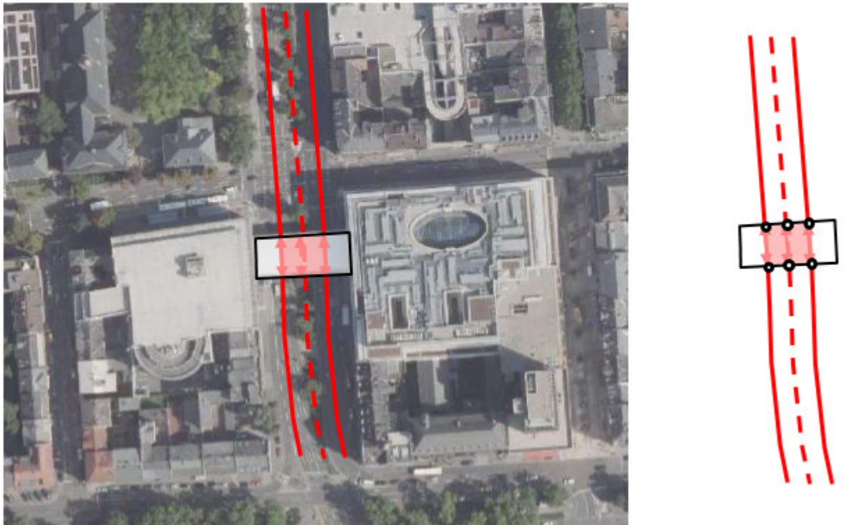
Abbildung 65: Modellierung einer flächenförmigen Durchfahrt
