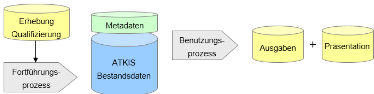
Abbildung 87: Übersicht zum Prozessablauf in ATKIS
