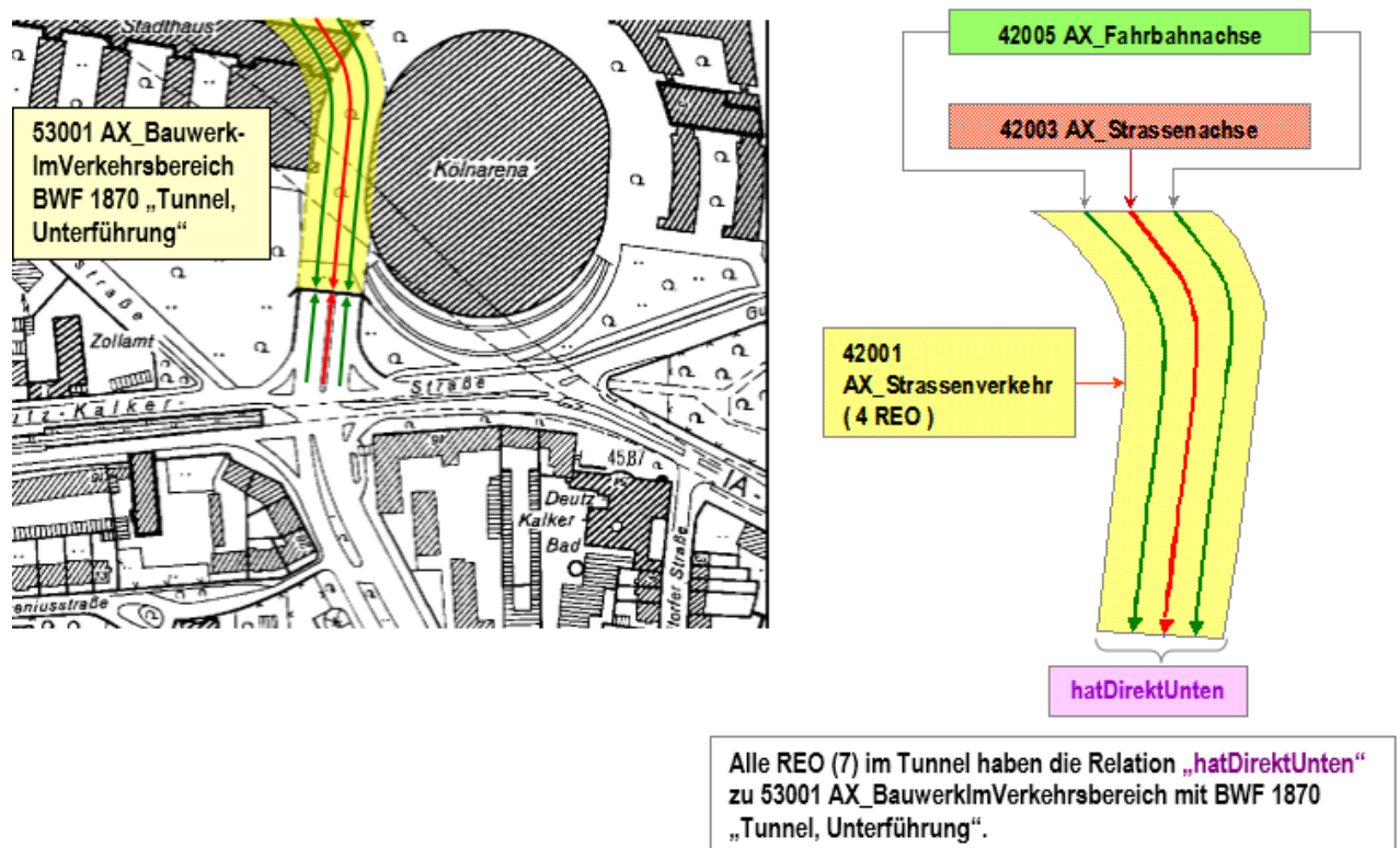
Abbildung 63: Modellierung eines flächenförmigen Tunnels mit mehreren Objekten
