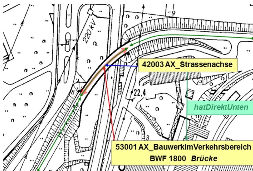
Abbildung 19: Vertikale Abbildung der Landschaft mit der Relation „hatDirektUnten“
