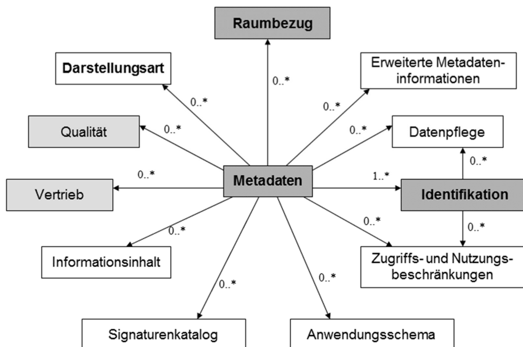
Abbildung 85: ISO-Hauptklassen
