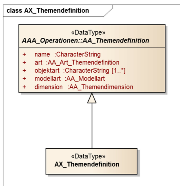
Abbildung 6: Klassendiagramm AX_Themendefinition
