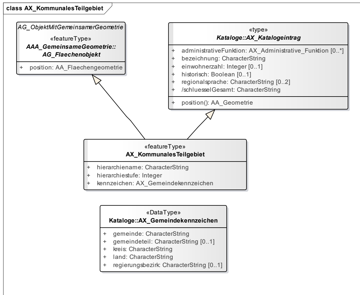
Abbildung 83: Klassendiagramm AX_KommunalesTeilgebiet
