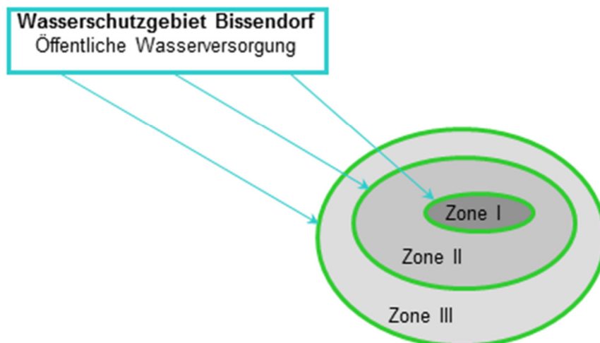
Abbildung 79: Beispiel „AX_SchutzgebietNachWasserrecht“
