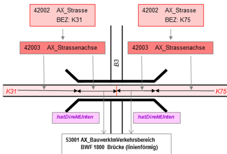
Abbildung 58: Modellierung einer linienförmigen Brücke
