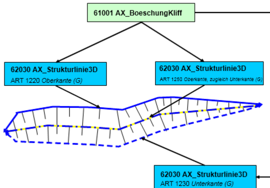
Abbildung 74: Modellierung einer Böschung mit Strukturlinien3D und Gefällewechsel
