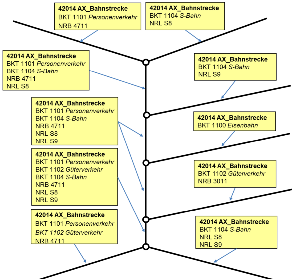
Abbildung 50: Modellierung von Bahnstrecken mit Strecken- und Liniennummern
