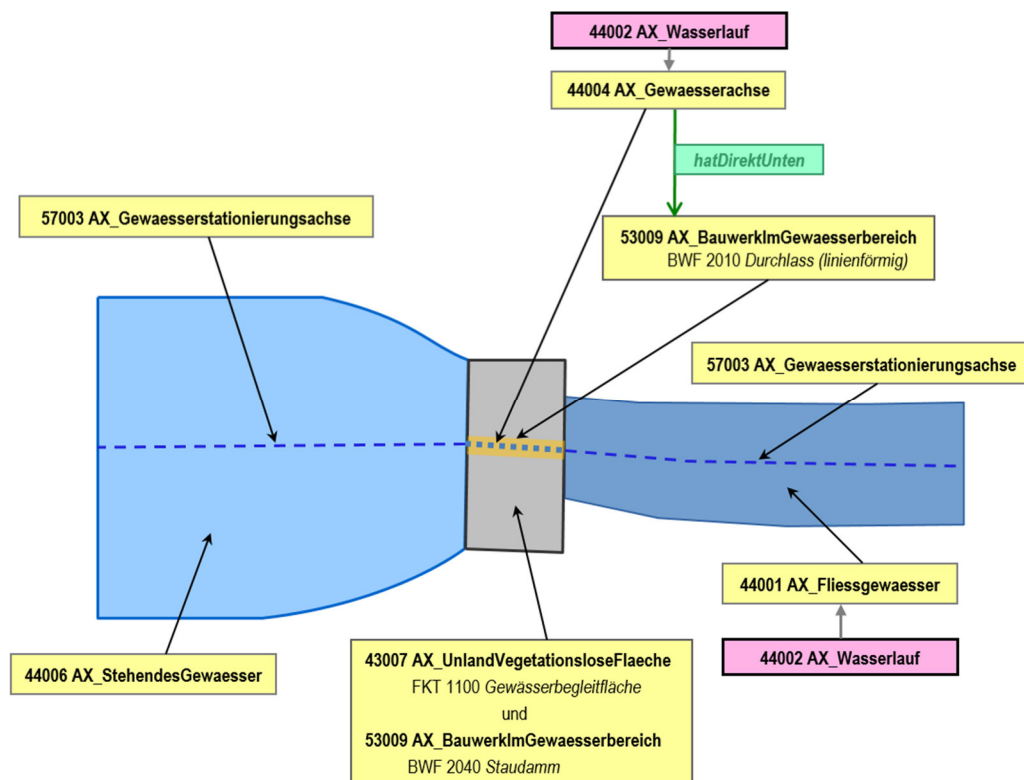
Abbildung 70: Modellierung von Wasserlauf unter Staudamm in linienförmigem Durchlass
