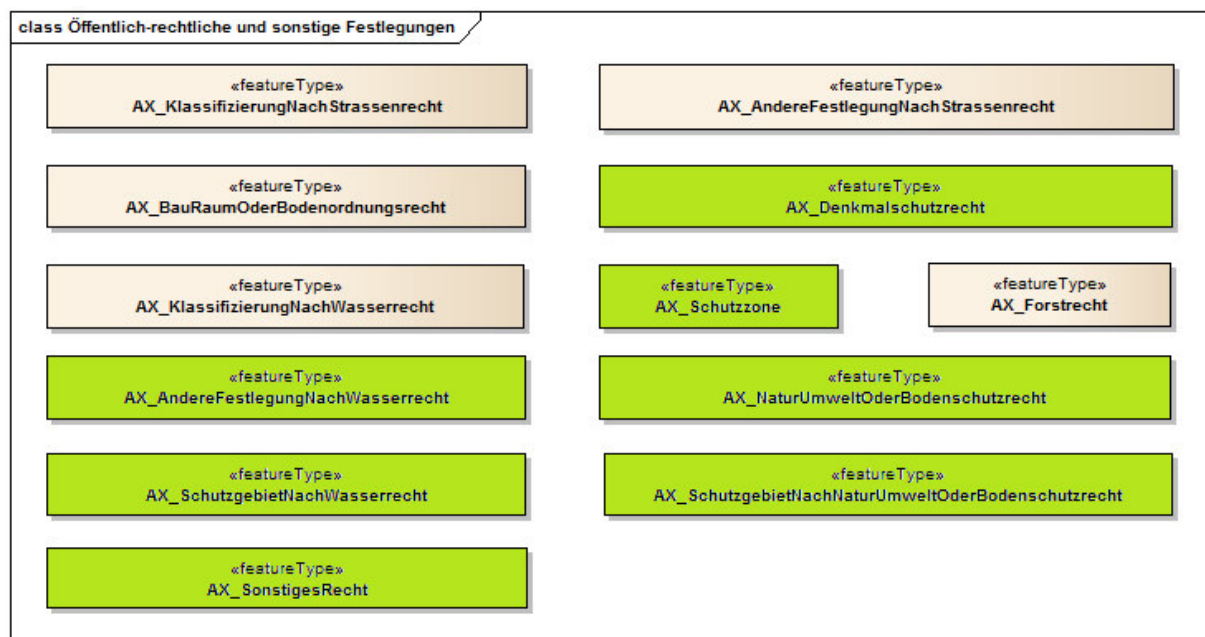
Abbildung 77: Gesetzliche Festlegungen aus UML
