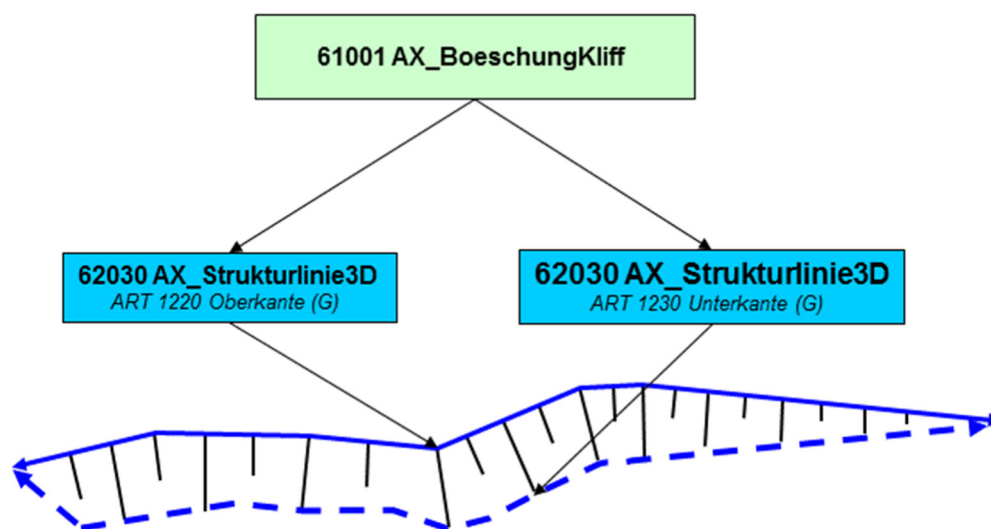
Abbildung 73: Modellierung einer Böschung mit Strukturlinien3D
