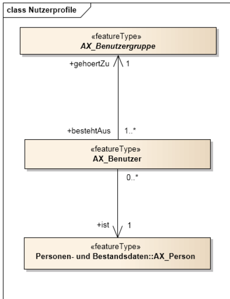
Abbildung 84: Objektartengruppe „Nutzerprofile“ in UML
