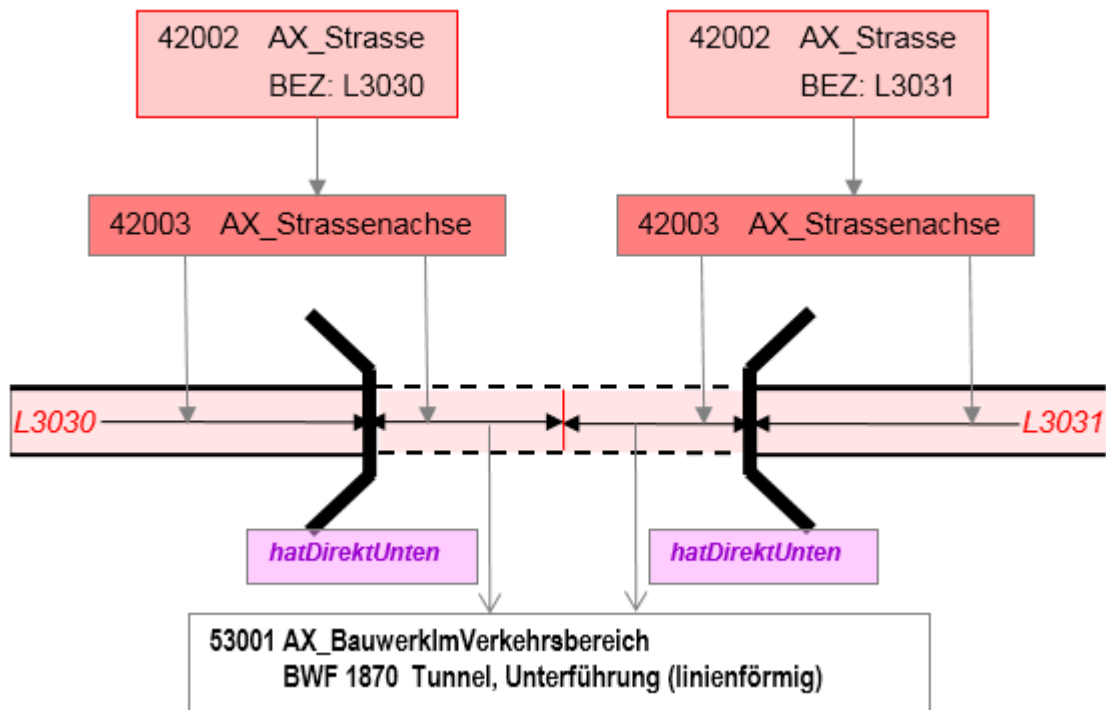
Abbildung 61: Modellierung eines linienförmigen Tunnels
