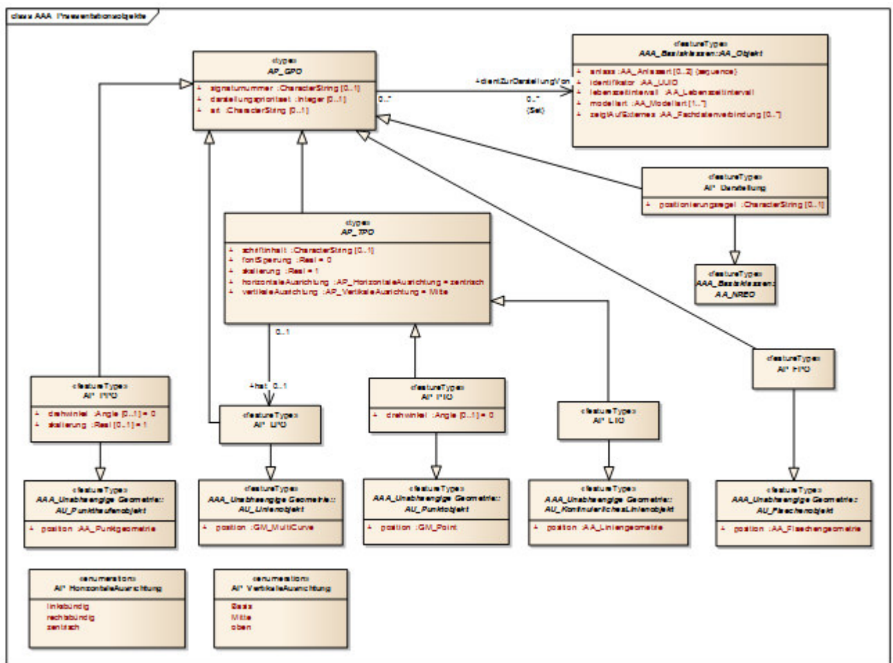
Abbildung 30: AAA-Präsentationsobjekte
