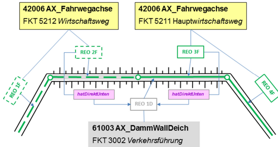
Abbildung 75: Modellierung eines linienförmigen Dammes mit mehreren Fahrwegachsen
