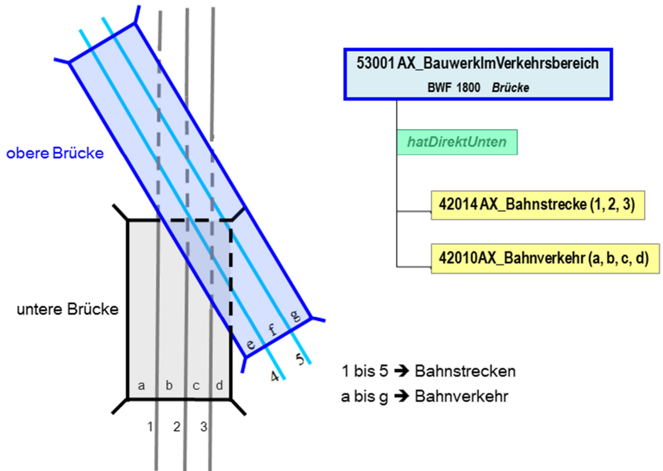
Abbildung 22: Vergabe der Relation „hatDirektUnten“ bei Brücke über Brücke
