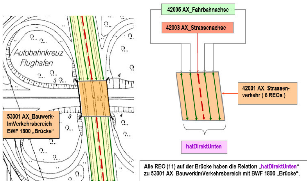
Abbildung 60: Modellierung einer flächenförmigen Brücke mit mehreren Objekten
