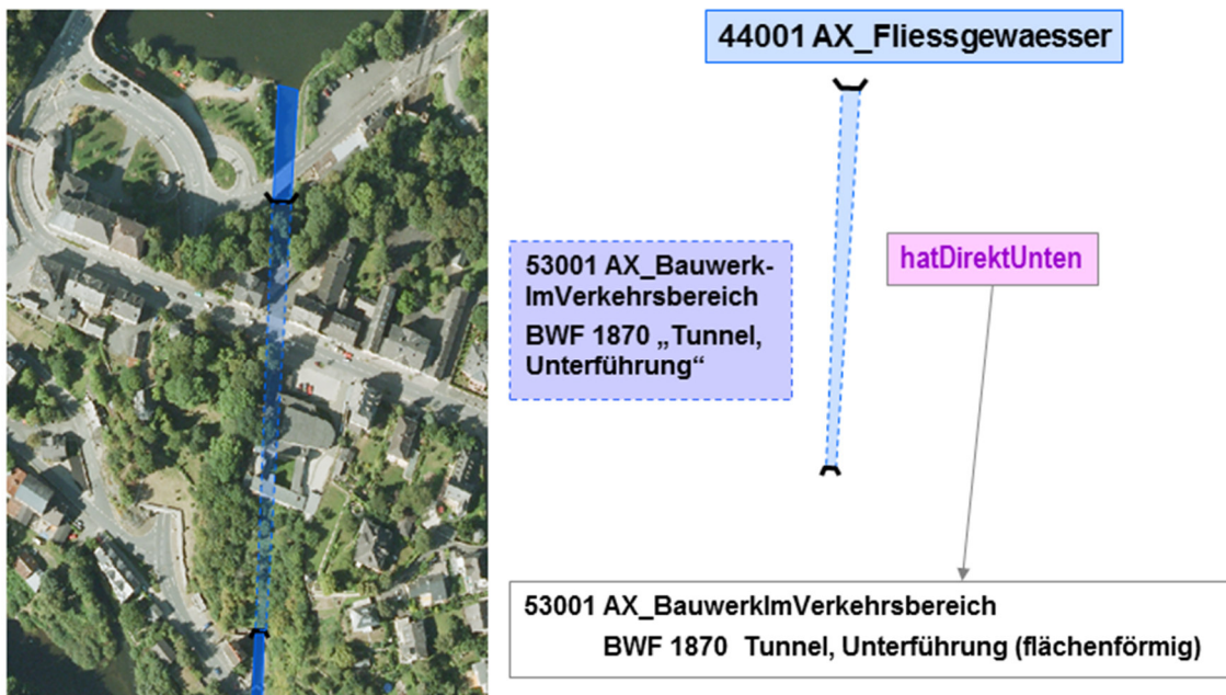
Abbildung 62: Modellierung eines flächenförmigen Tunnels mit einem flächenförmigen Objekt
