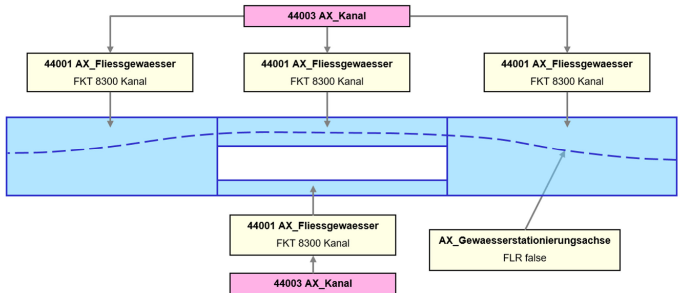
Abbildung 54: Modellierung von Kanälen im Zusammenhang mit Gewässerstationierungsachse und Fließrichtung
