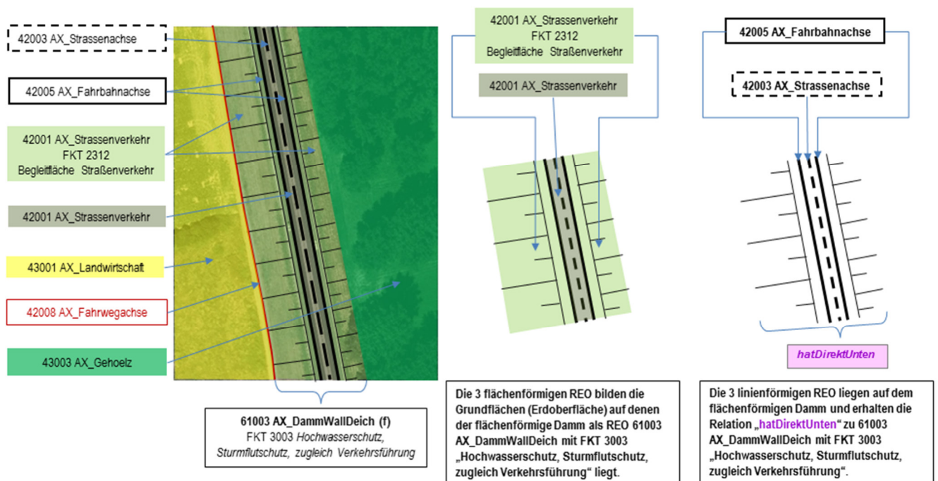
Abbildung 76: Modellierung eines flächenförmigen Dammes mit Straßen- und Fahrbahnachsen
