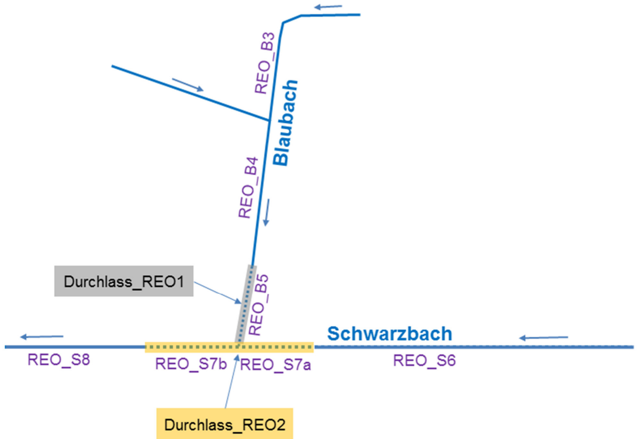
Abbildung 68: Modellierung eines linienförmigen Durchlasses
