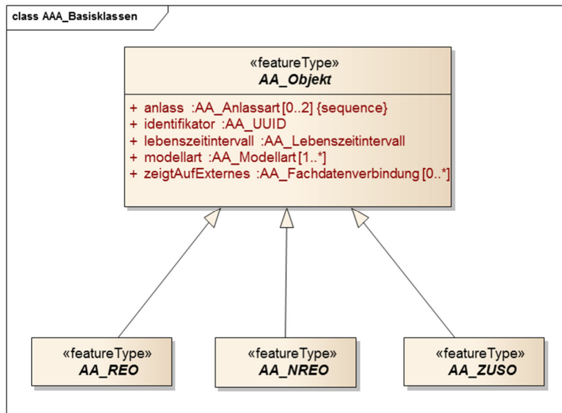
Abbildung 5: Modellierung der Basisklasse AA_Objekt in UML
