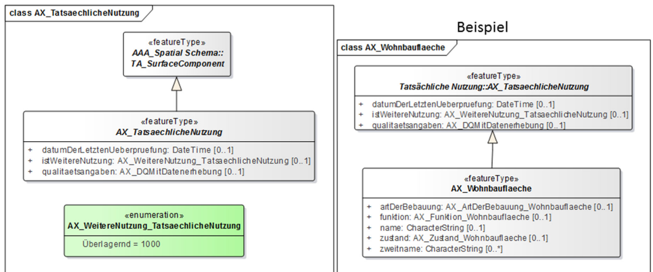
Abbildung 7: Abstrakte Klasse AX_TatsaechlicheNutzung vererbt an AX_Wohnbauflaeche
