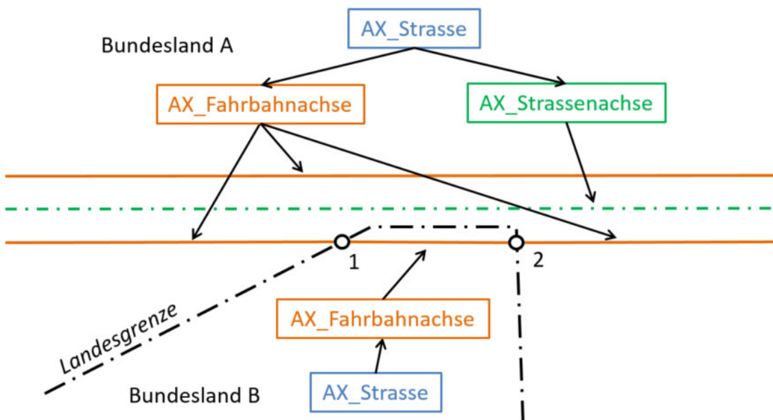
Abbildung 12: Beispiel für die Objektbildung einer komplex modellierten Straße (nur mit AX_Fahrbahnachse) im Bereich einer Landesgrenze
