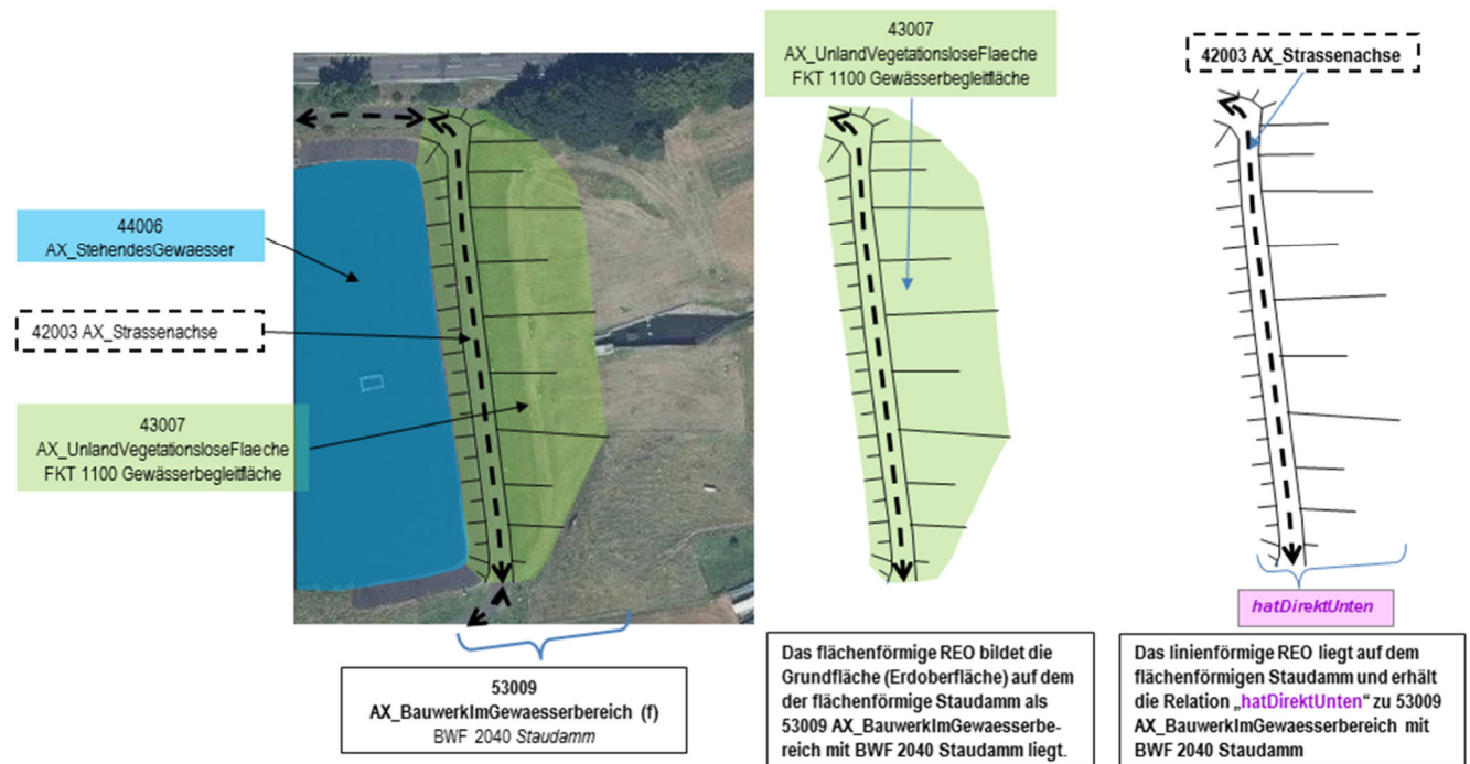
Abbildung 72: Modellierung eines REO Staudamm (flächenförmig) mit einer Straßenachse
