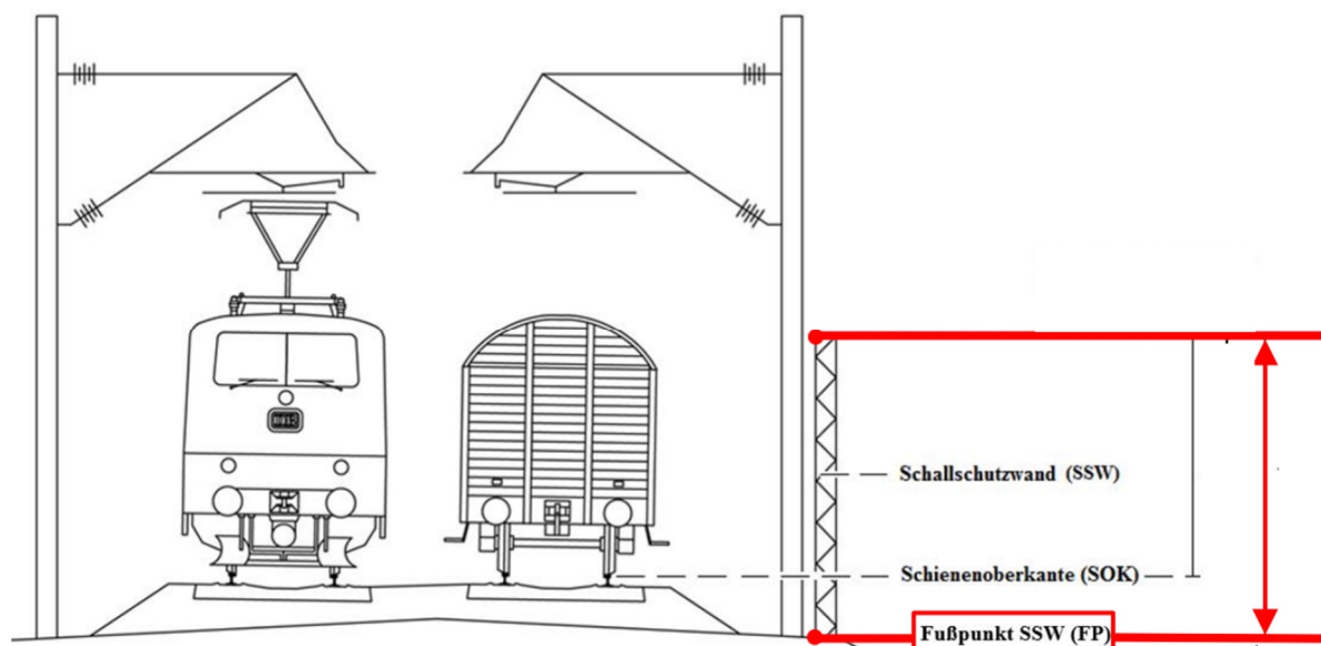
Abbildung 57: Höhenbezugspunkte für die Erhebung von Lärmschutzwänden
