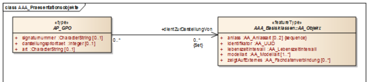
Abbildung 31: Auszug aus Basisschema, AP_GPO
