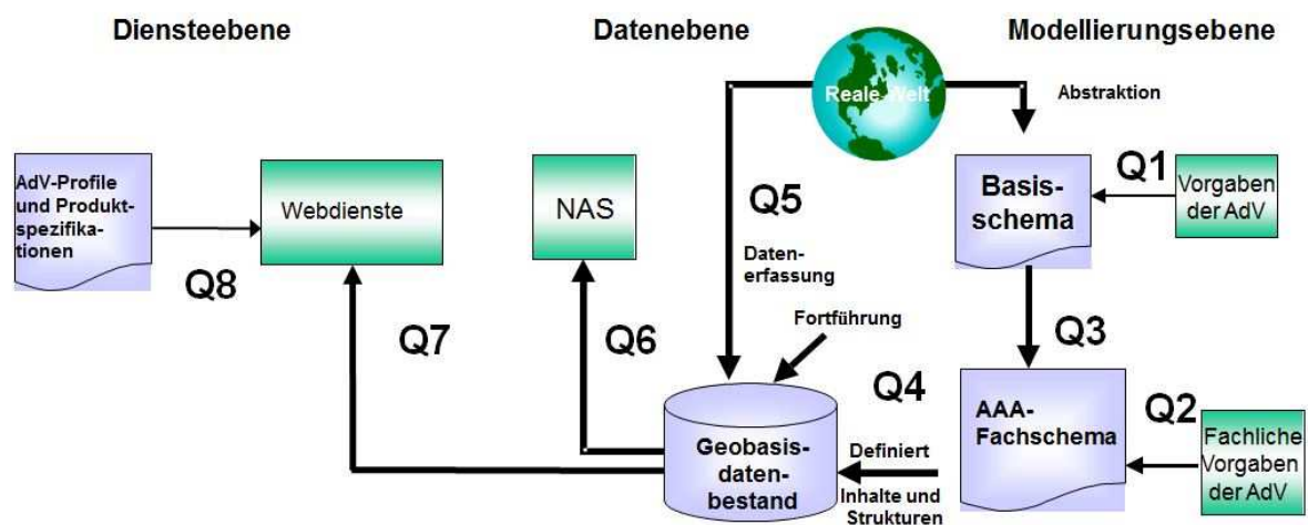
Abbildung 47: Das AdV-Qualitätssicherungsmodell für AAA und Dienste
