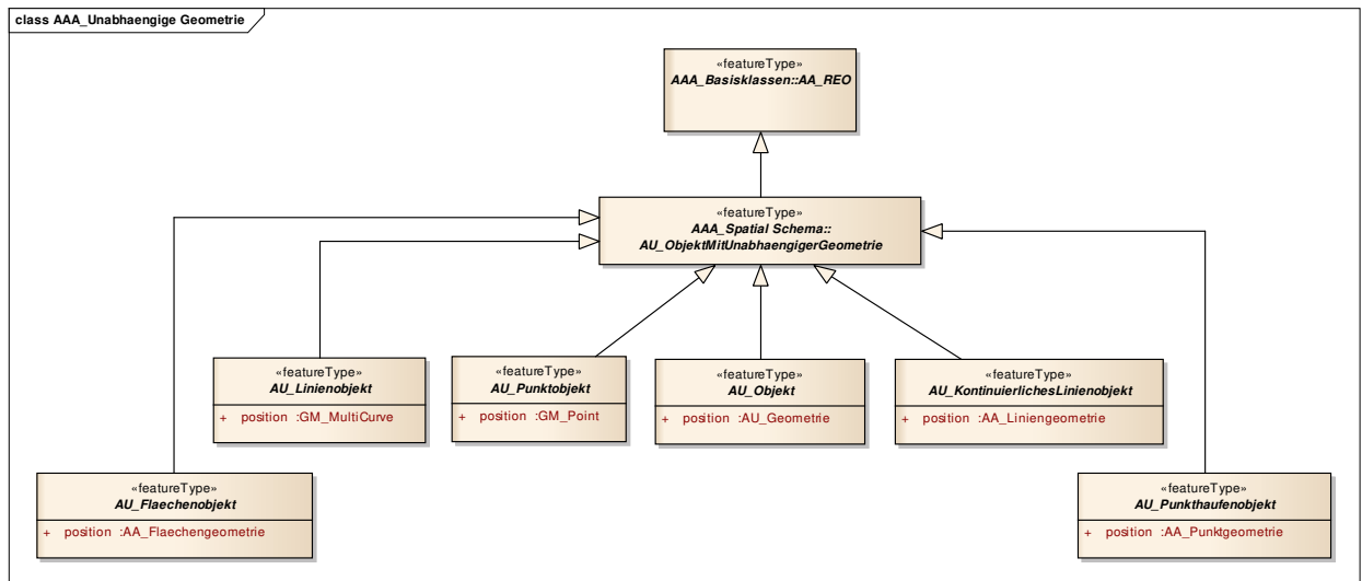
Abbildung 13: 2D-Objekte mit unabhängiger Geometrie
