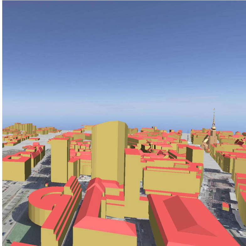
Abbildung 24: LoD 2
