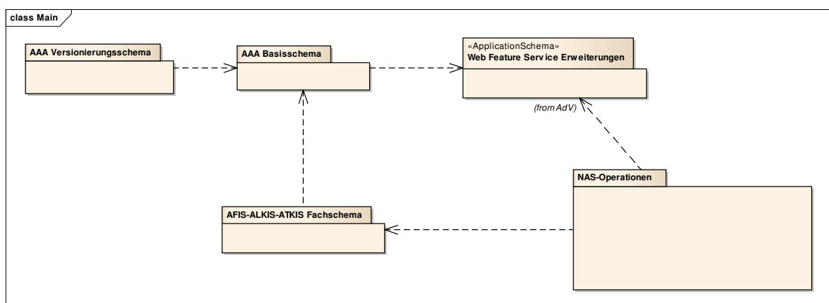
Abbildung 44: Das UML-Paket "NAS-Operationen" im Kontext der Bestandteile des Anwendungsschemas
