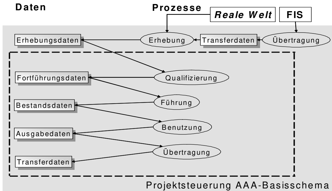
Abbildung 34: Prozesse und Daten der Geoinformationen des amtlichen Vermessungswesens
