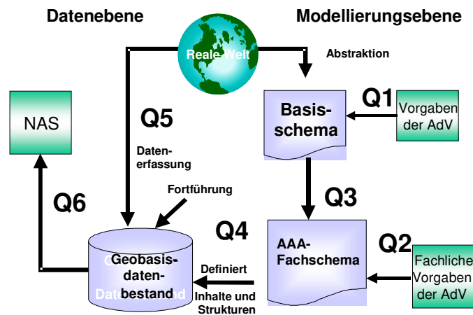
Abbildung 48: Das Qualitätssicherungsmodell des AFIS-ALKIS-ATKIS-Projektes
