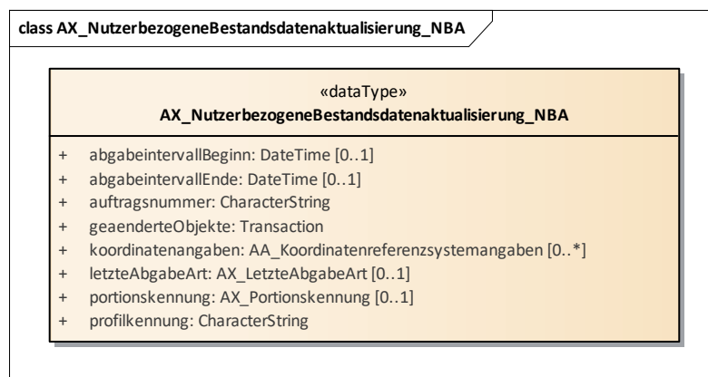
Abbildung 45: Geänderte Objektart AX_Nutzerbezogene-BestandsdatenaktualisierungNBA
