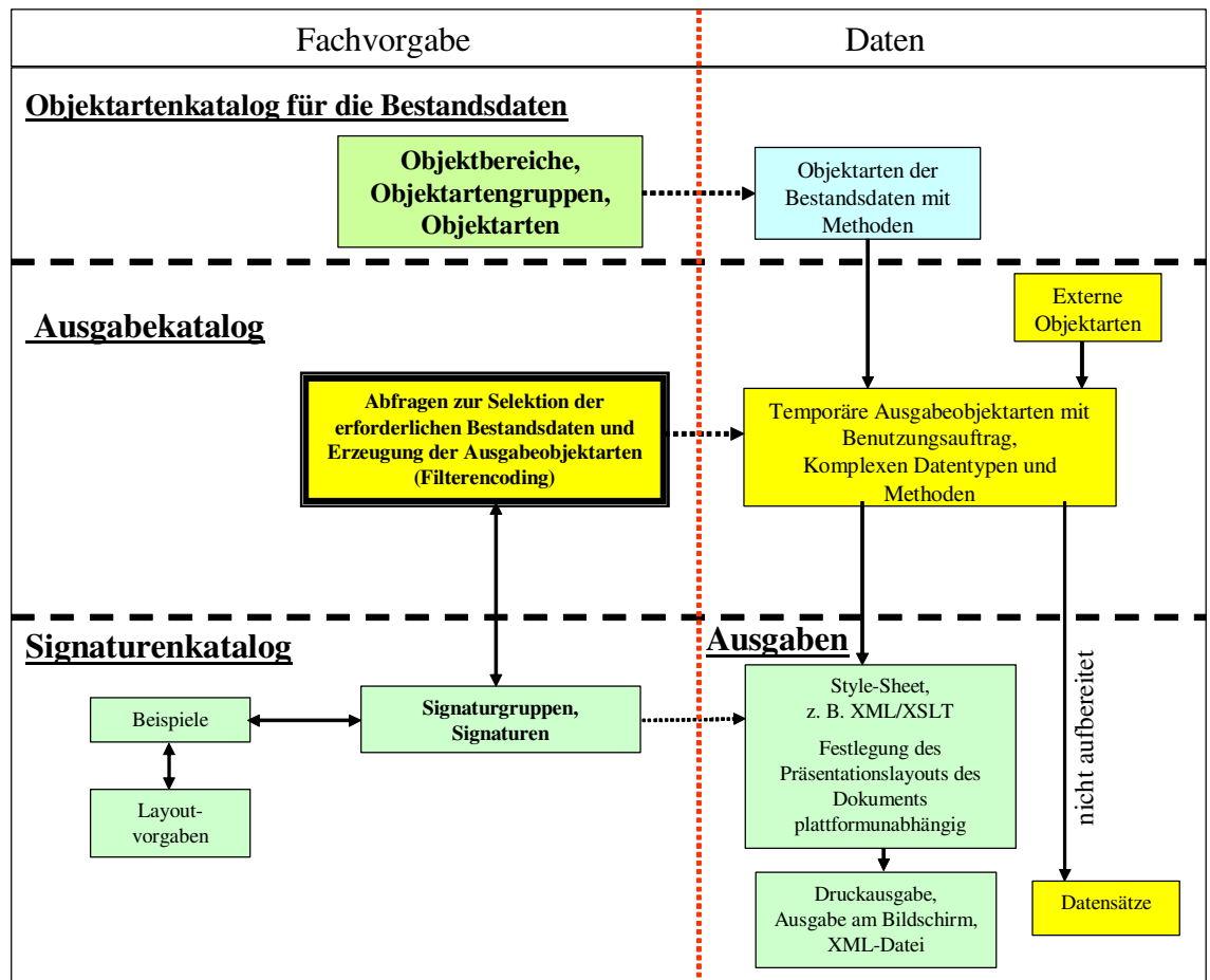
Abbildung 36: Ausgabeschema von ALKIS
