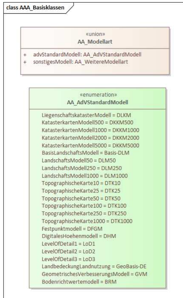
Abbildung 22: Modellarten im Basisschema
