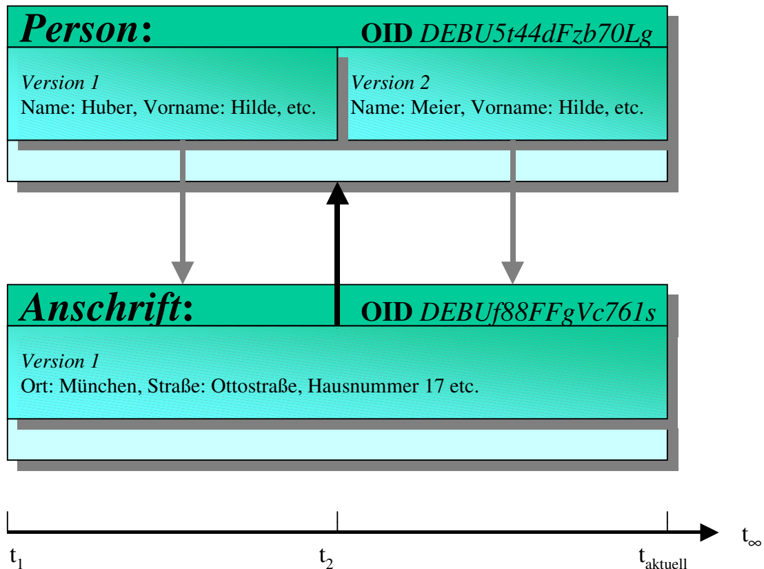
Abbildung 28: Beispiel zur Versionierung nach Änderung von Attributen
