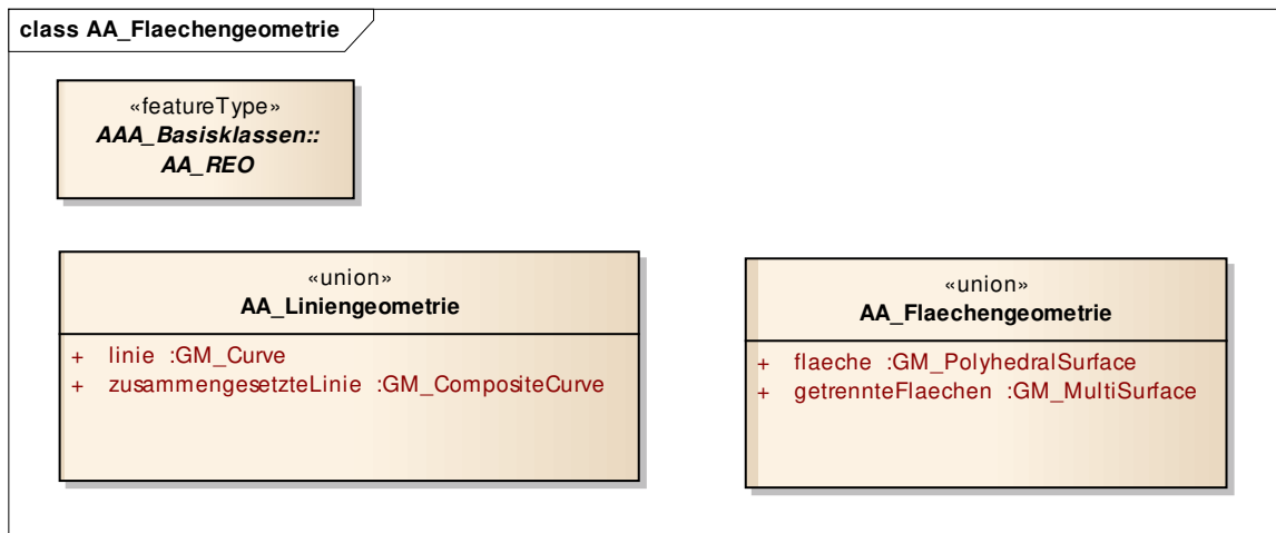
Abbildung 10: Auswahldatentypen zur Bildung unterschiedlicher geometrischer Objektinstanzen
