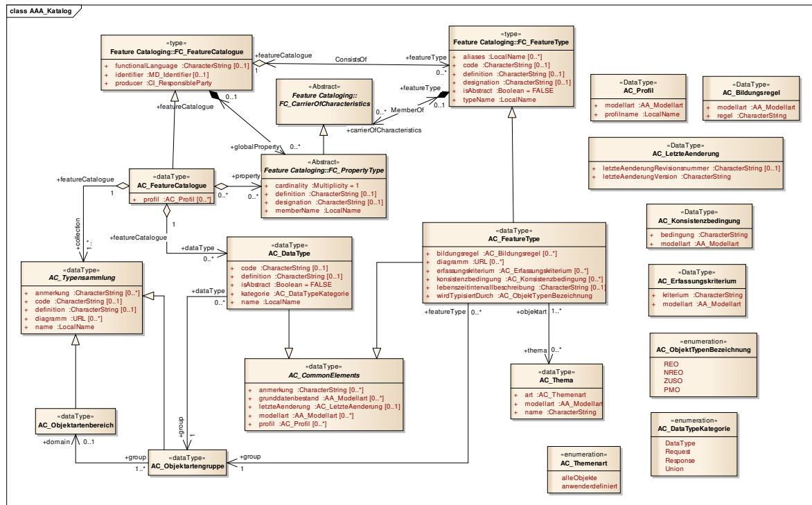
Abbildung 32: Erweiterungen der genormten Struktur der Objektartenkataloge
