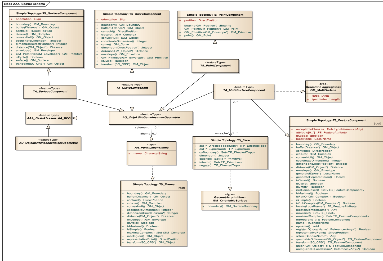
Abbildung 9: Zusammenfassende Darstellung der für AFIS-ALKIS-ATKIS erforderlichen Ergnzungen am genormten Spatial Schema
