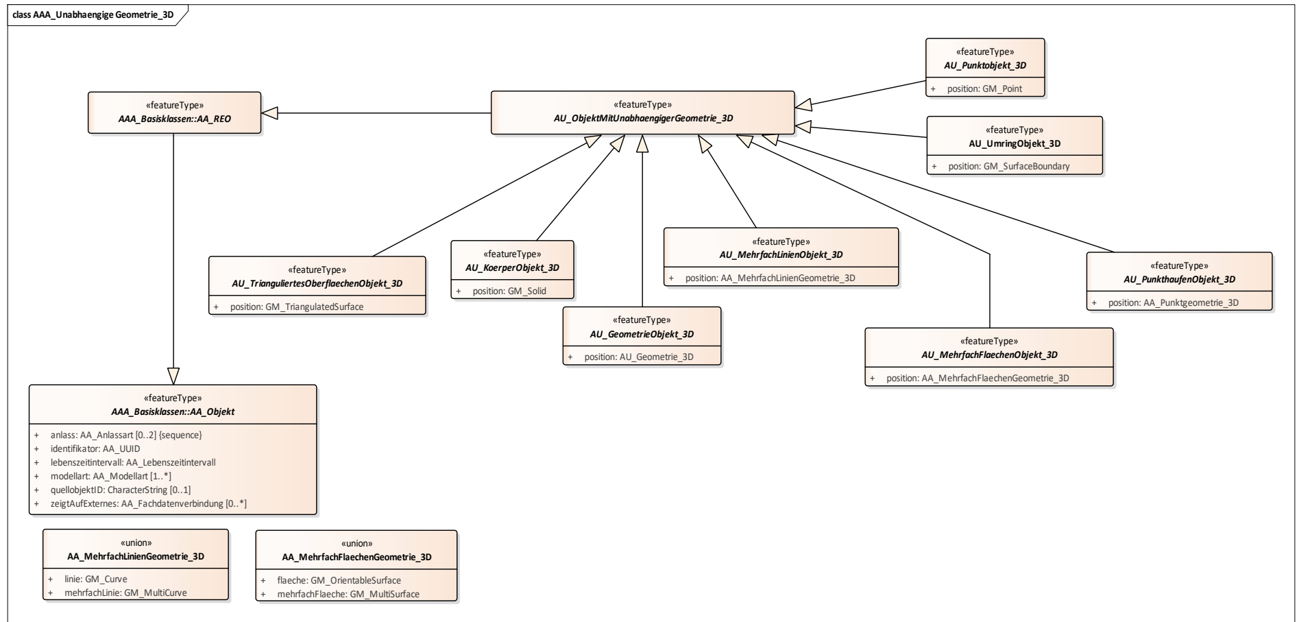
Abbildung 15: 3D-Objekte mit unabhängiger Geometrie
