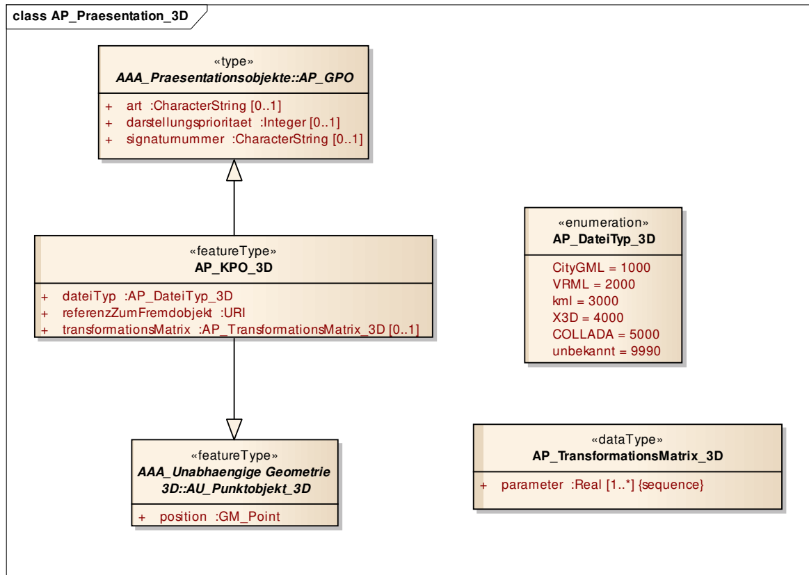
Abbildung 20: Präsentationsobjekte_3D
