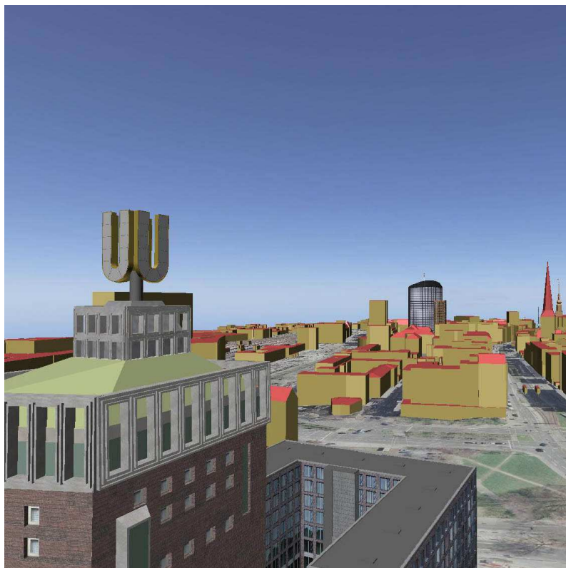
Abbildung 25: LoD 3
