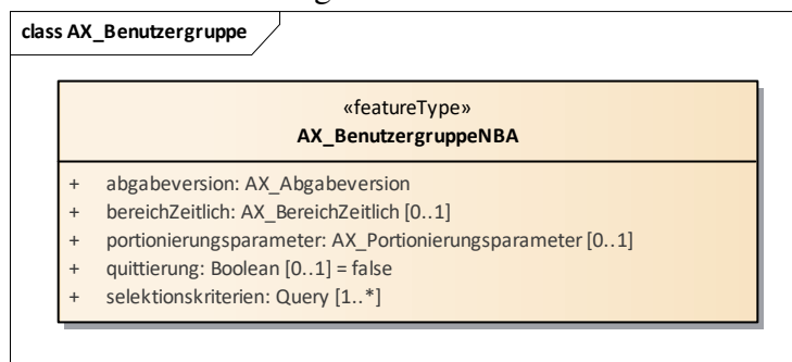
Abbildung 31: Neue Attributart ‚abgabeverision‘ zur Selektion von Objekten verschiedener GeoInfoDok-Versionen
