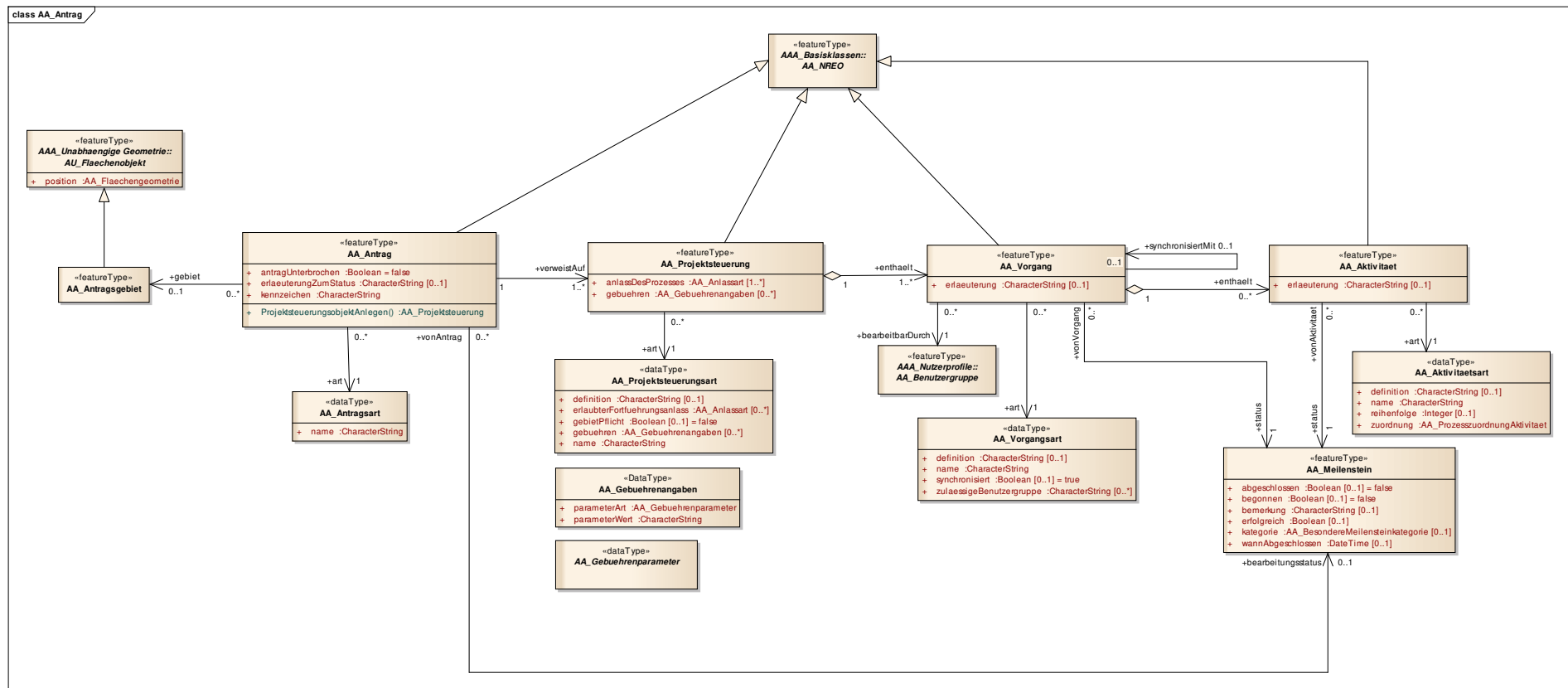
Abbildung 37: Klassendiagramm "AA_Antrag"
