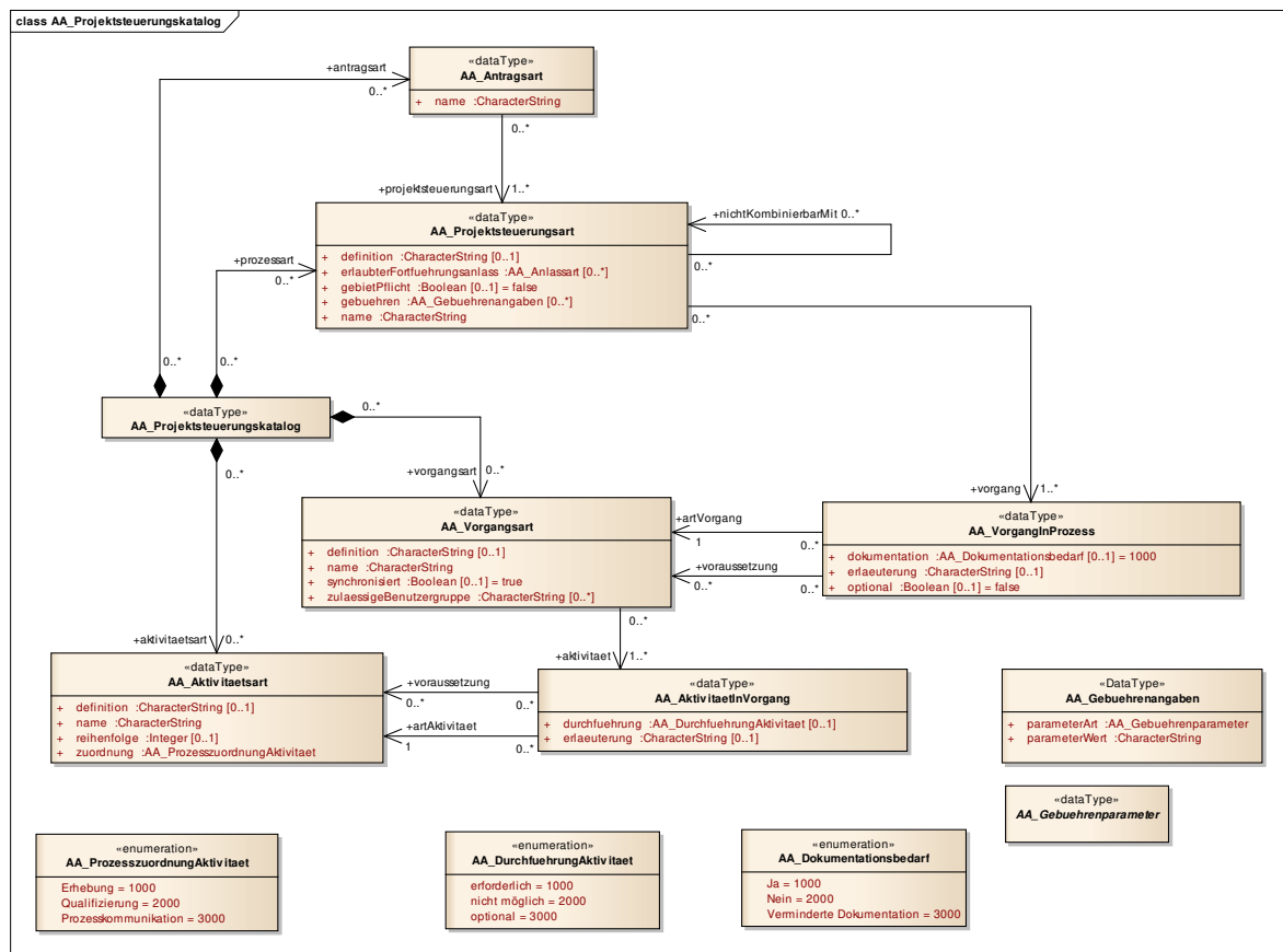
Abbildung 38: Klassendiagramm "AA_Projektsteuerungskatalog"
