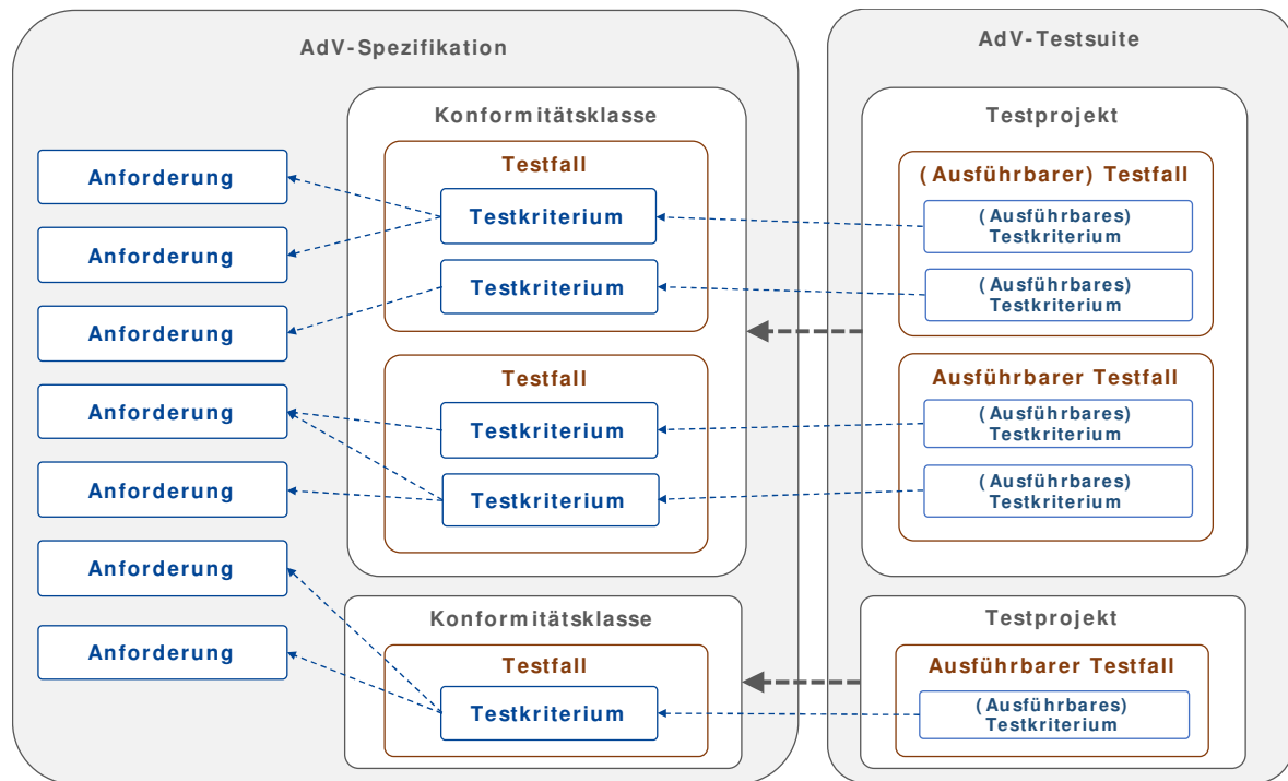
Abbildung 49: Hierarchie von Konformitätsklasse, Testfall und Testkriterium
