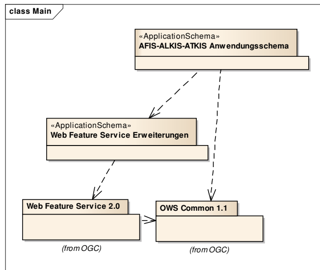
Abbildung 3: Abhängigkeit des AFIS-ALKIS-ATKIS-Anwendungsschemas von den genormten Strukturen aus OGC
