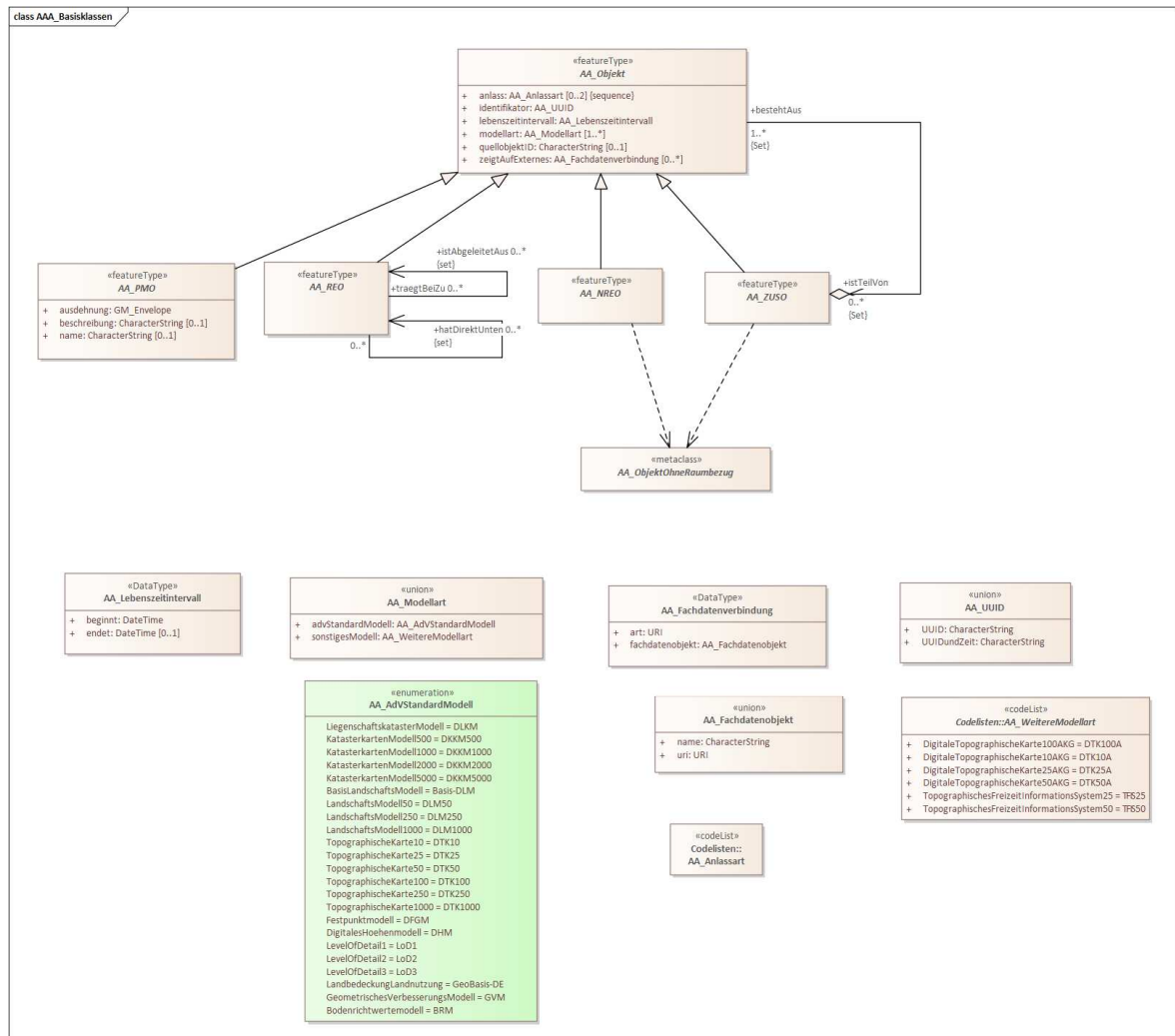
Abbildung 8: Modellierung der AAA-Basisklassen
