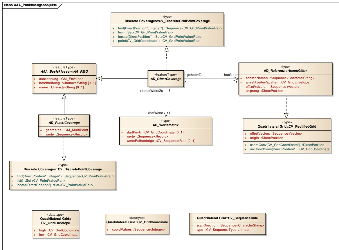
Abbildung 21: Modellierung der Punktmengenobjekte
