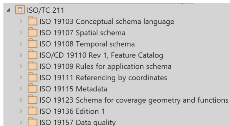
Abbildung 4: Verwendete Teile aus der Normfamilie ISO 19100 (Auszug aus dem UML-Datenmodell)
