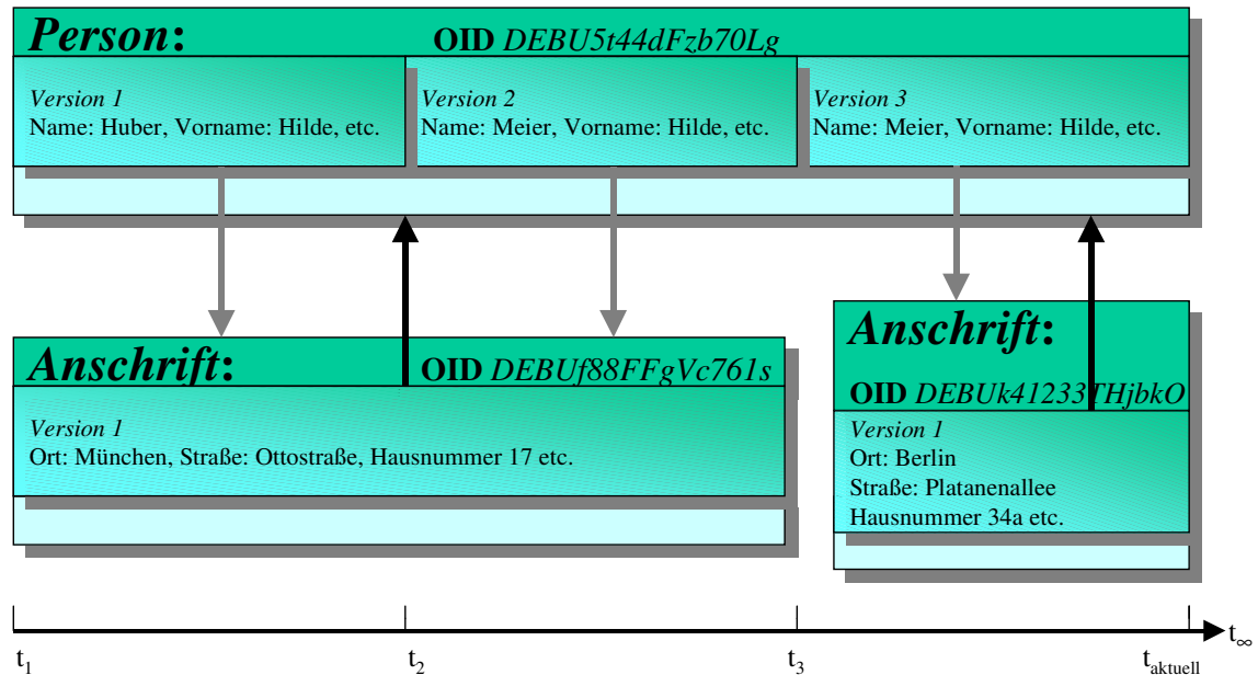
Abbildung 29: Beispiel zur Versionierung nach Änderung von Relationen
