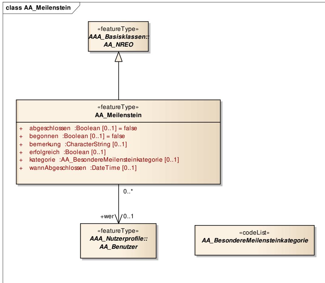
Abbildung 39: Klassendiagramm "AA_Meilenstein"
