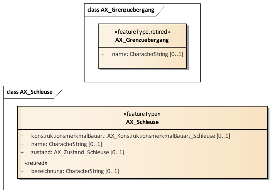
Abbildung 30: Beispiel für eine zurückgezogene Objektart (AX_Grenzübergang) und eine zurückgezogene Attributart („bezeichnung“ in AX_Schleuse)
