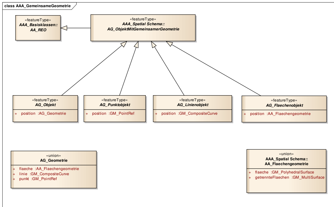
Abbildung 11: Objekte mit gemeinsamer Geometrie
