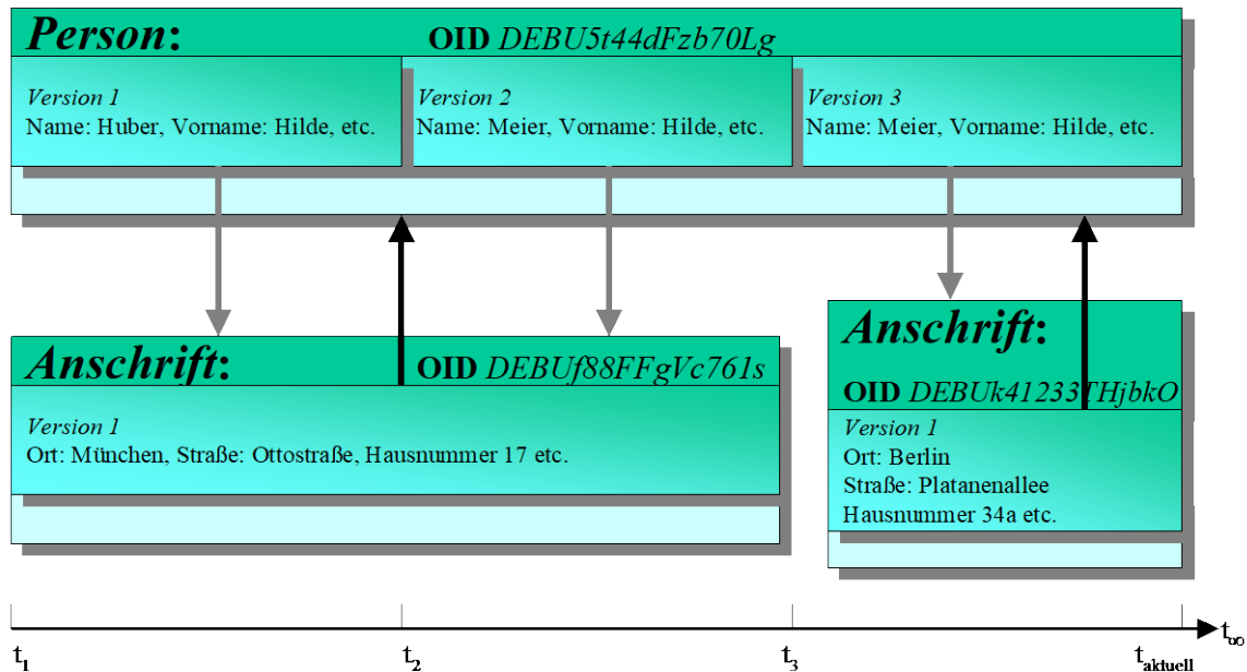
Abbildung 29: Beispiel zur Versionierung nach Änderung von Relationen
