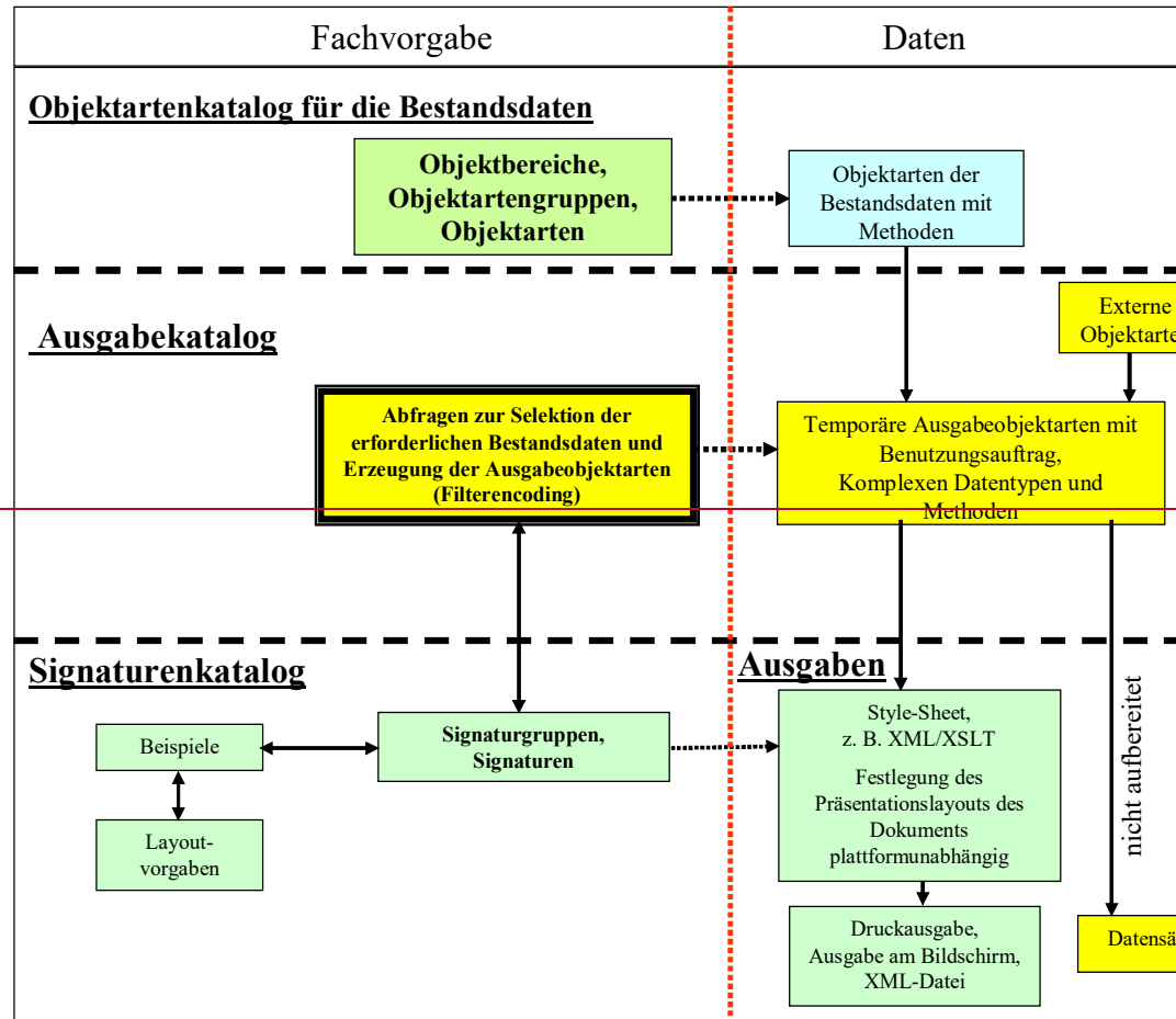
Abbildung 36: Ausgabeschema von ALKIS
