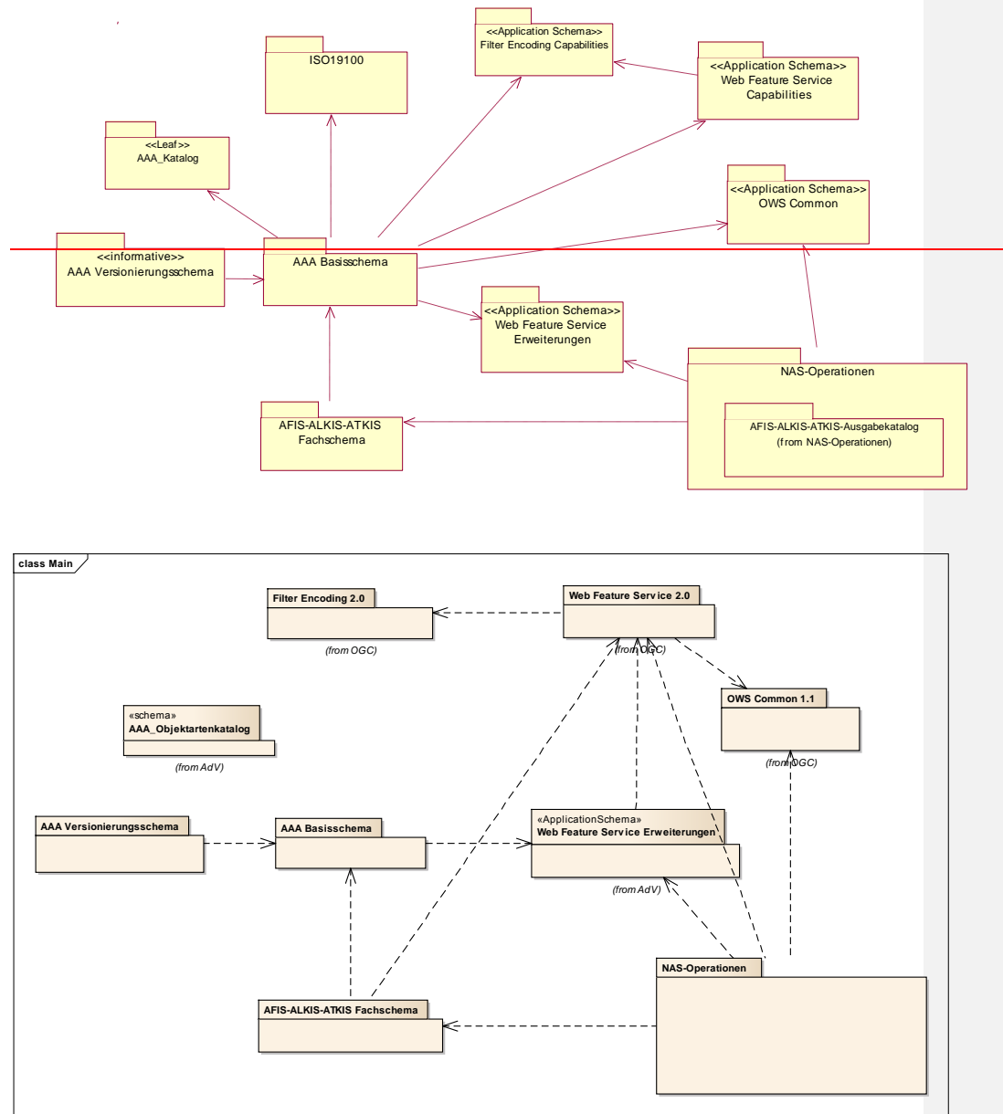
Abbildung 5: Die Bestandteile des AFIS-ALKIS-ATKIS-Anwendungsschemas
