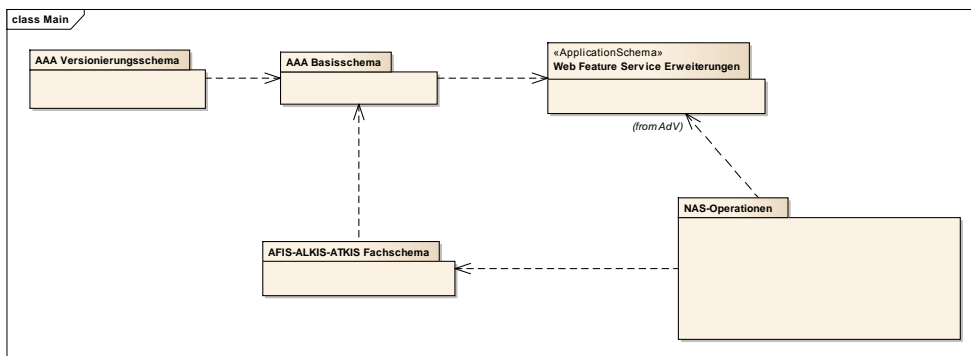
Abbildung 48: Das UML-Paket "NAS-Operationen" im Kontext der Bestandteile des Anwendungsschemas
