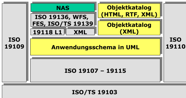
Abbildung 45: Einbettung der NAS in Normen und Standards
