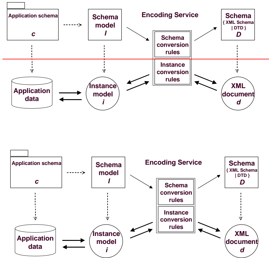
Abbildung 46: XML-basierende Kodierungsregeln gemäß ISO 19118
