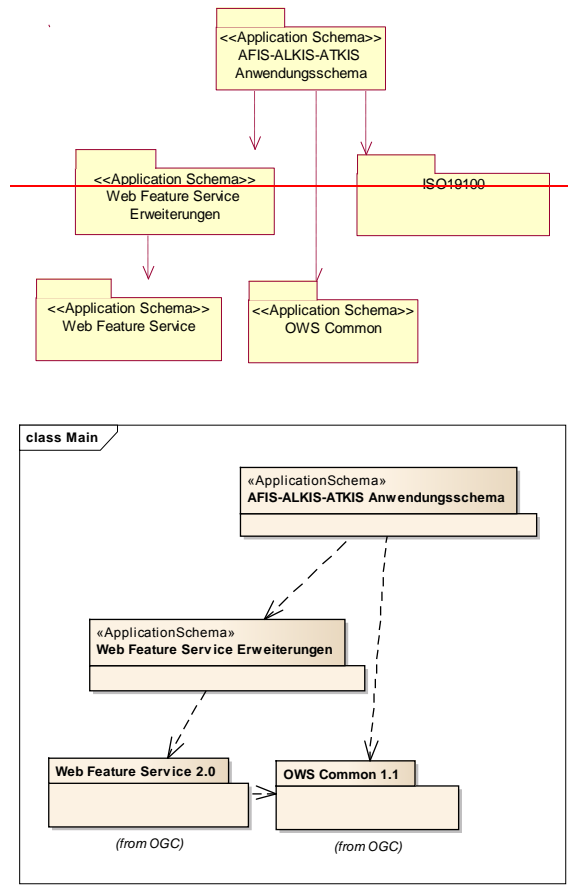
Abbildung 3: Abhängigkeit des AFIS-ALKIS-ATKIS-Anwendungsschemas von den genormten Strukturen aus ISO 19100 und OGC
