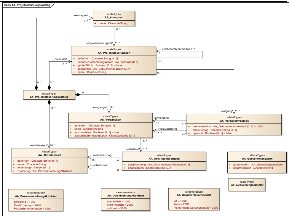
Abbildung 42: Klassendiagramm "AA_Projektsteuerungskatalog"
