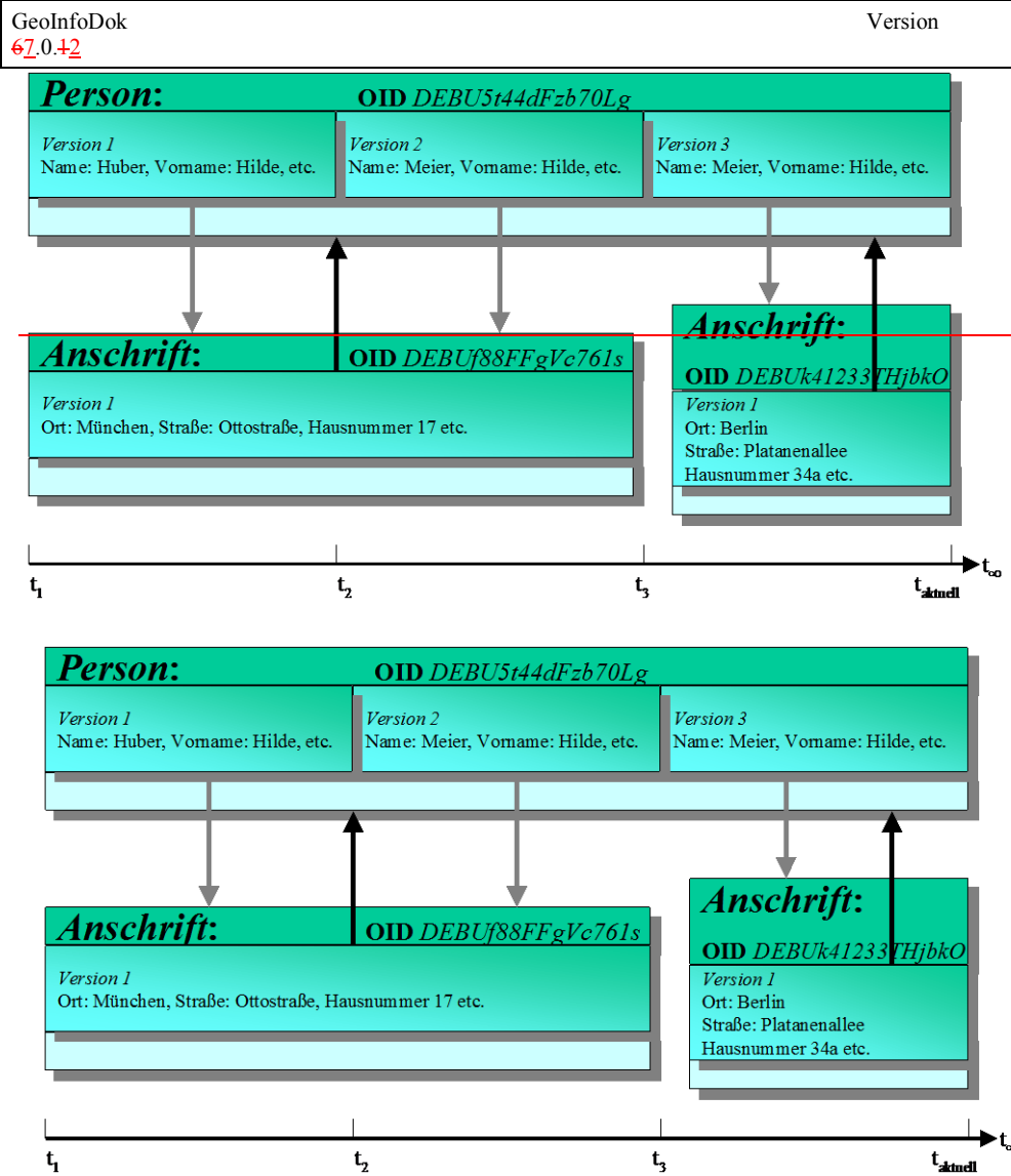
Abbildung 35: Beispiel zur Versionierung nach Änderung von Relationen
