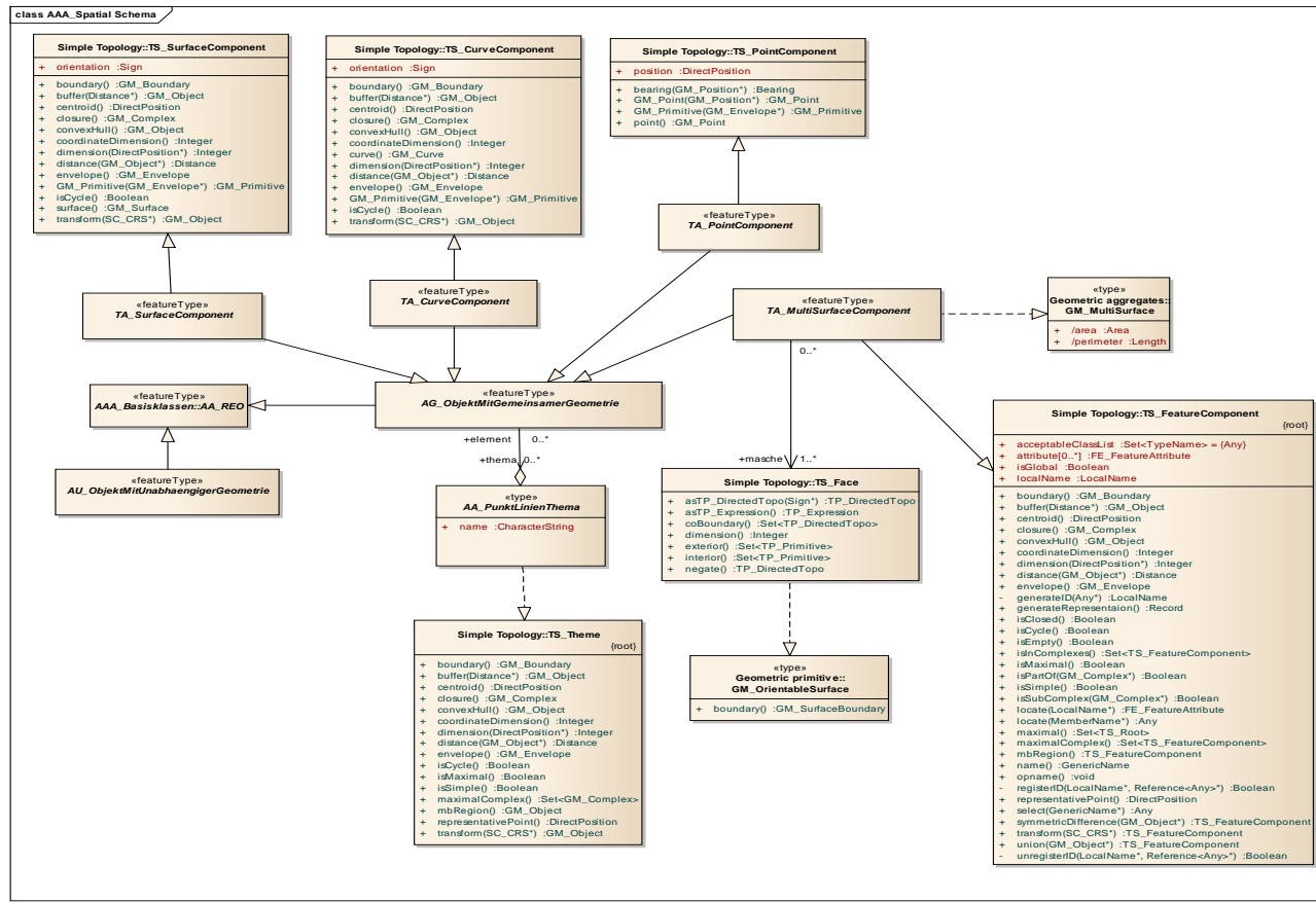
Abbildung 12: Zusammenfassende Darstellung der für AFIS-ALKIS-ATKIS erforderlichen Erganzen am genormten Spatial Schema
