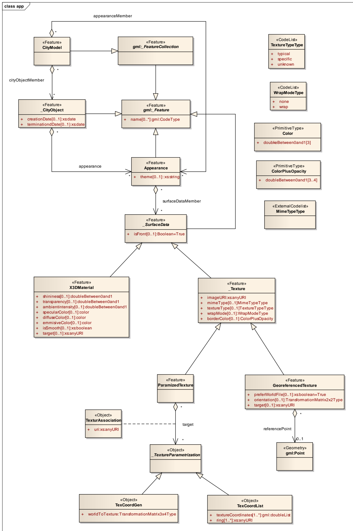
Abbildung 8: CityGML-Profil für LoD 2 der AdV (Appearance)
