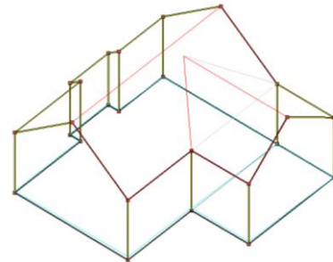
Abbildung 10: Verwendung der Objektart WallSurface
