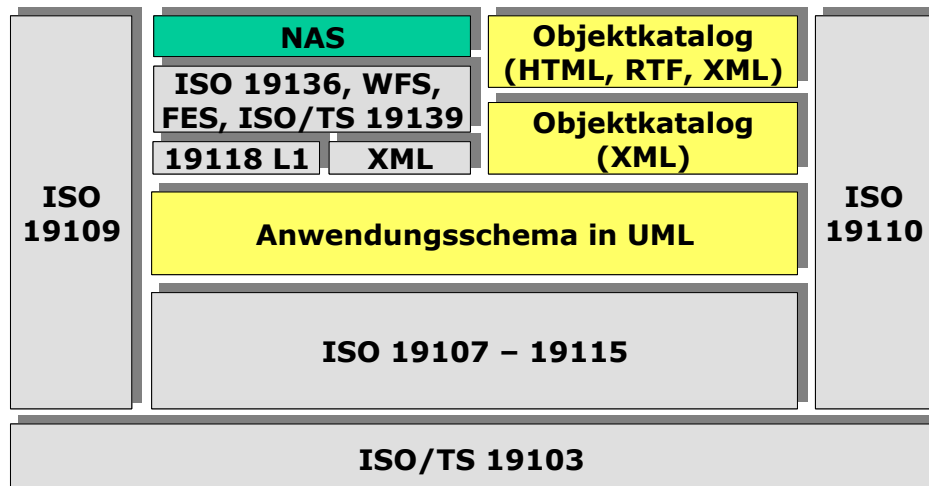
Abbildung 40: Einbettung der NAS in Normen und Standards
