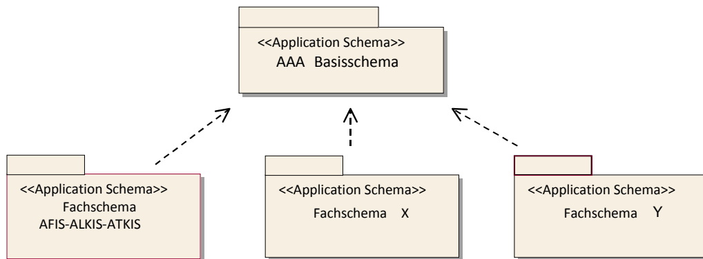
Abbildung 6: Das Basisschema als Grundlage für anwendungsspezifische Fachschemata (z.B. AFIS, ALKIS und ATKIS)
