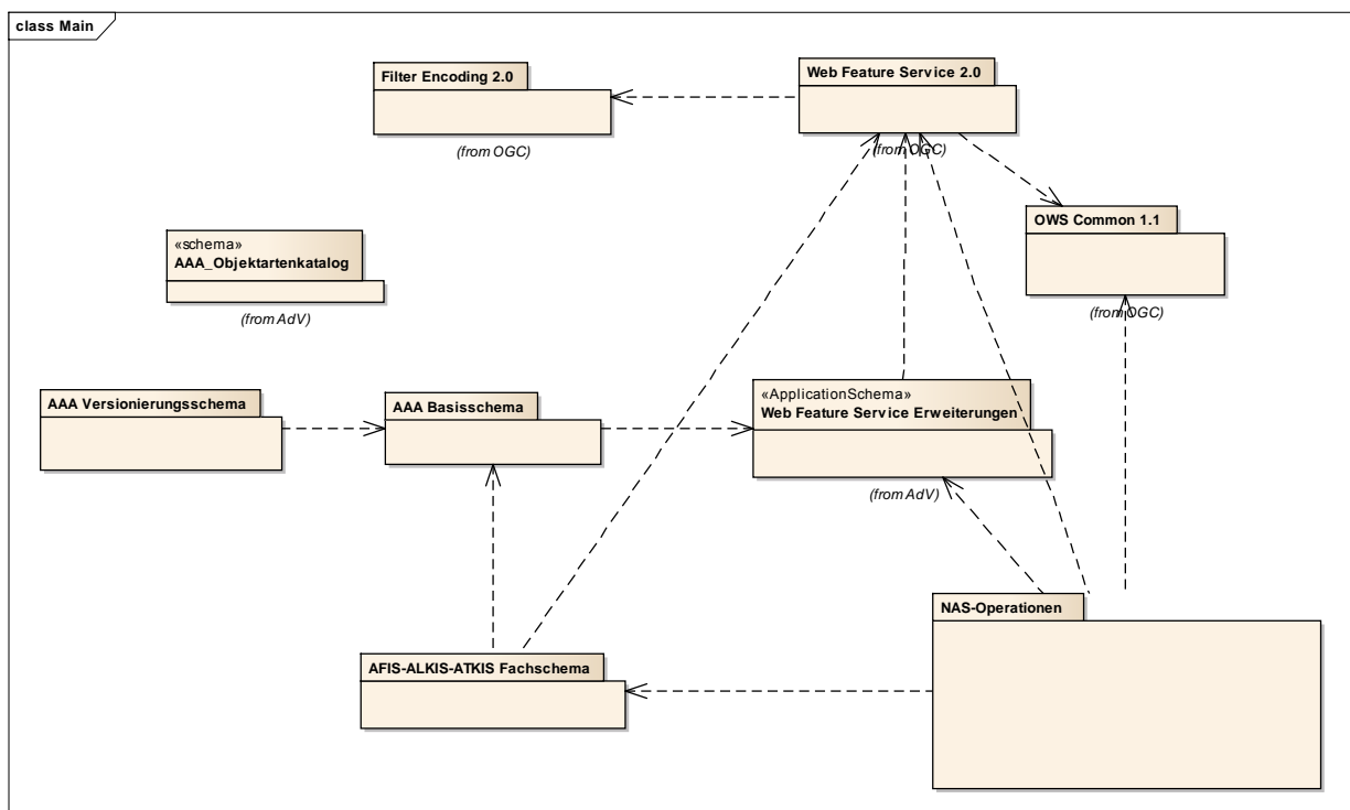
Abbildung 5: Die Bestandteile des AFIS-ALKIS-ATKIS-Anwendungsschemas
