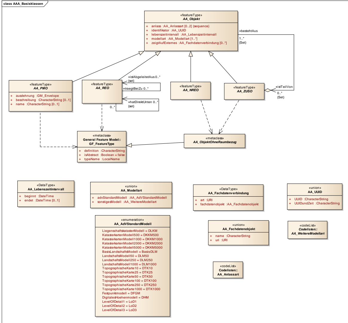
Abbildung 8: Modellierung der AAA-Basisklassen
