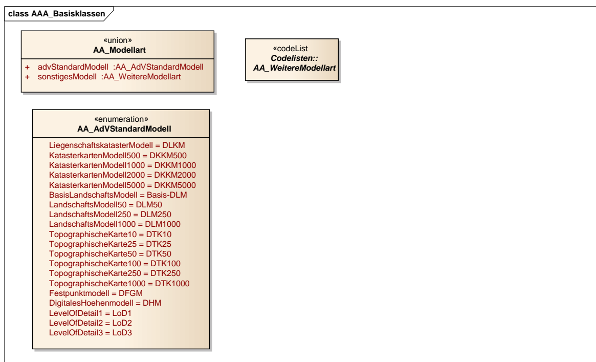
Abbildung 23: Modellarten im Basisschema
