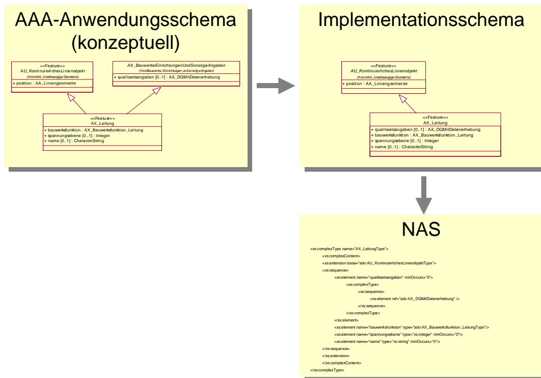
Abbildung 39: Zweistufiger Ableitungsprozess der NAS
