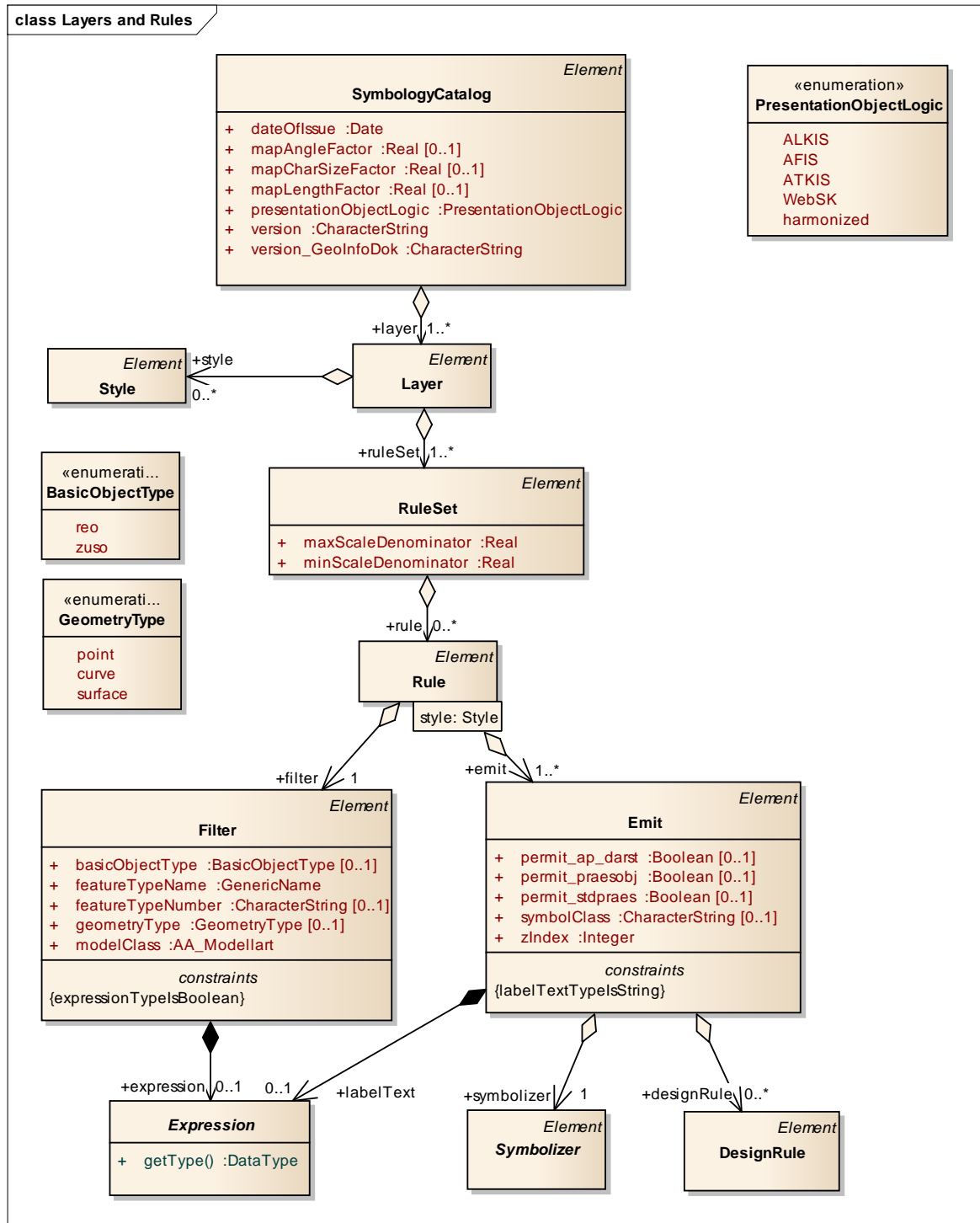
Abbildung 32: Schema SK-Objektmodell
