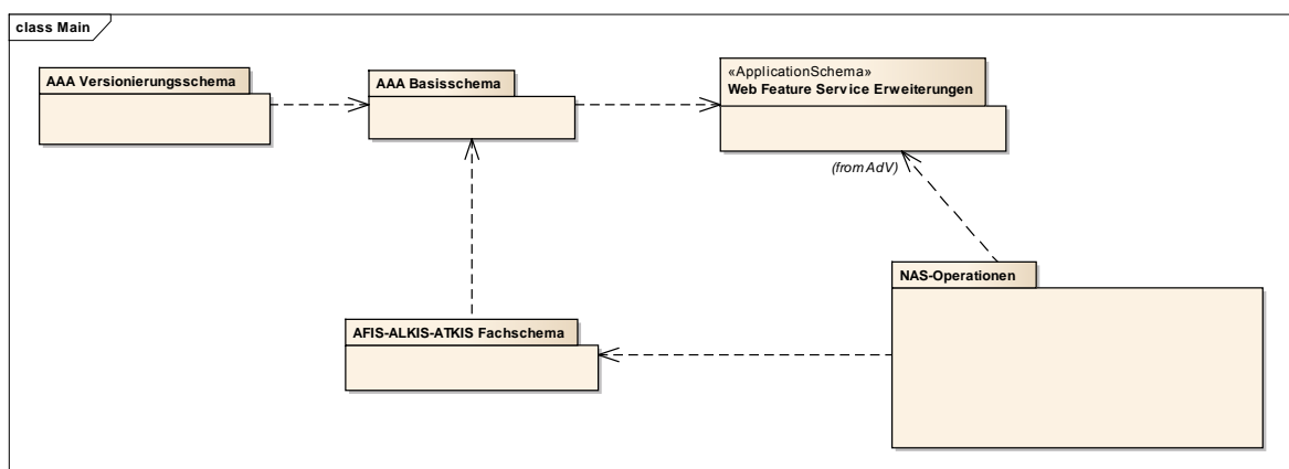
Abbildung 43: Das UML-Paket "NAS-Operationen" im Kontext der Bestandteile des Anwendungsschemas
