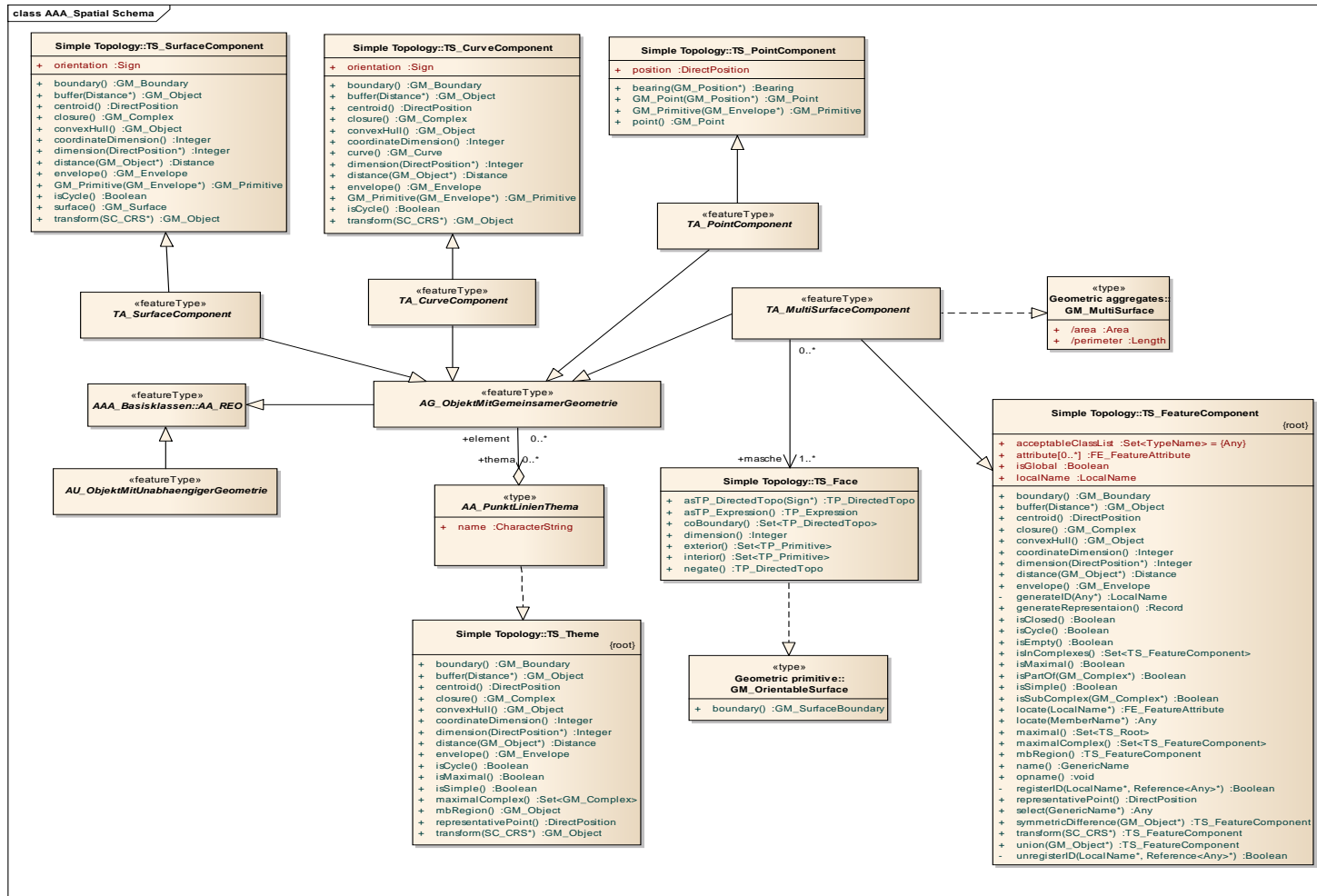
Abbildung 9: Zusammenfassende Darstellung der für AFIS-ALKIS-ATKIS erforderlichen Ergänzungen am genormten Spatial Schema
