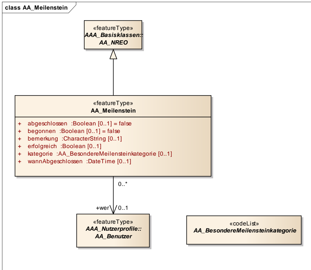
Abbildung 38: Klassendiagramm "AA_Meilenstein"
