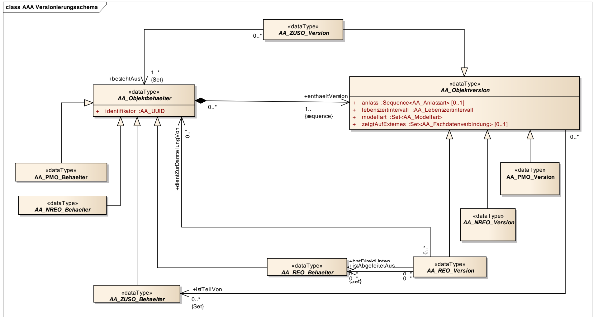
Abbildung 28: Versionierungsschema
