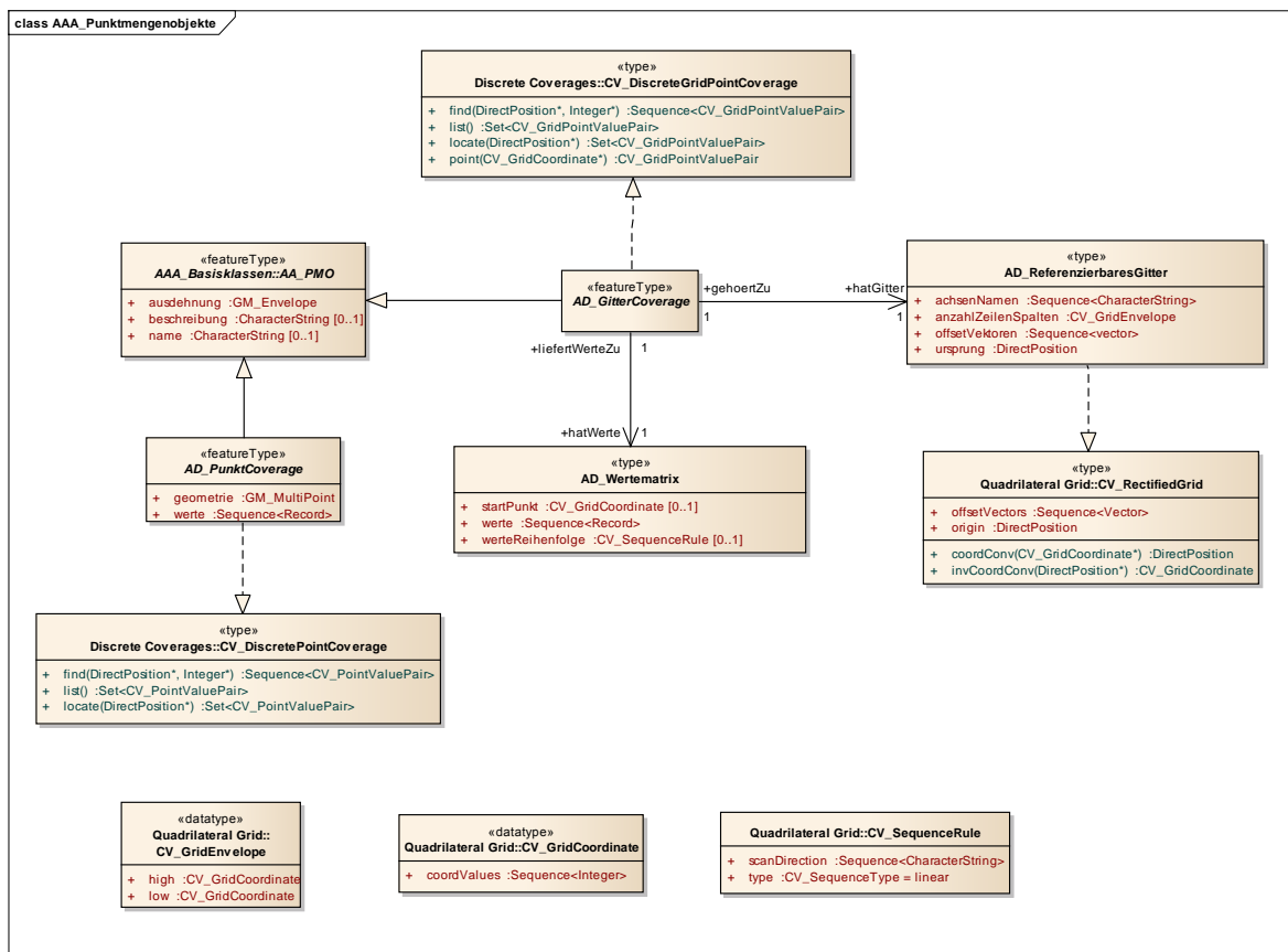
Abbildung 22: Modellierung der Punktmengenobjekte
