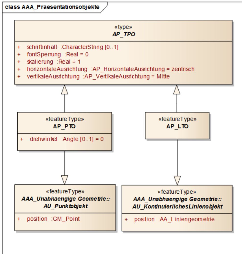
Abbildung 27: Auszug aus Basisschema, AP_TPO
