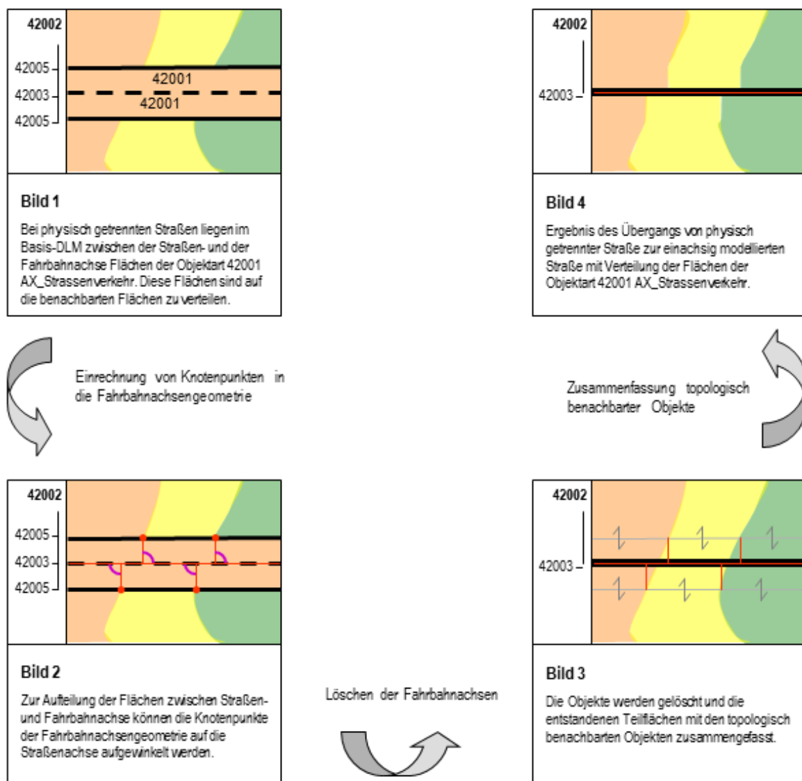
Abbildung 21: Flächenaufteilung beim Übergang von physisch getrennten zu einfach modellierten Straßen
