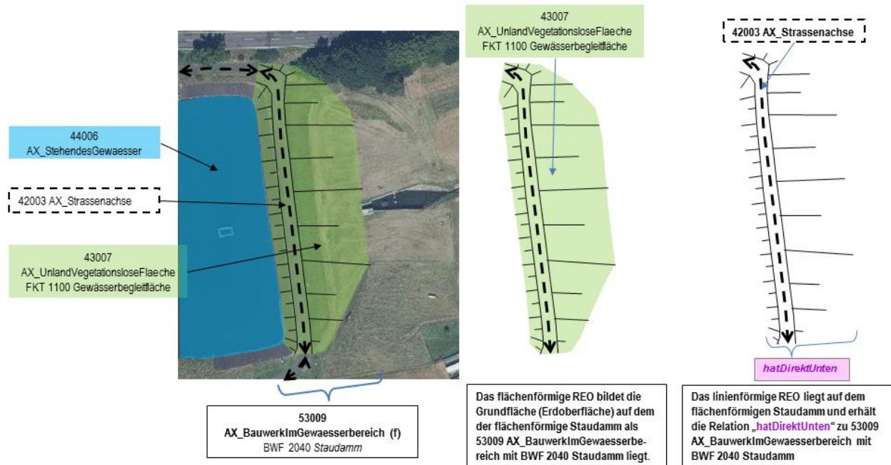
Abbildung 55: Modellierung eines REO Staudamm (flächenförmig) mit einer Straßenachse
