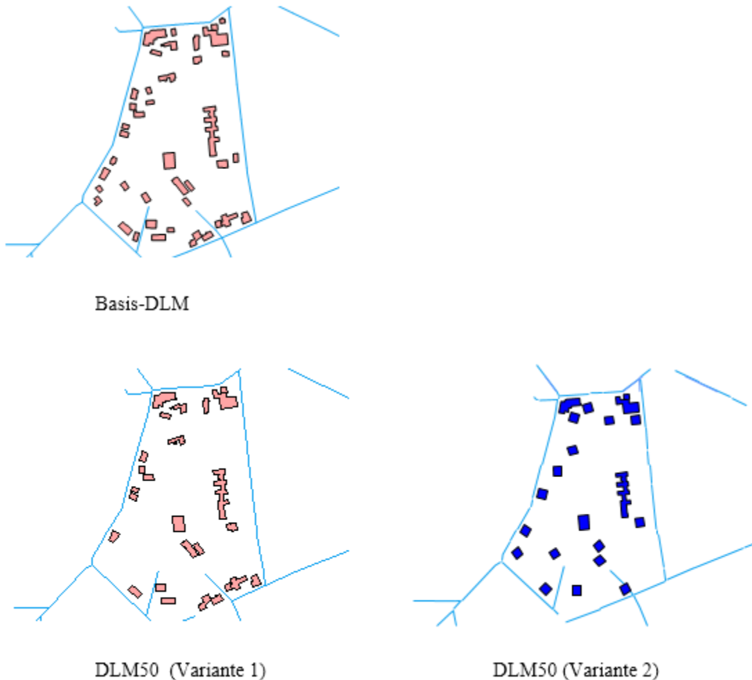
Abbildung 28: Gebäudebestand im Basis-DLM und Ergebnis der Generalisierung im DLM50 in beiden Herstellungsverfahren
