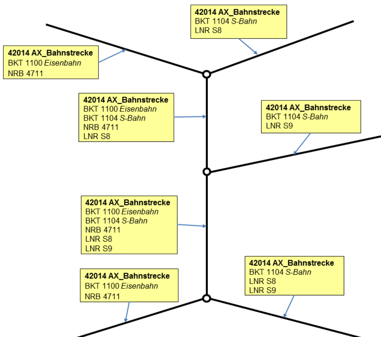
Abbildung 37: Modellierung von Bahnstrecken mit Strecken- und Liniennummern
