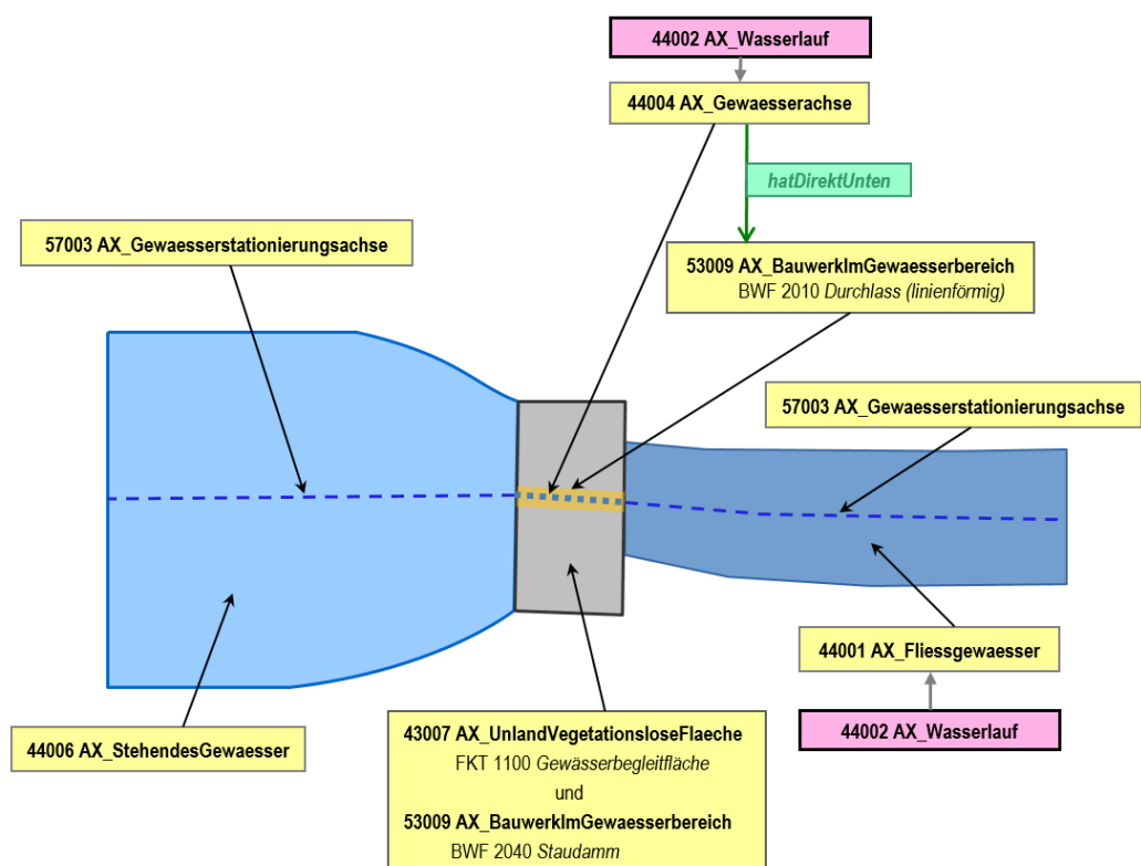
Abbildung 53: Modellierung von Wasserlauf unter Staudamm in linienförmigem Durchlass
