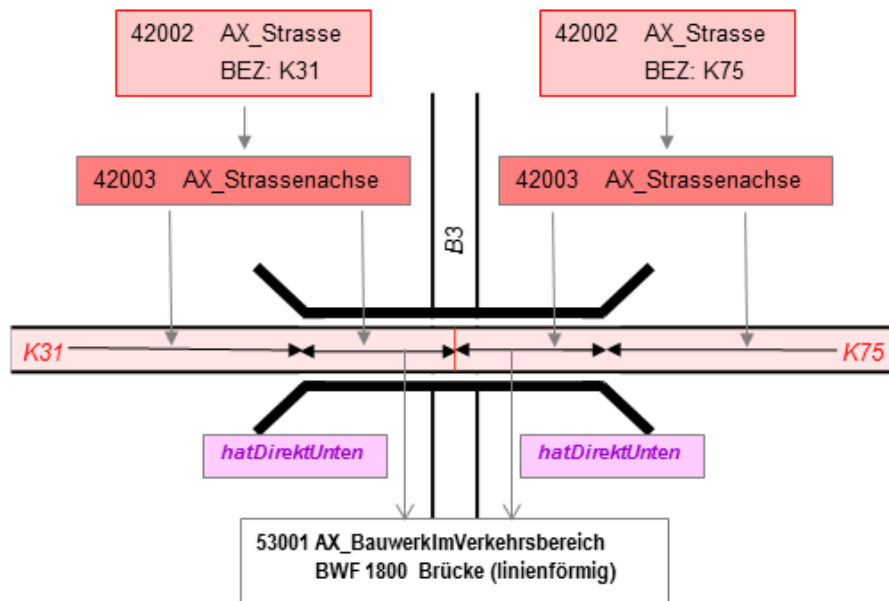
Abbildung 44: Modellierung einer linienförmigen Brücke
