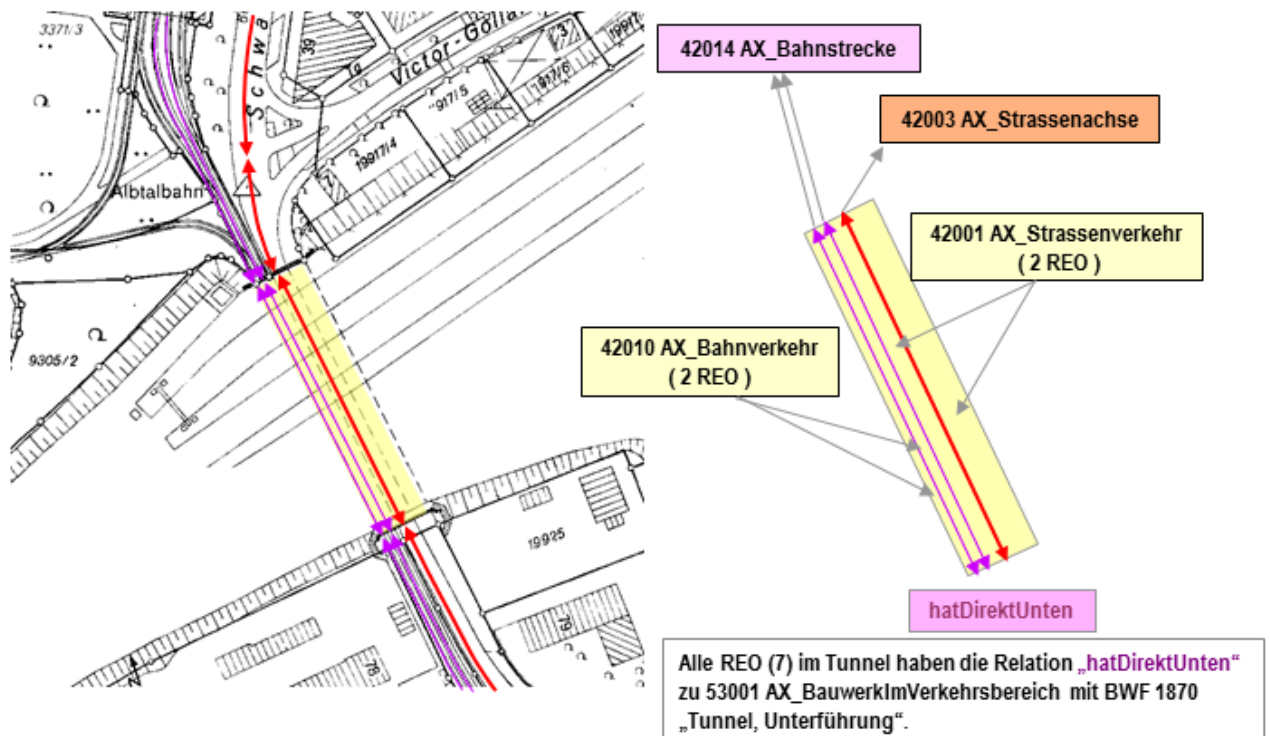
Abbildung 48: Modellierung eines flächenförmigen Tunnels mit mehreren Objekten
