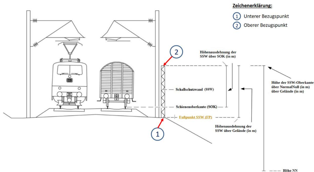
Abbildung 43: Höhenbezugspunkte für die Erhebung von Lärmschutzwänden (Quelle: Eisenbahn-Bundesamt, Referat 53, Datenmodell_Schallschutzwände_DB-fremde_Quellen_v2.0, Version 2.0, Stand: 07.08.2024)
