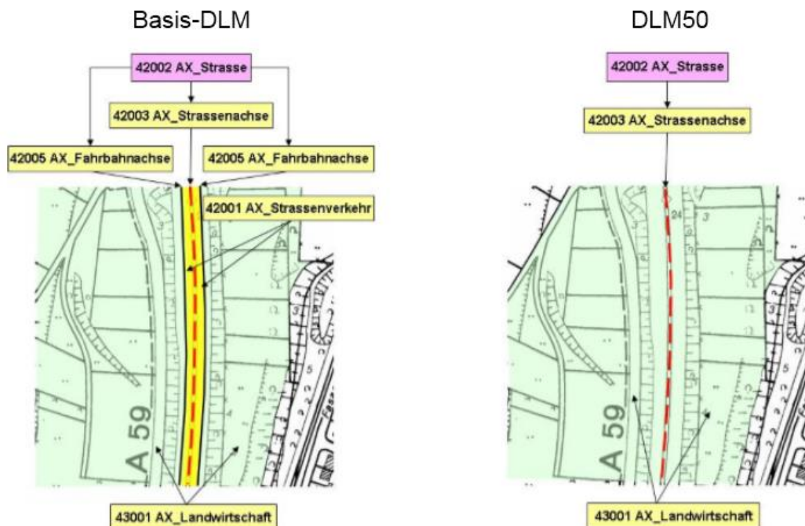
Abbildung 32: Modellierung einer Straße mit physisch getrennten Richtungsfahrbahnen im Basis-DLM und DLM50
