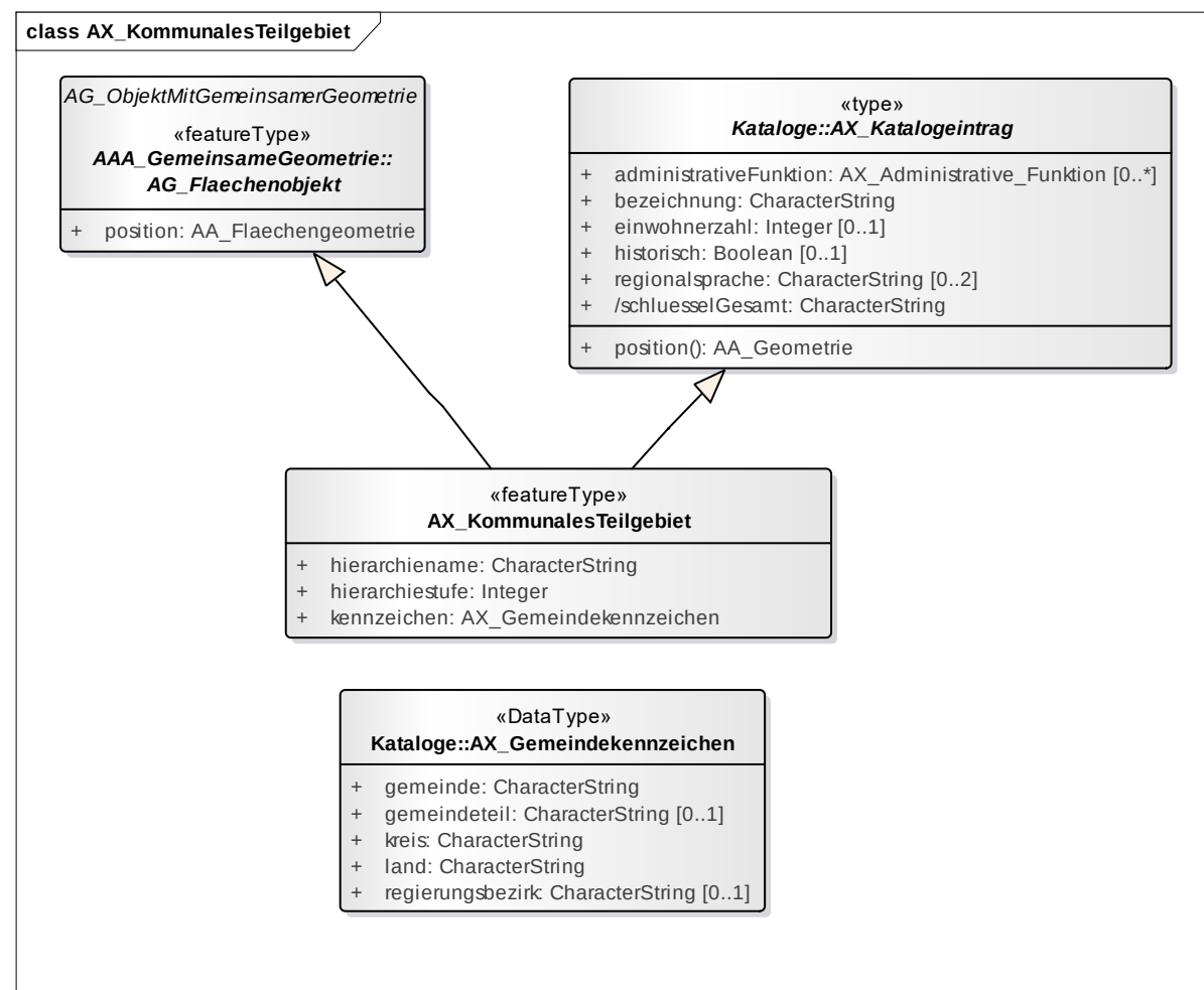
Abbildung 64: Klassendiagramm AX_KommunalesTeilgebiet
