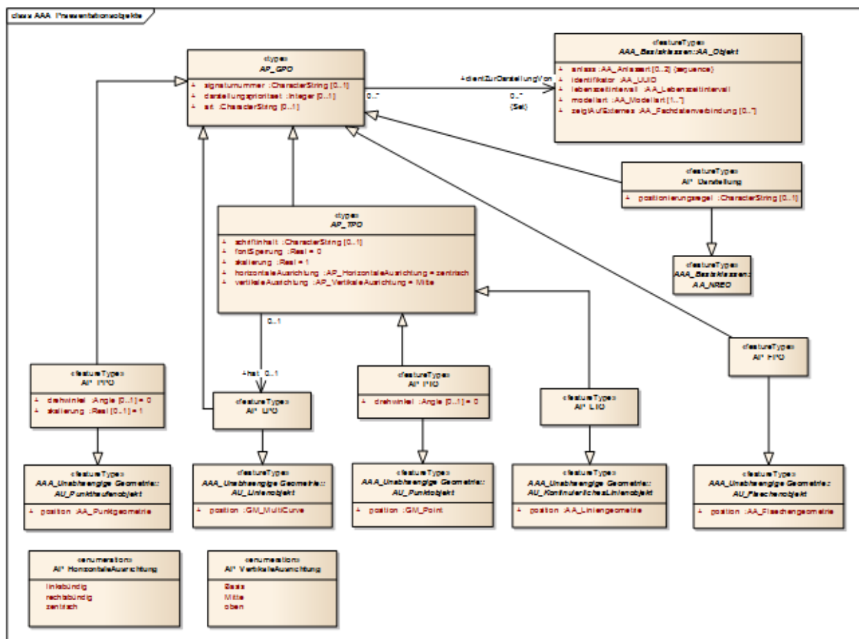
Abbildung 24: AAA-Präsentationsobjekte
