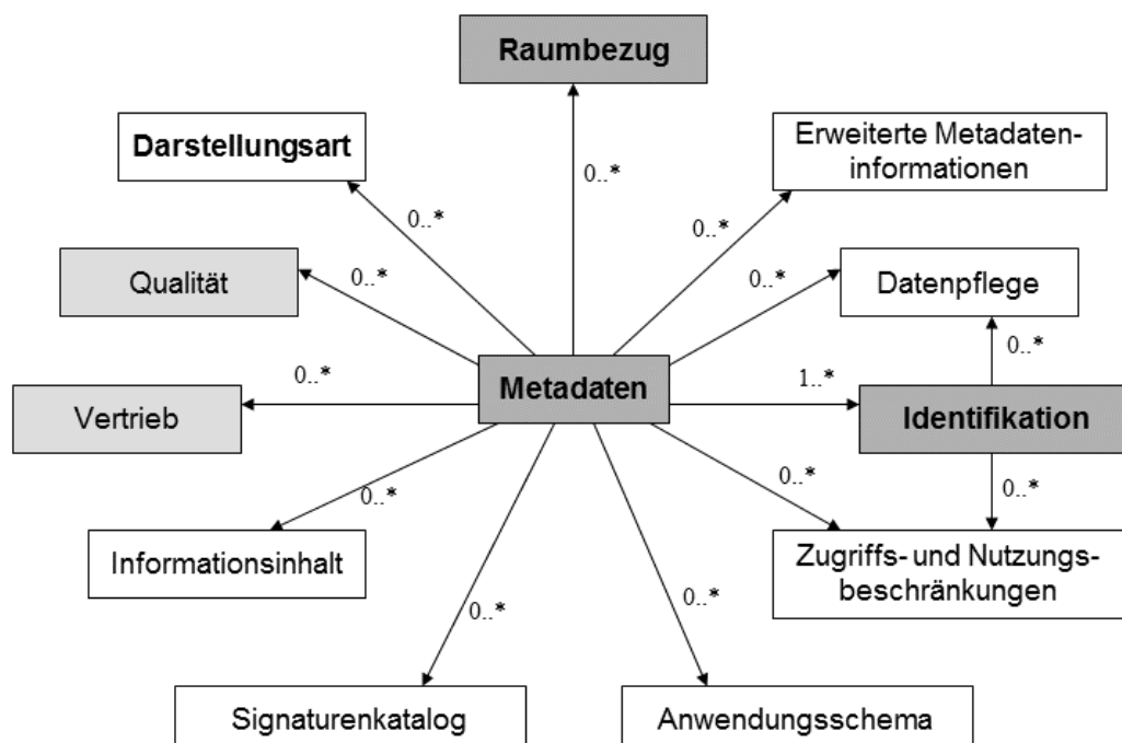
Abbildung 66: ISO-Hauptklassen
