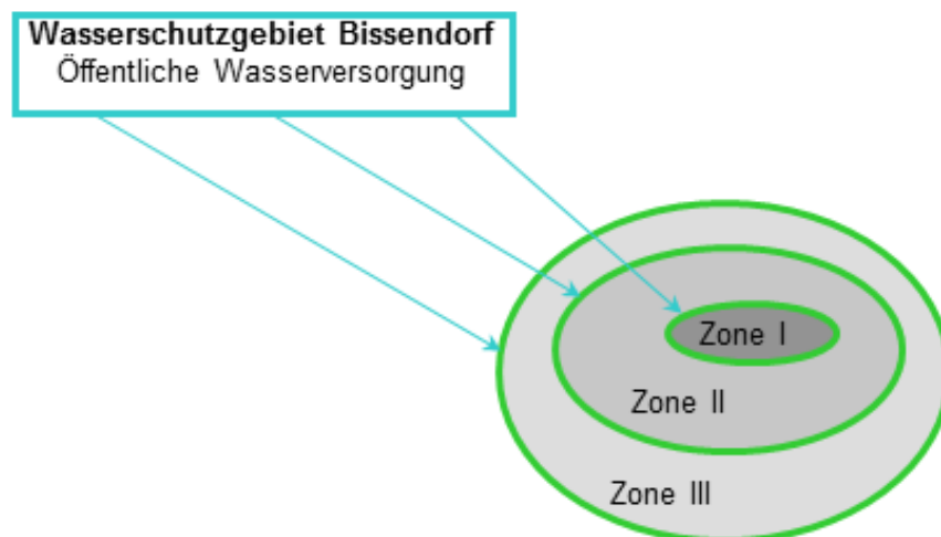
Abbildung 60: Beispiel „AX_SchutzgebietNachWasserrecht“
