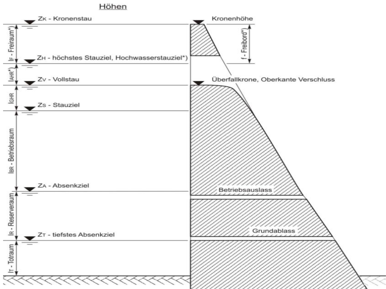
Abbildung 39: Schematische Darstellung der Stau- und Absenkziele bei einem Stausee
