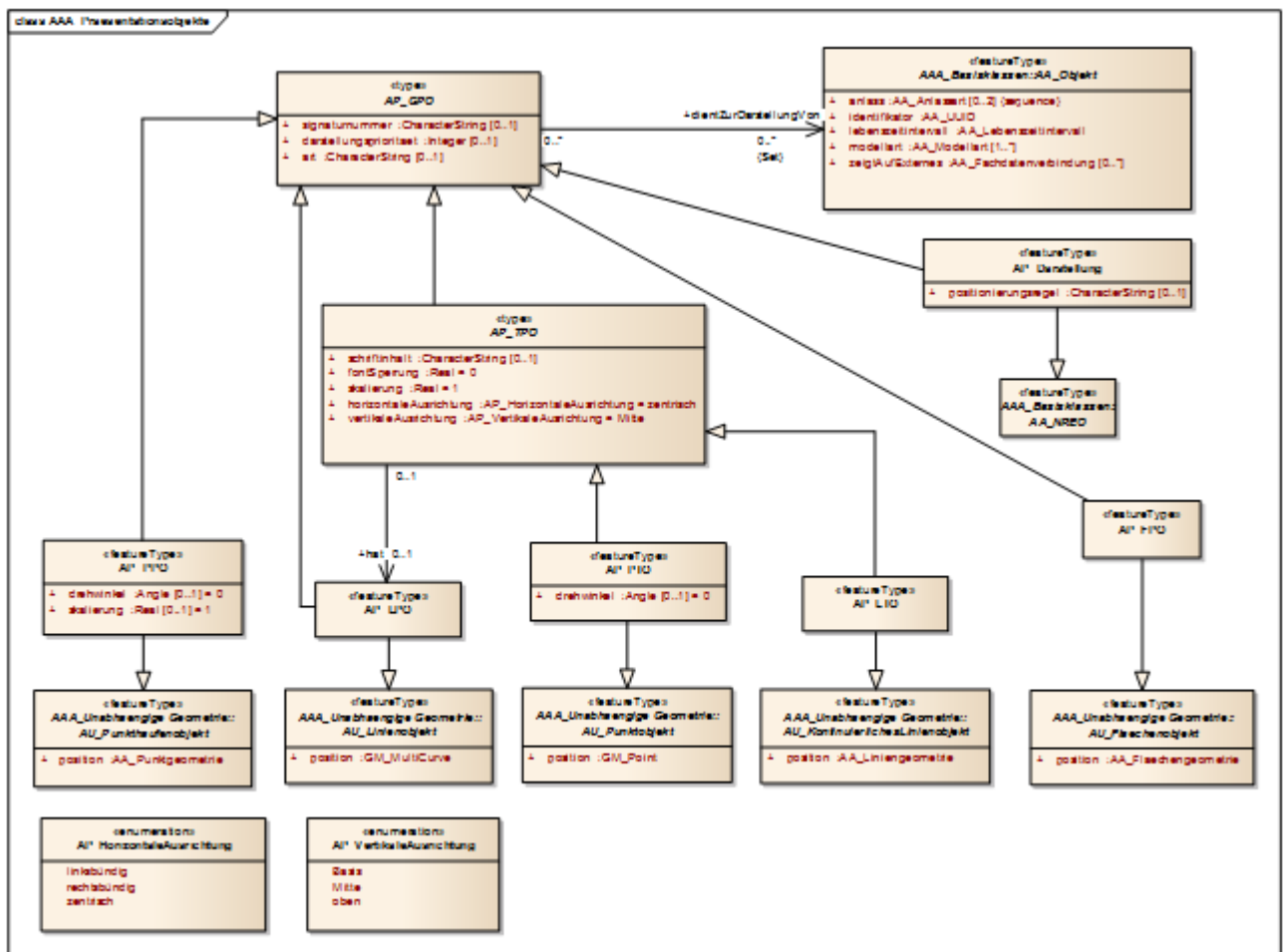
Abbildung 24: AAA-Präsentationsobjekte
