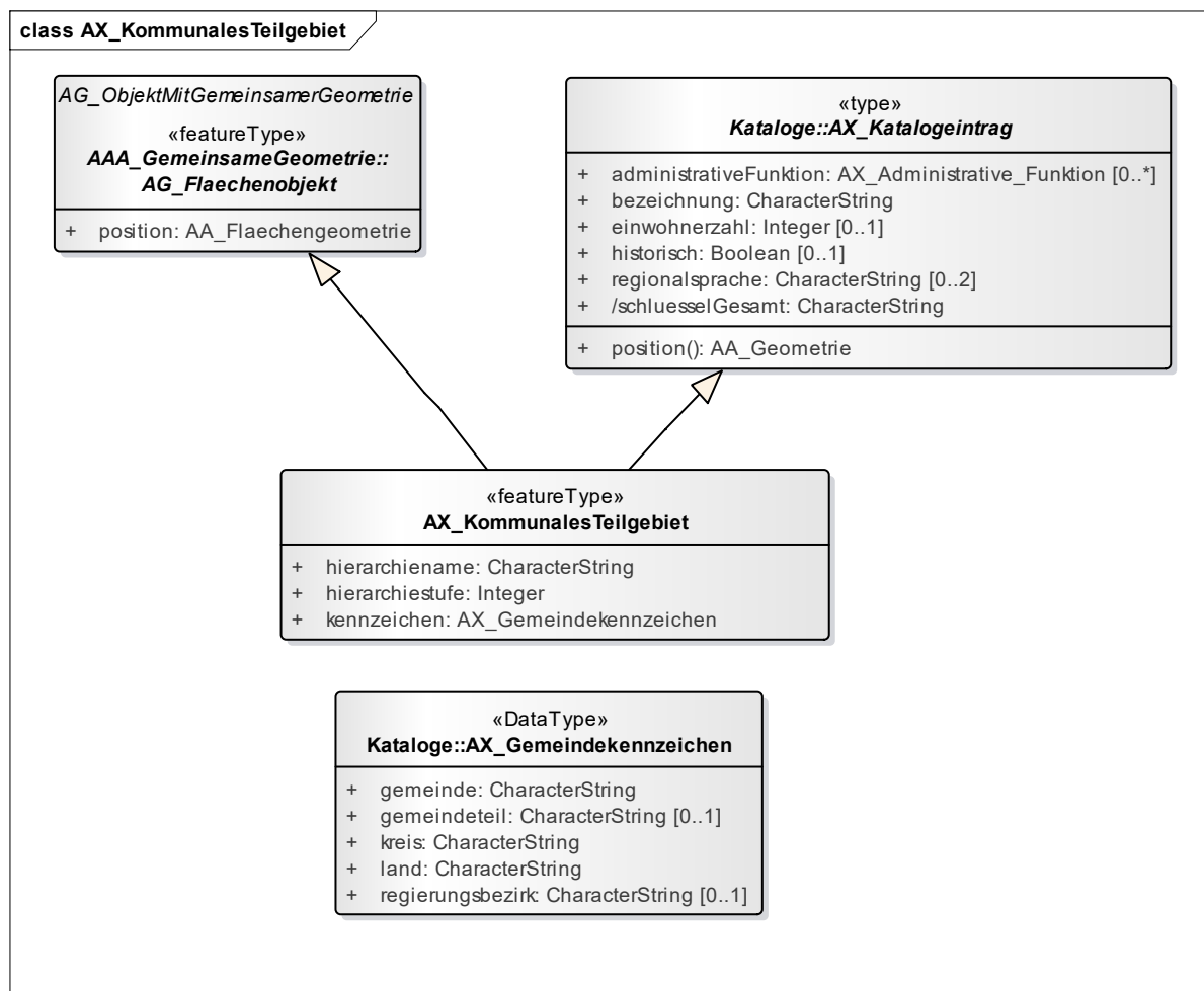
Abbildung 75: Klassendiagramm AX_KommunalesTeilgebiet
