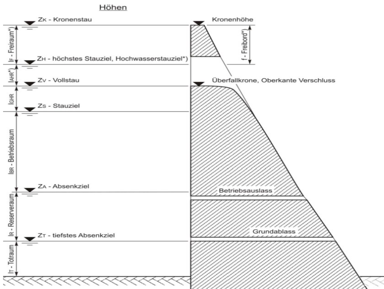
Abbildung 40: Schematische Darstellung der Stau- und Absenkeziele bei einem Stauee
