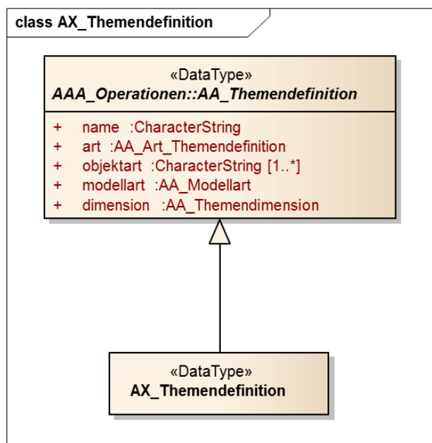
Abbildung 4: Klassendiagramm AX_Themendefinition
