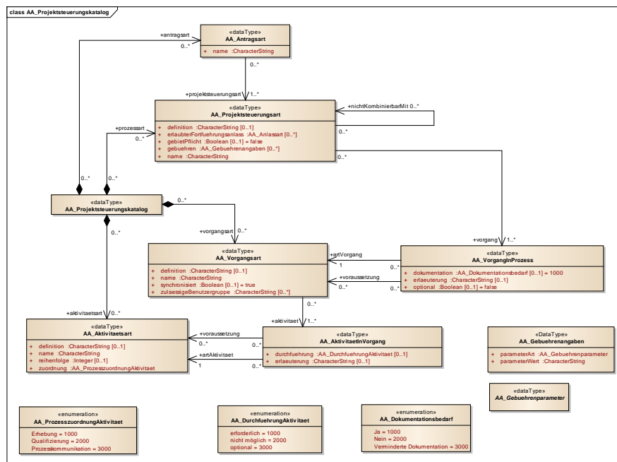
Abbildung 38: Klassendiagramm "AA_Projektsteuerungskatalog"
