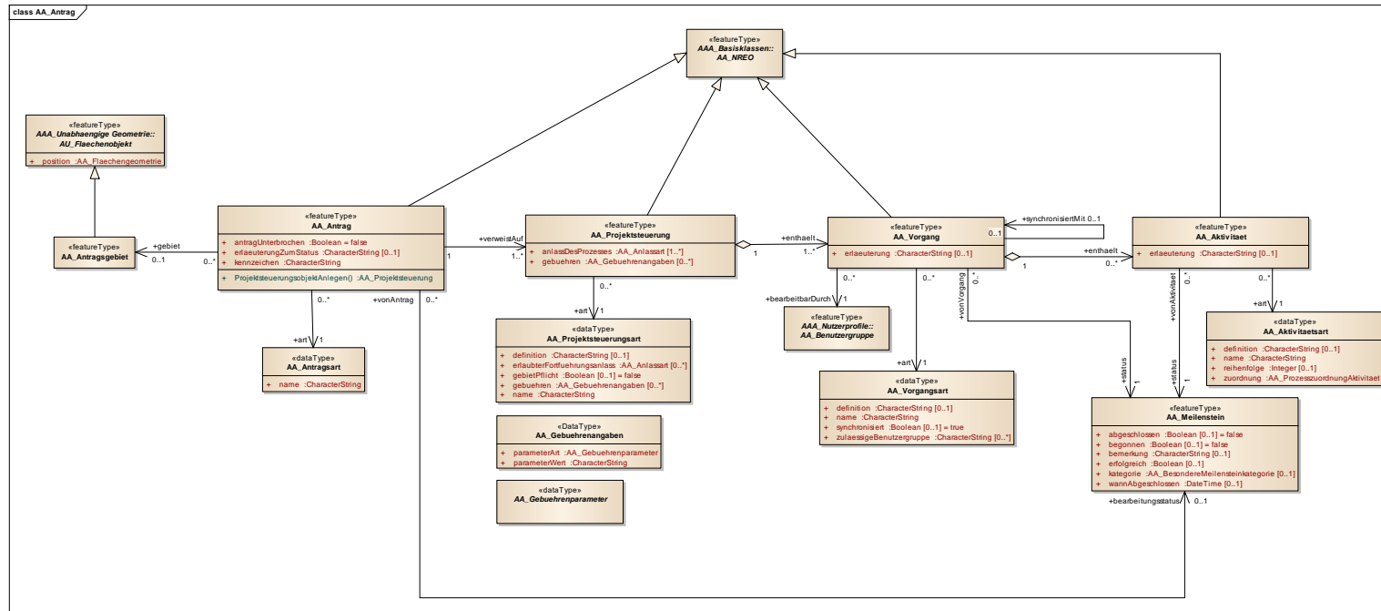
Abbildung 37: Klassendiagramm "AA_Antrag"
