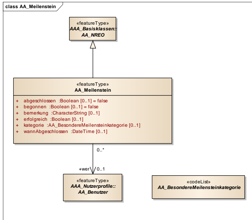
Abbildung 39: Klassendiagramm "AA_Meilenstein"
