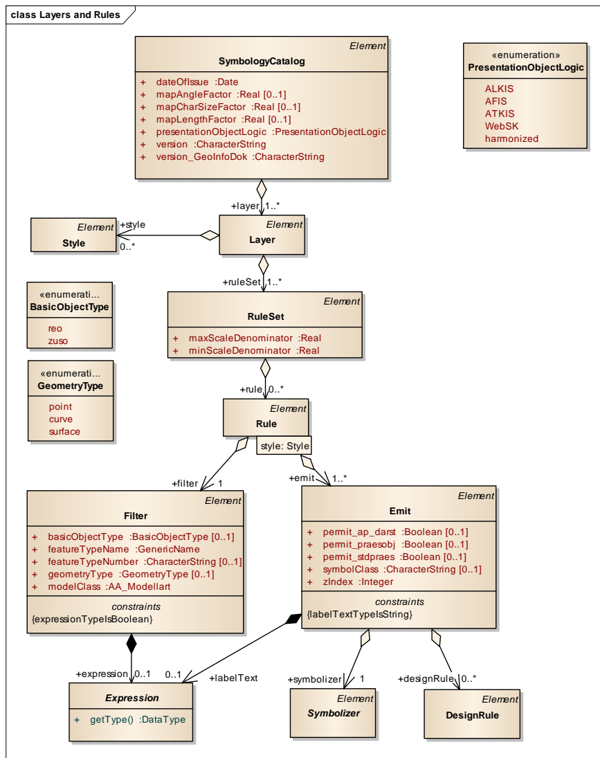
Abbildung 33: Schema SK-Objektmodell
