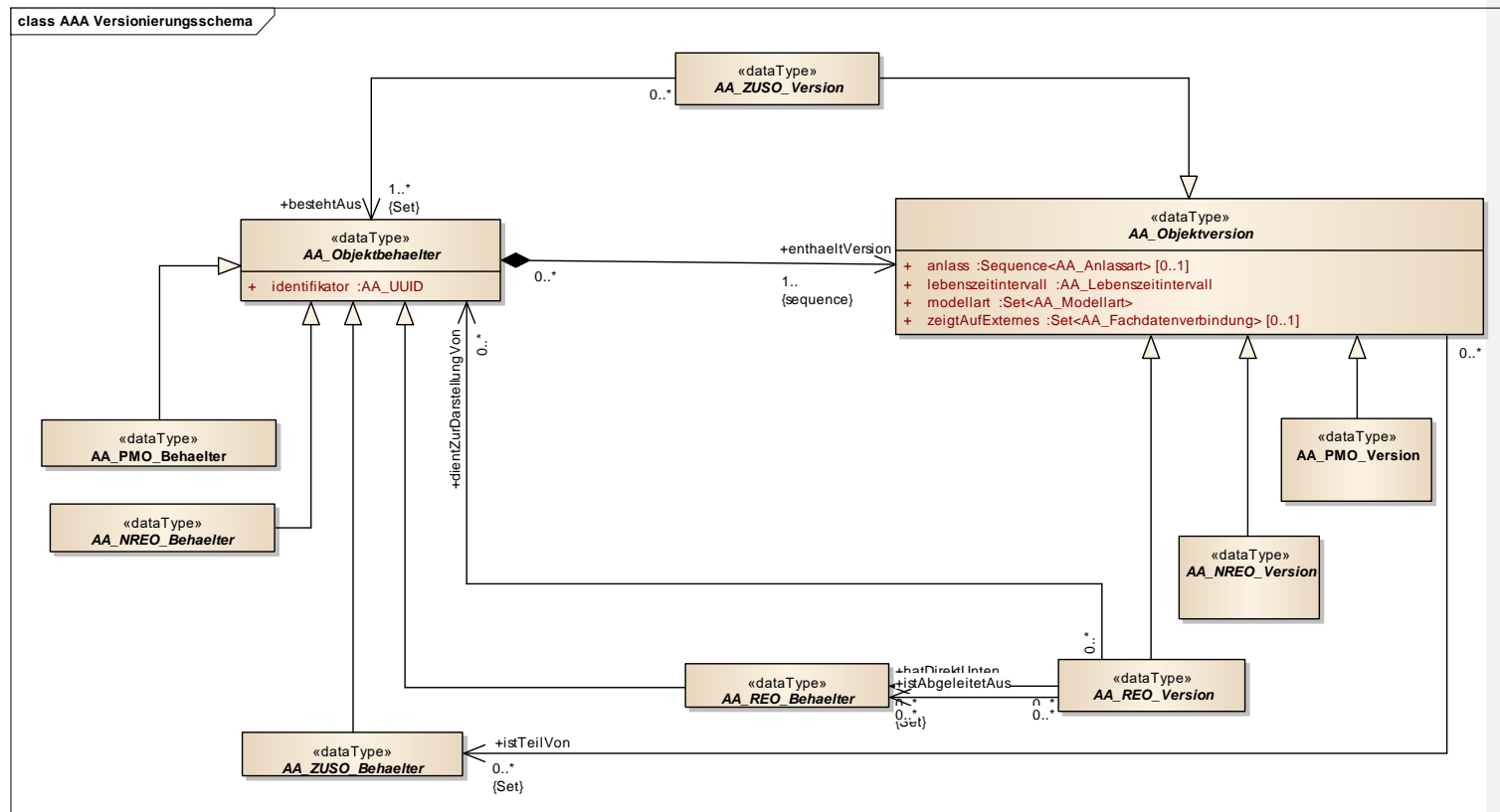
Abbildung 27: Versionierungsschema
