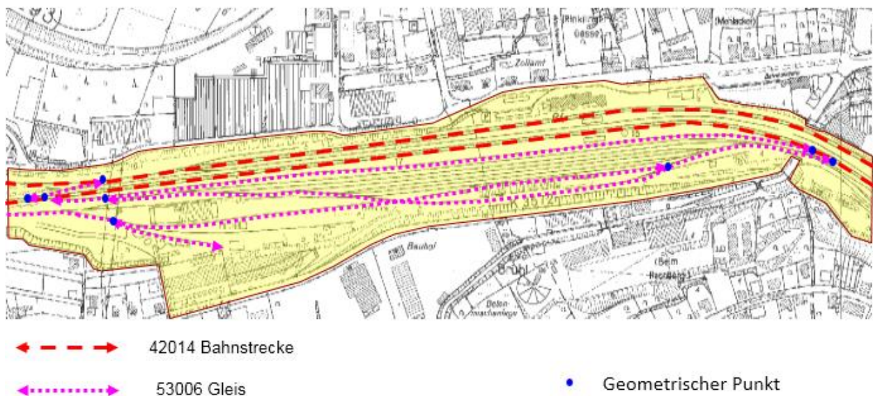
Abbildung 48: Modellierung von Gleisen
