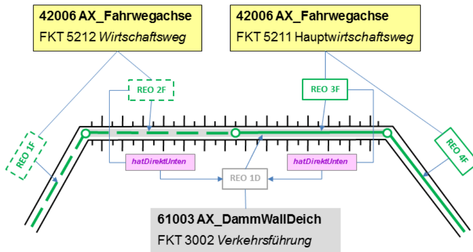
Abbildung 55: Modellierung eines linienförmigen Damms mit mehreren Fahrwegachsen
