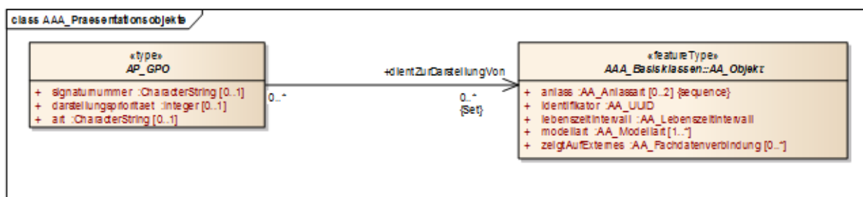
Abbildung 24: Auszug aus Basisschema, AP_GPO
