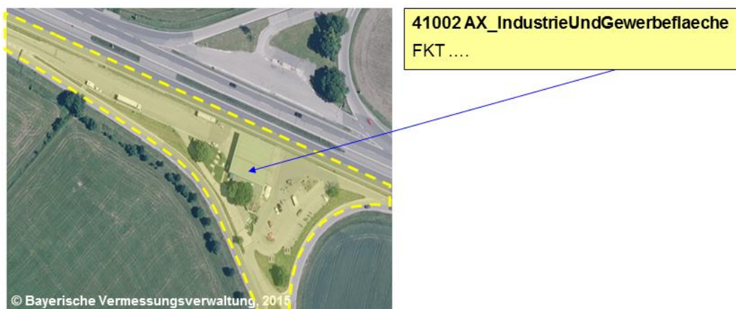
Abbildung 33: Modellierung einer Tankstelle
