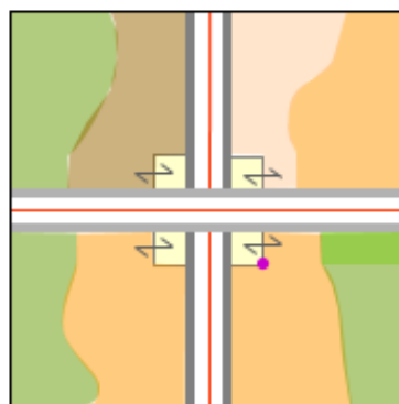
Abbildung 21: Flächenaufteilung bei Kreuzungen von physisch getrennten Straßen
