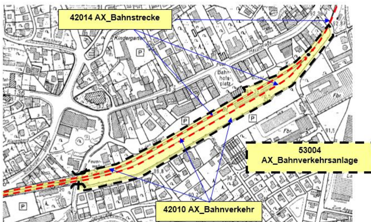
Abbildung 35: Modellierung mehrerer Bahnstrecken
