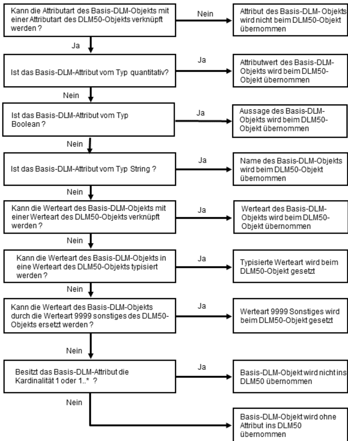
Abbildung 18: Entscheidungsbaum zur Überführung der Attribute
