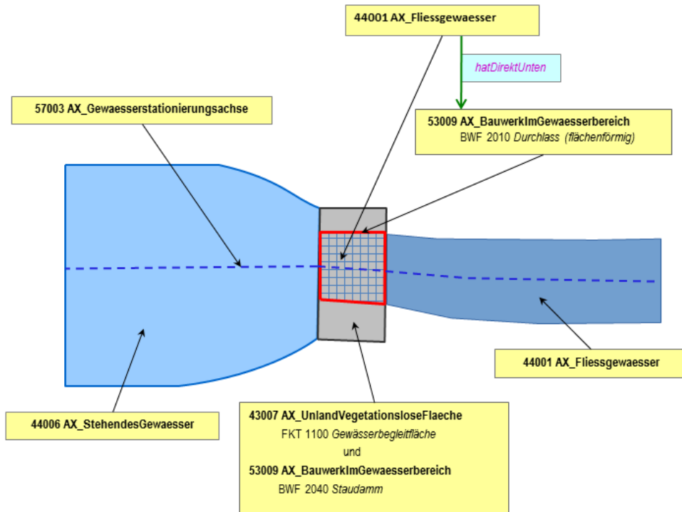
Abbildung 52: Modellierung von Wasserlauf unter Staudamm in flächenförmigem Durchlass
