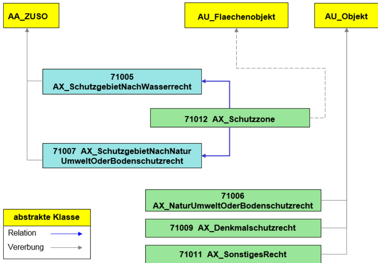
Abbildung 56: Öffentlich-rechtliche und sonstige Festlegungen
