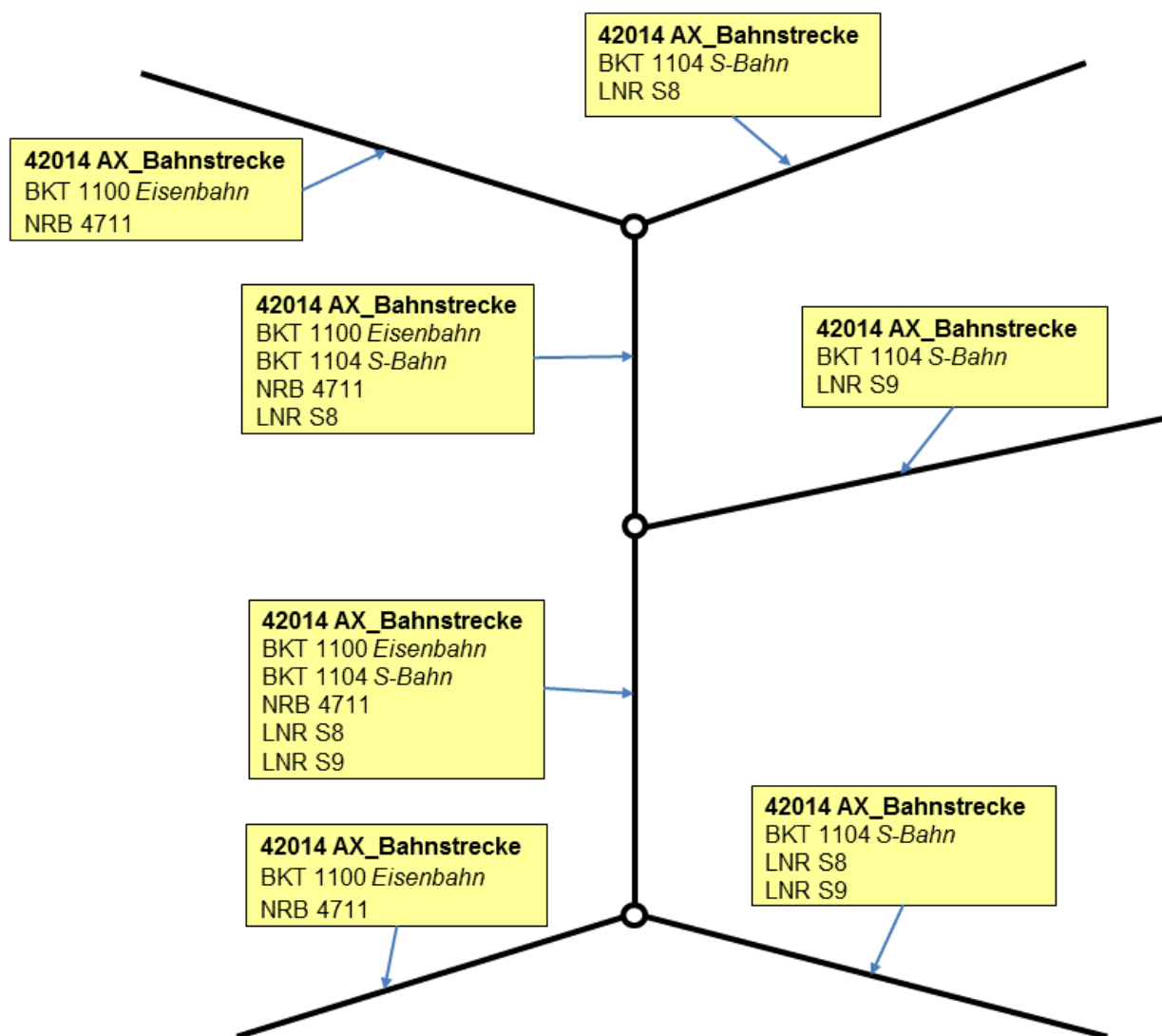
Abbildung 36: Modellierung von Bahnstrecken mit Strecken- und Liniennummern
