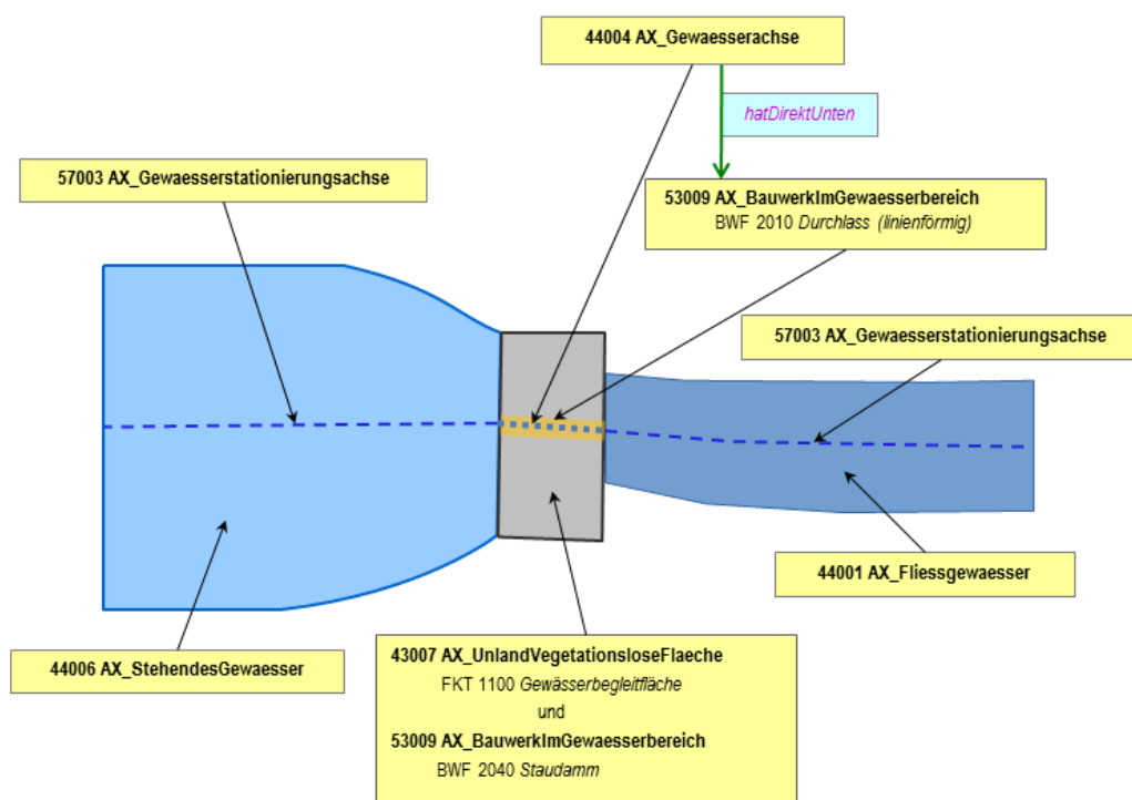
Abbildung 51: Modellierung von Wasserlauf unter Staudamm in linienförmigem Durchlass
