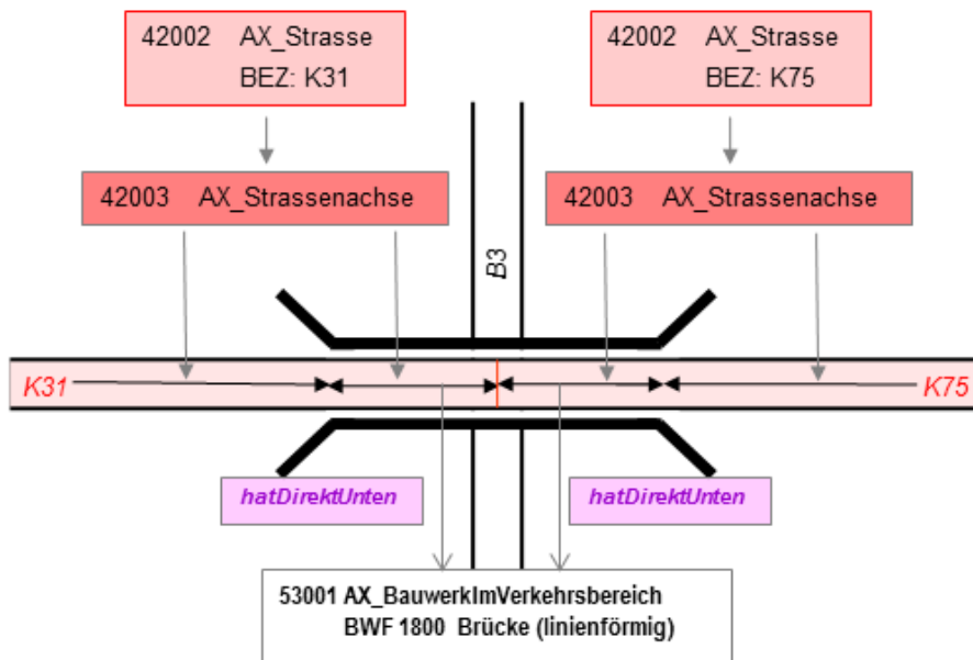
Abbildung 42: Modellierung einer linienförmigen Brücke
