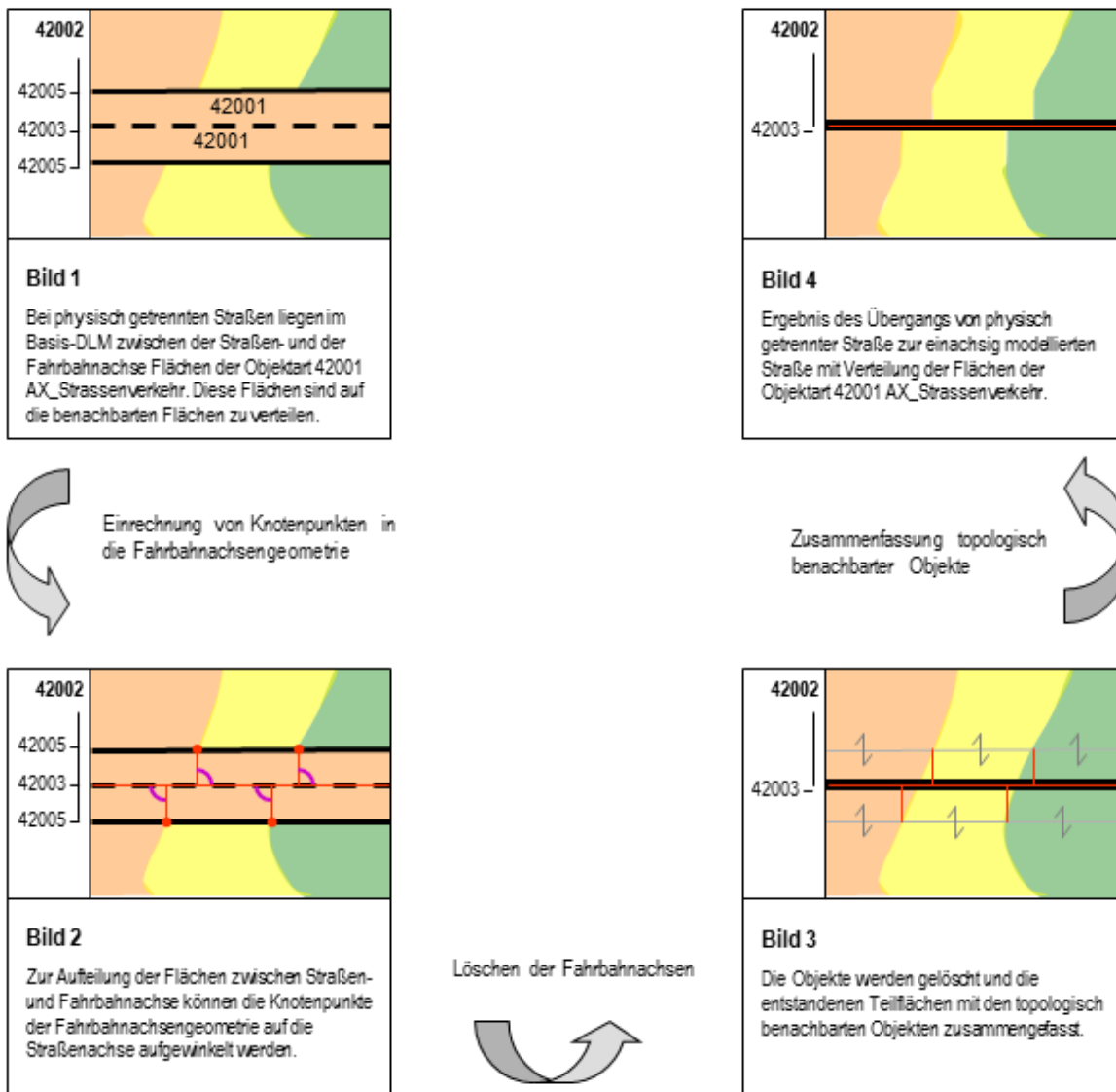
Abbildung 20: Flächenaufteilung beim Übergang von physisch getrennten zu einfach modellierten Straßen
