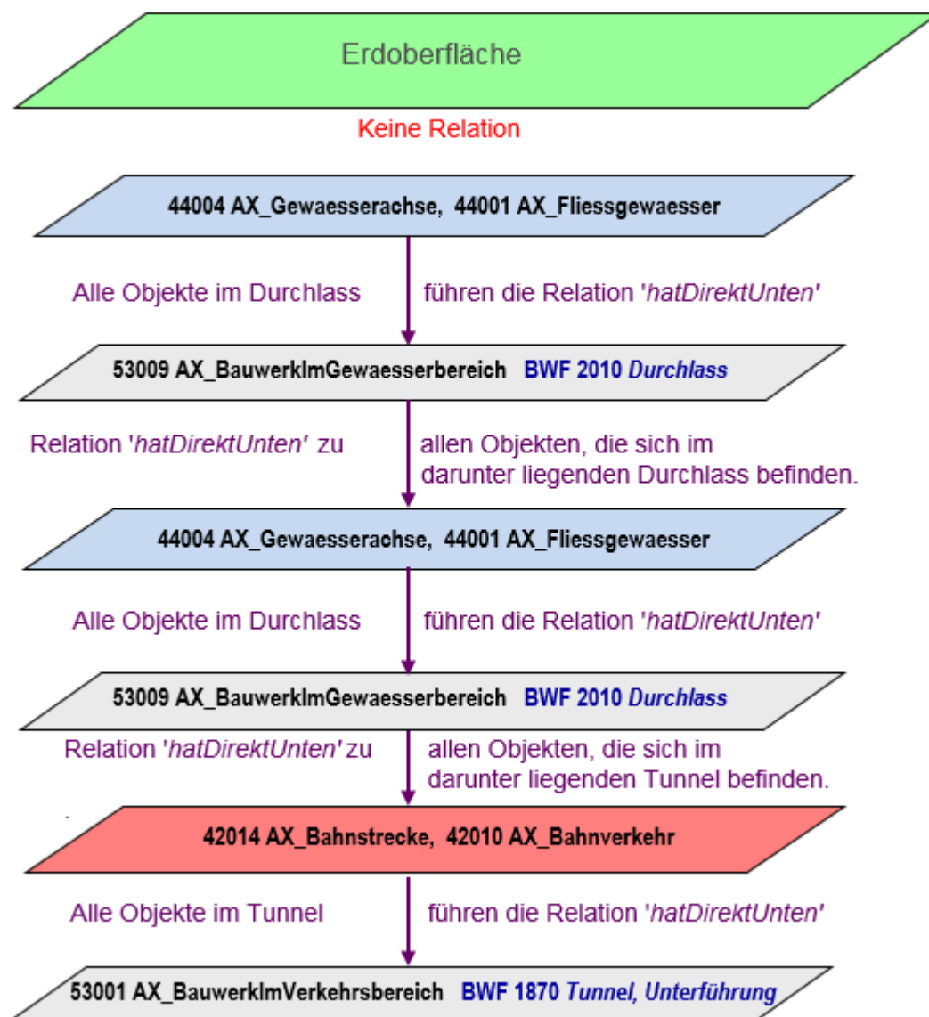
Abbildung 14: Vertikale Abbildung der Landschaft unter der Erdoberfläche
