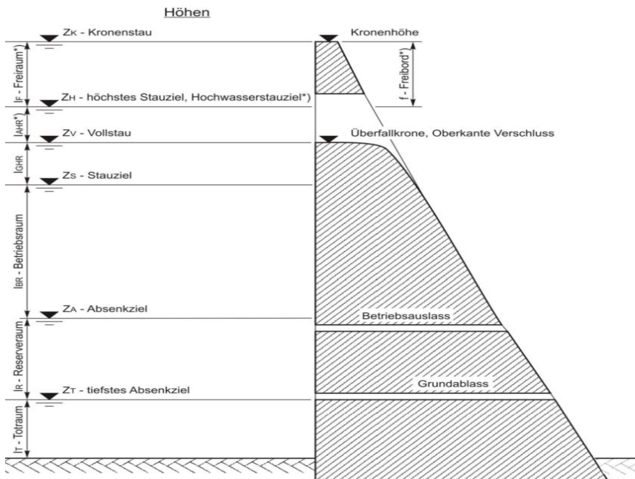
Abbildung 38: Schematische Darstellung der Stau- und Absenkziele bei einem Stauee
