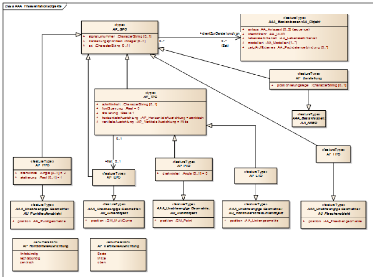
Abbildung 23: AAA-Präsentationsobjekte
