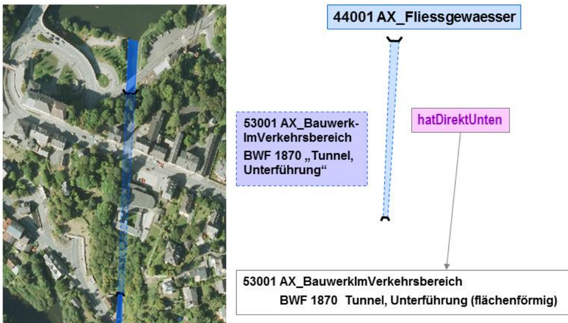
Abbildung 45: Modellierung eines flächenförmigen Tunnels mit einem flächenförmigen Objekt
