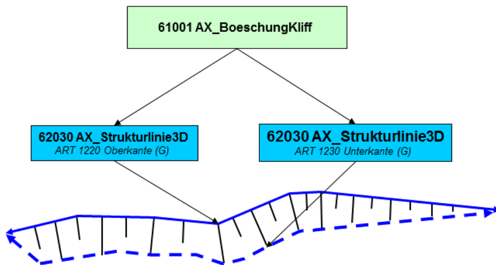
Abbildung 53: Modellierung einer Böschung mit Strukturlinien3D
