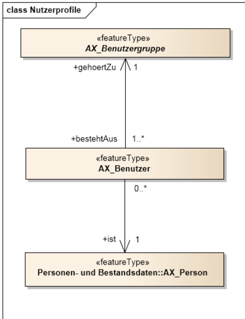
Abbildung 62: Objektartengruppe „Nutzerprofile“ in UML
