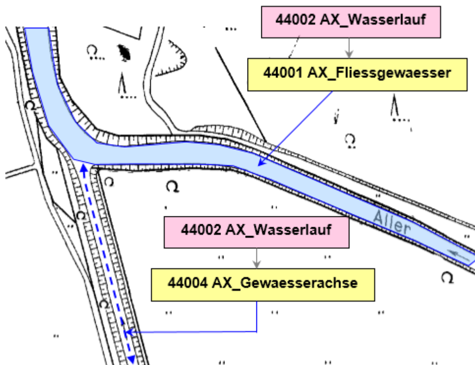
Abbildung 37: Modellierung von Wasserläufen
