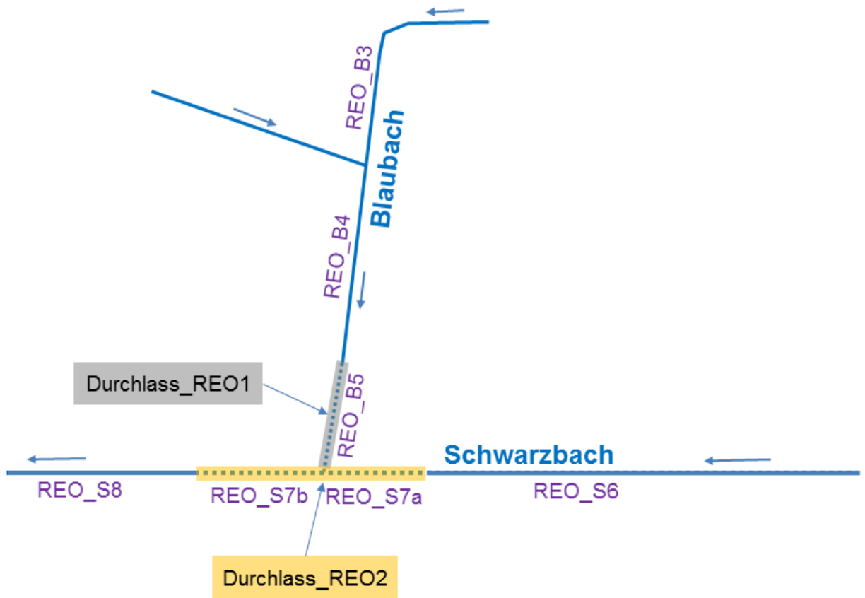
Abbildung 49: Modellierung eines linienförmigen Durchlasses
