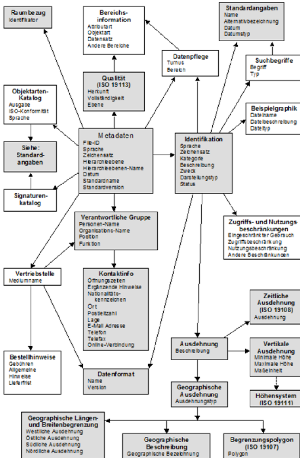
Abbildung 64: Übersicht der Metadatenelementarten
