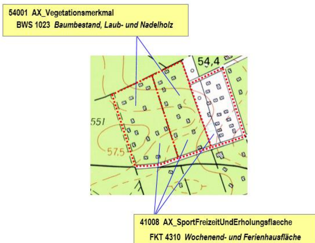
Abbildung 28: Beispiel für die Überlagerung einer Sport-, Freizeit- und Erholungsfläche mit Vegetation
