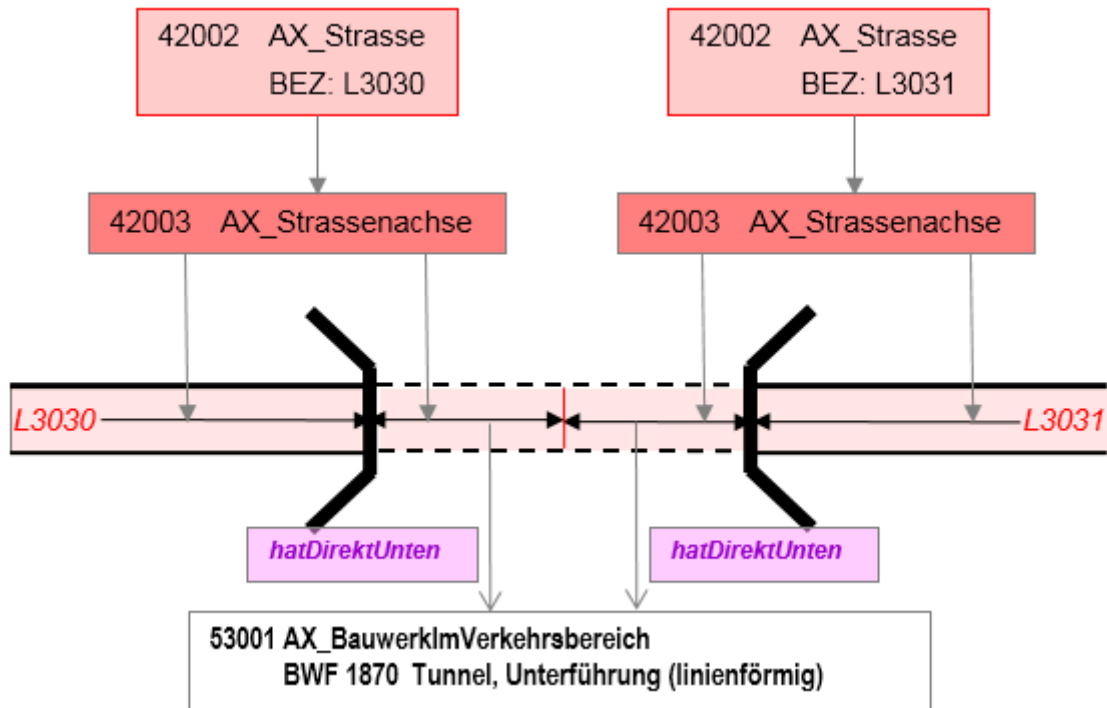
Abbildung 44: Modellierung eines linienförmigen Tunnels
