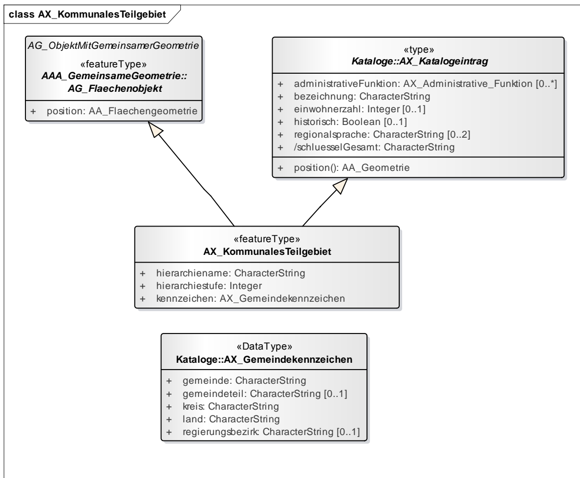
Abbildung 61: Klassendiagramm AX_KommunalesTeilgebiet
