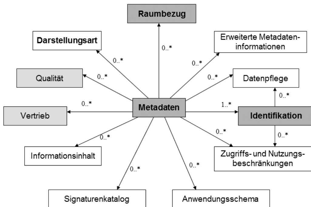
Abbildung 63: ISO-Hauptklassen
