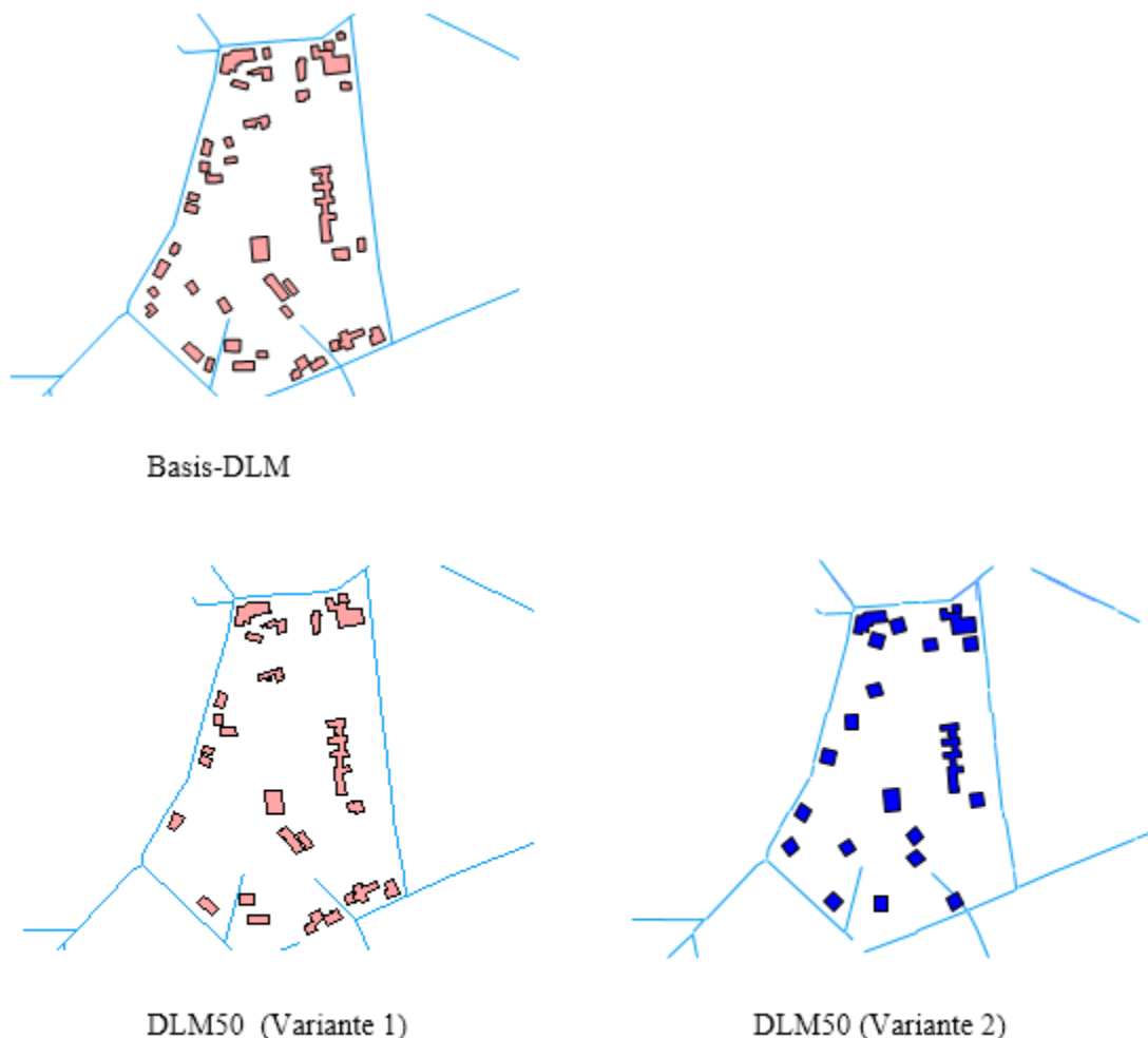
Abbildung 27: Gebäudebestand im Basis-DLM und Ergebnis der Generalisierung im DLM50 in beiden Herstellungsvarianten
