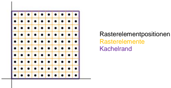
Abbildung 1: Schema der Anordnung von DOM Rasterelementen
