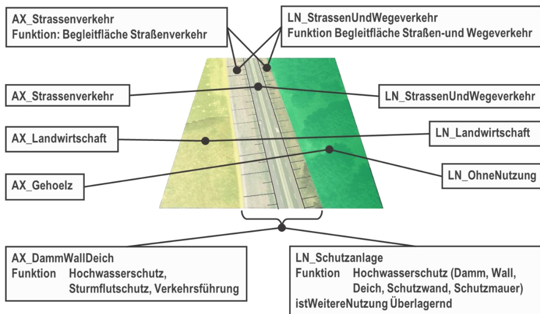
Abbildung 10: Modellierung einer Polderfläche
