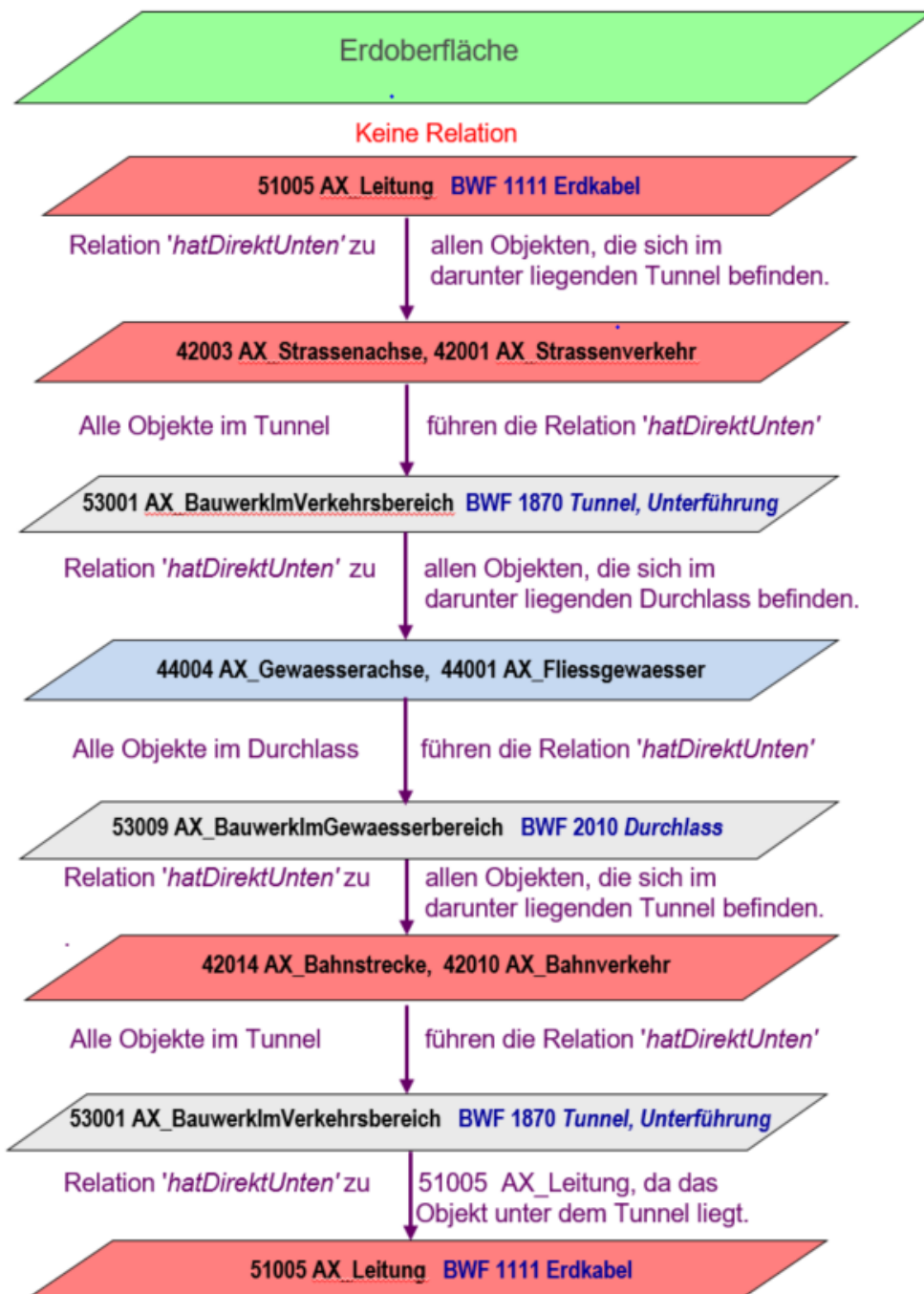
Abbildung 13: Vertikale Abbildung der Landschaft unter der Erdoberfläche
