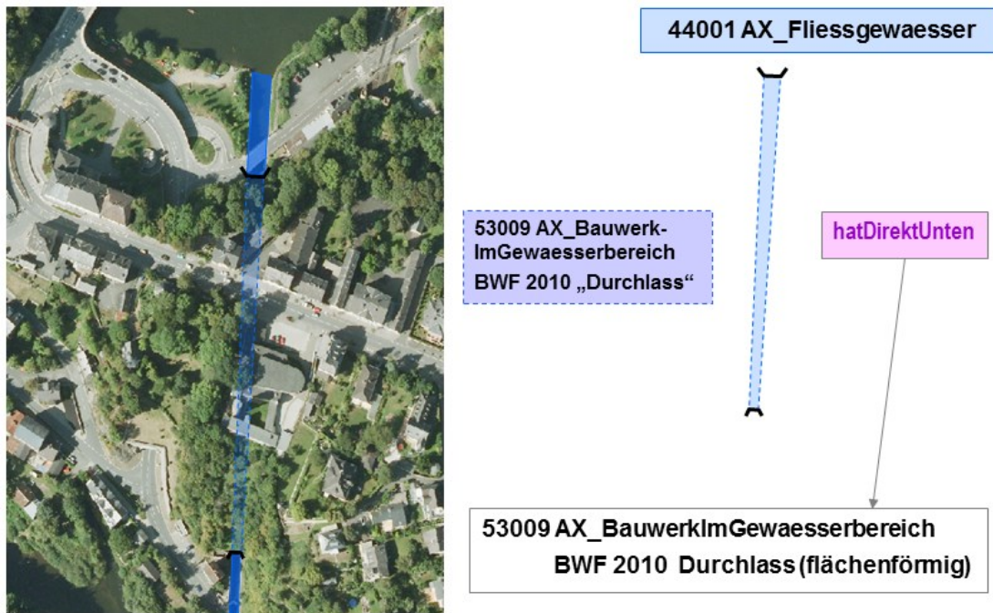
Abbildung 53: Modellierung eines flächenförmigen Durchlasses mit einem flächenförmigen Objekt
