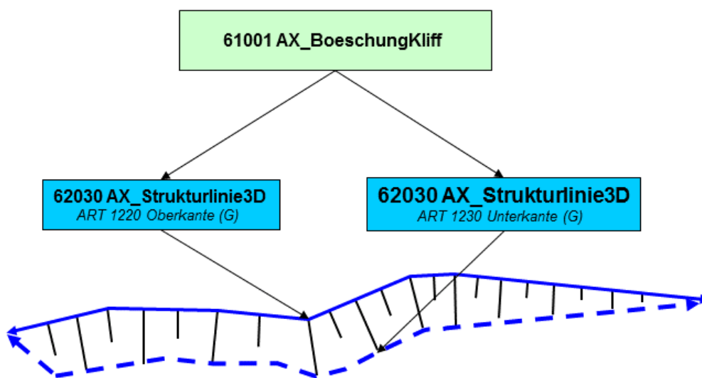
Abbildung 57: Modellierung einer Böschung mit Strukturlinien3D
