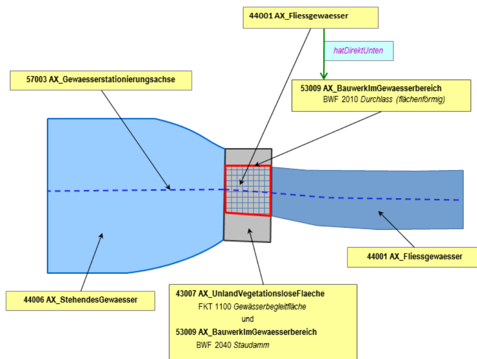
Abbildung 69: Modellierung von Wasserlauf unter Staudamm in flächenförmigem Durchlass
