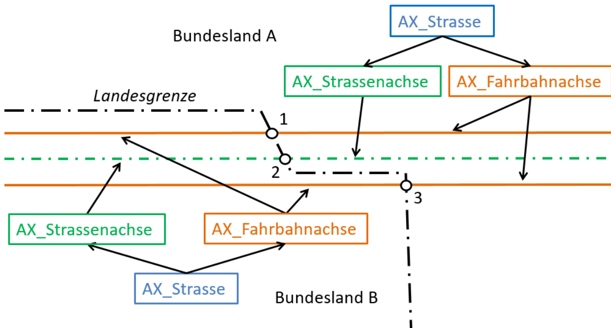
Abbildung 12: Beispiel für die Objektbildung einer komplex modellierten Straße im Bereich einer Landesgrenze
