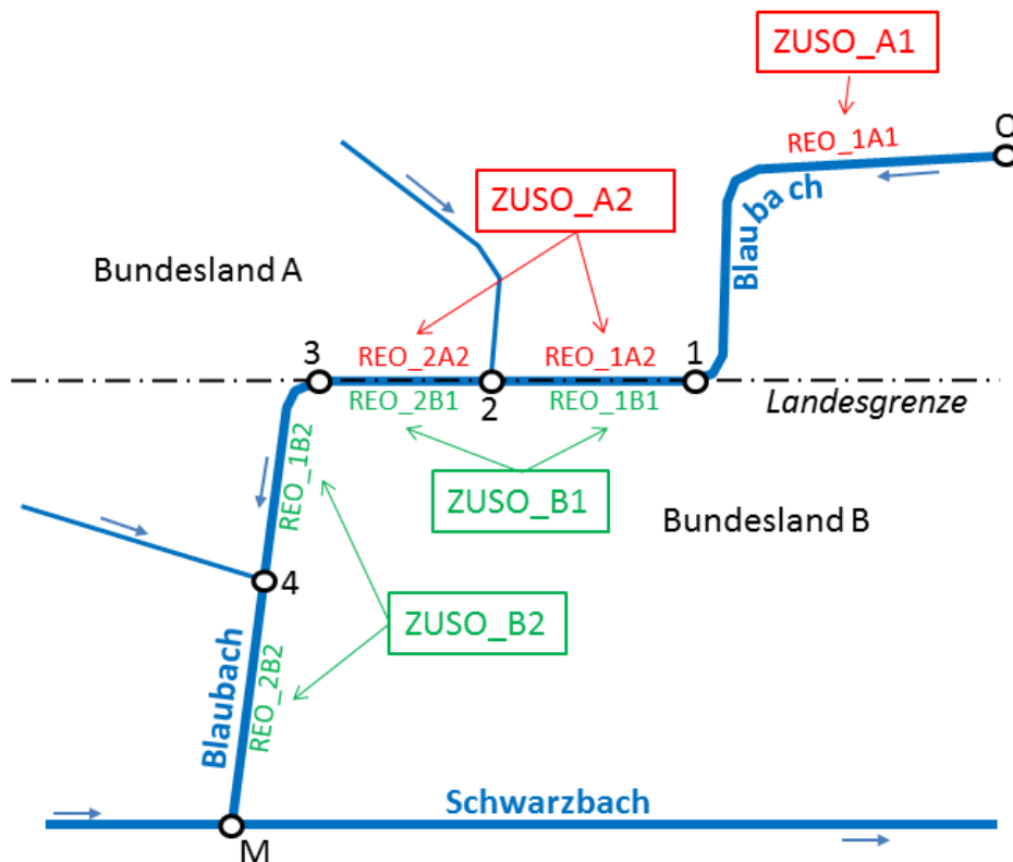
Abbildung 10: Beispiel eines linienförmigen Gewässers auf der Landesgrenze
