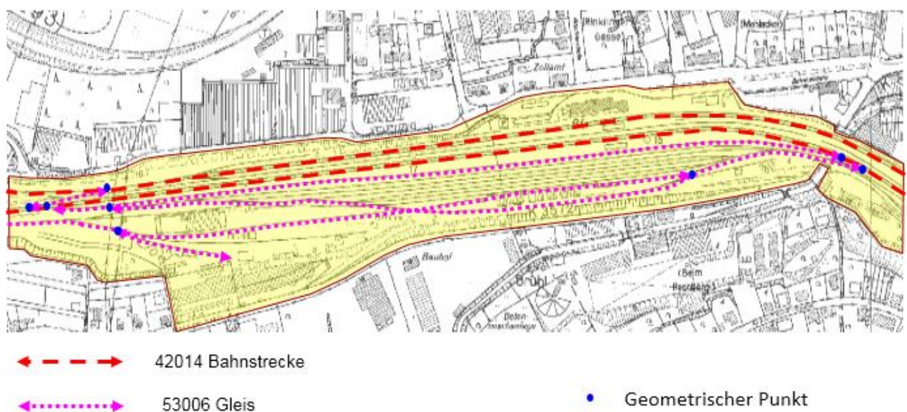
Abbildung 65: Modellierung von Gleisen
