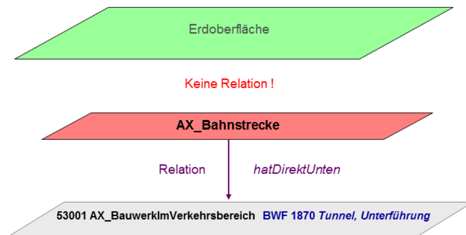
Abbildung 19: Vertikale Abbildung der Landschaft unter der Erdoberfläche
