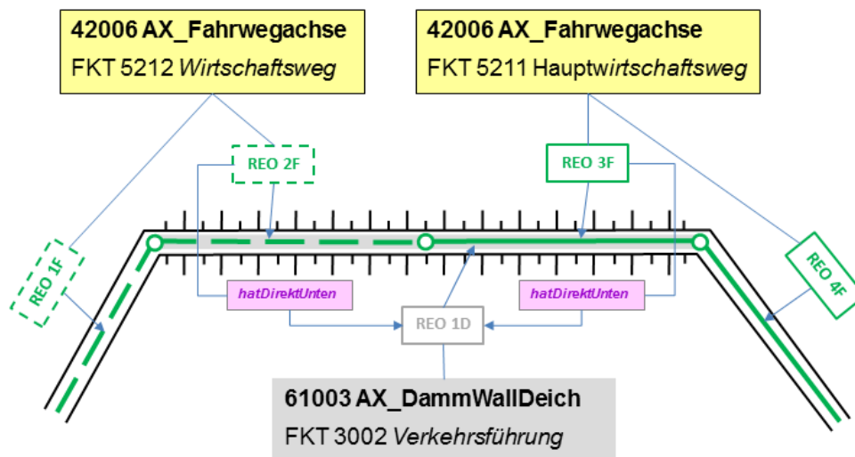
Abbildung 73: Modellierung eines linienförmigen Dammes mit mehreren Fahrwegachsen
