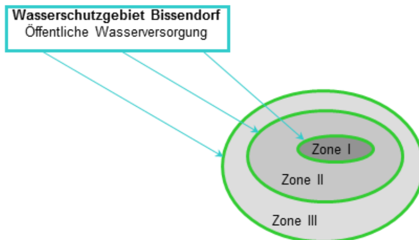
Abbildung 77: Beispiel „AX_SchutzgebietNachWasserrecht“
