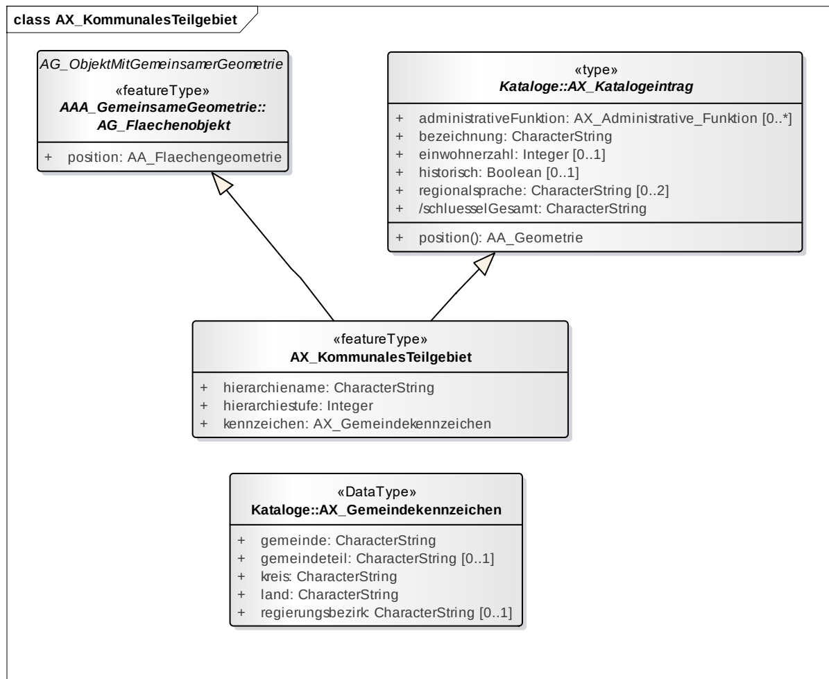
Abbildung 81: Klassendiagramm AX_KommunalesTeilgebiet
