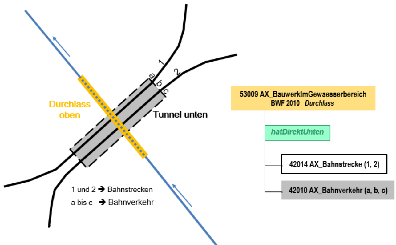
Abbildung 25: Vergabe der Relation „hatDirektUnten“ bei Durchlass über Tunnel
