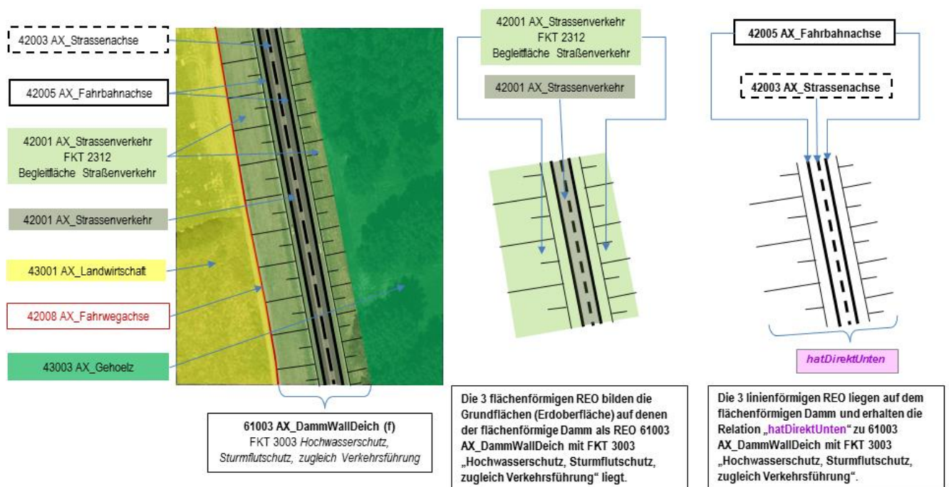
Abbildung 74: Modellierung eines flächenförmigen Dammes mit Straßen- und Fahrbahnachsen
