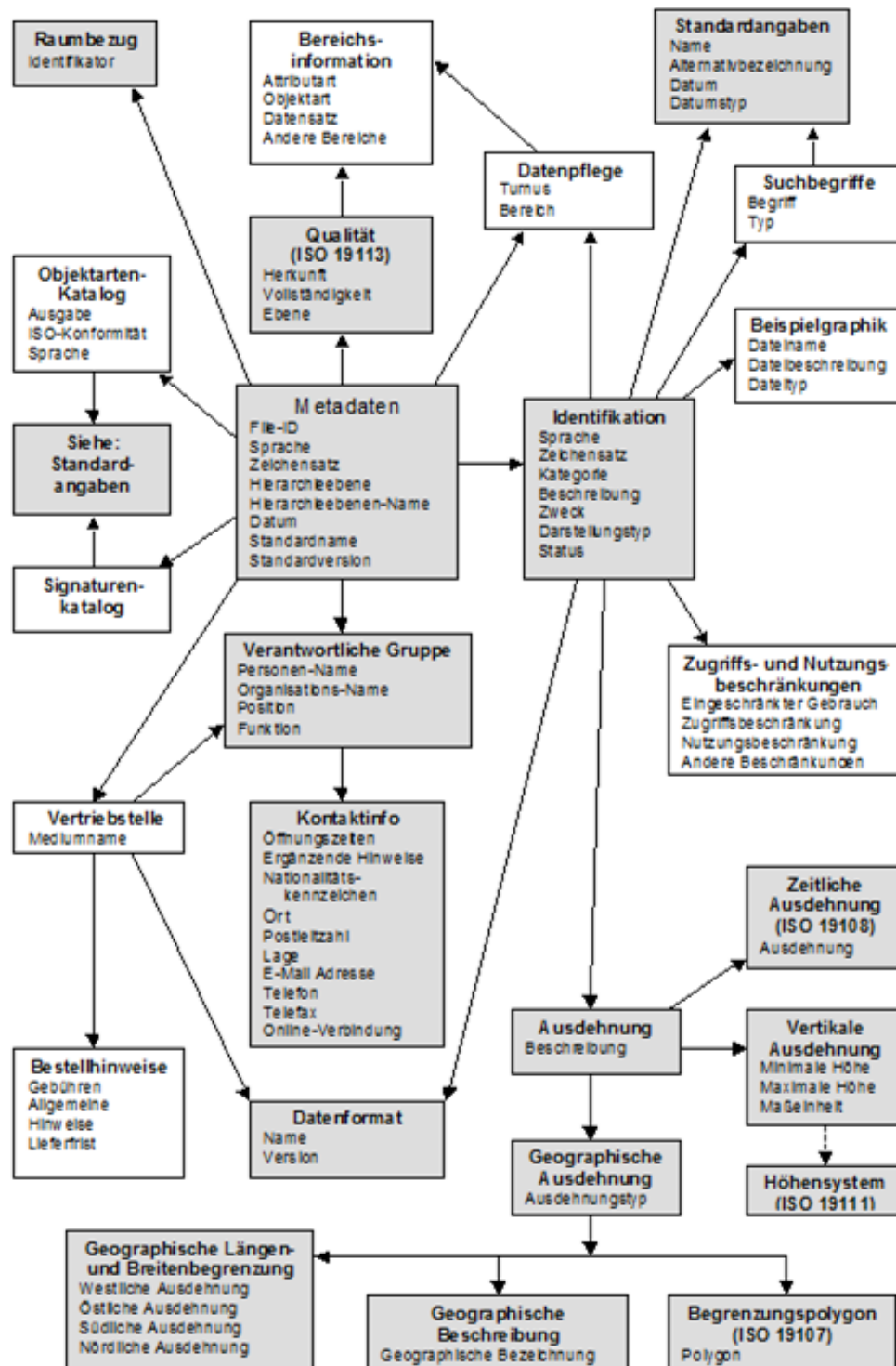
Abbildung 67: Übersicht der Metadatenelementarten
