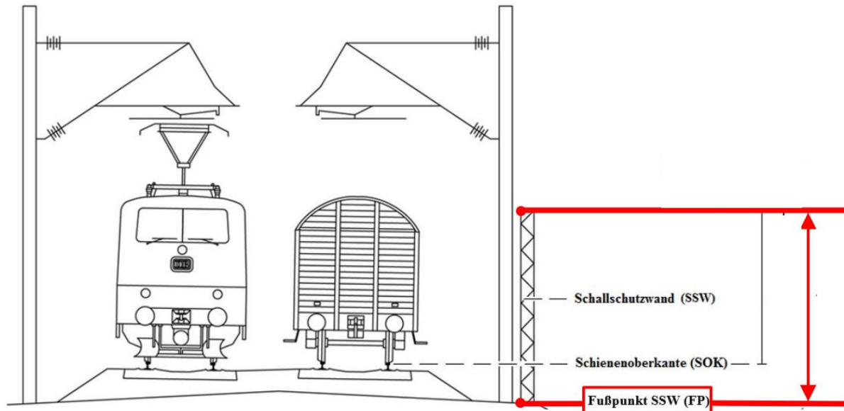
Abbildung 43: Höhenbezugspunkte für die Erhebung von Lärmschutzwänden
