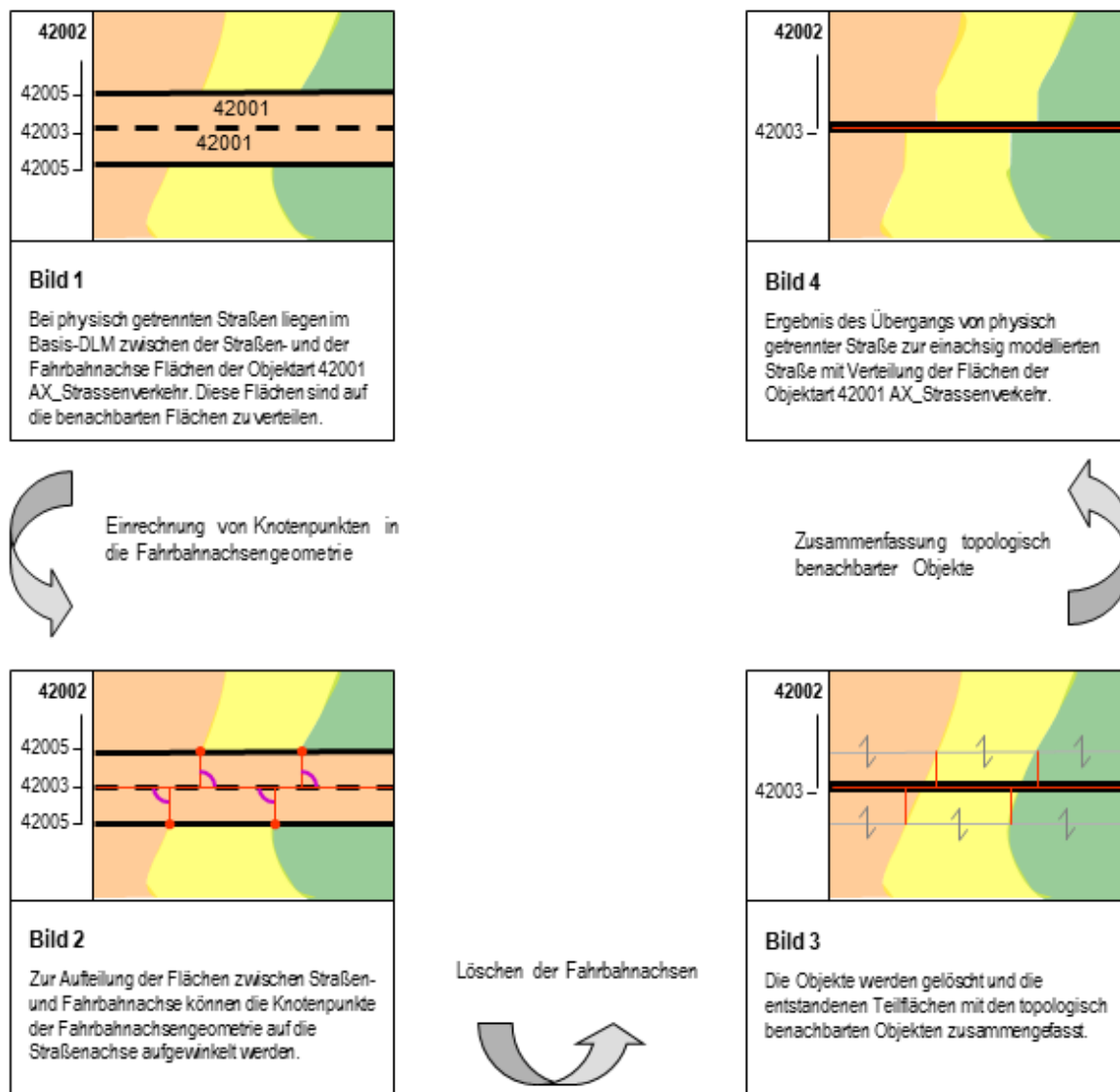
Abbildung 21: Flächenaufteilung beim Übergang von physisch getrennten zu einfach modellierten Straßen
