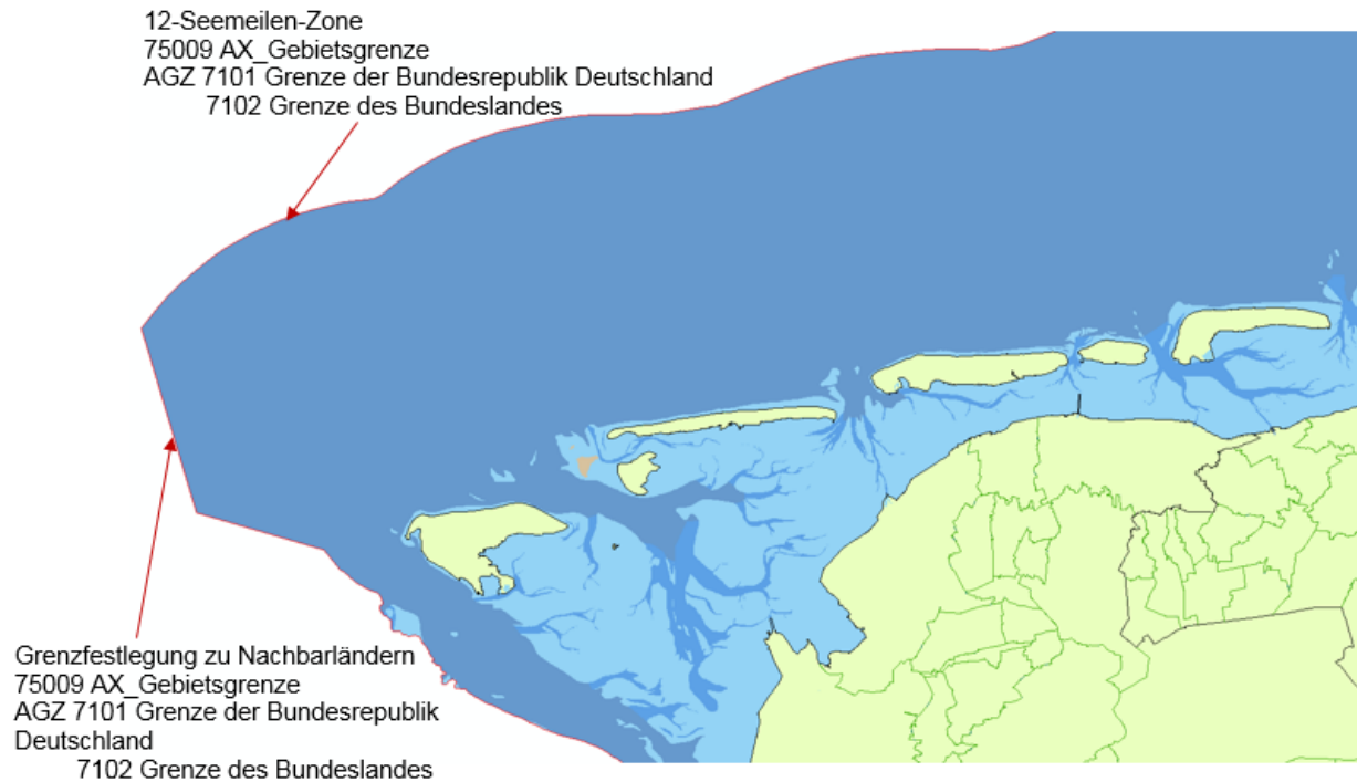
Abbildung 61: Grenzfestlegung in der Nordsee (Beispiel 1)
