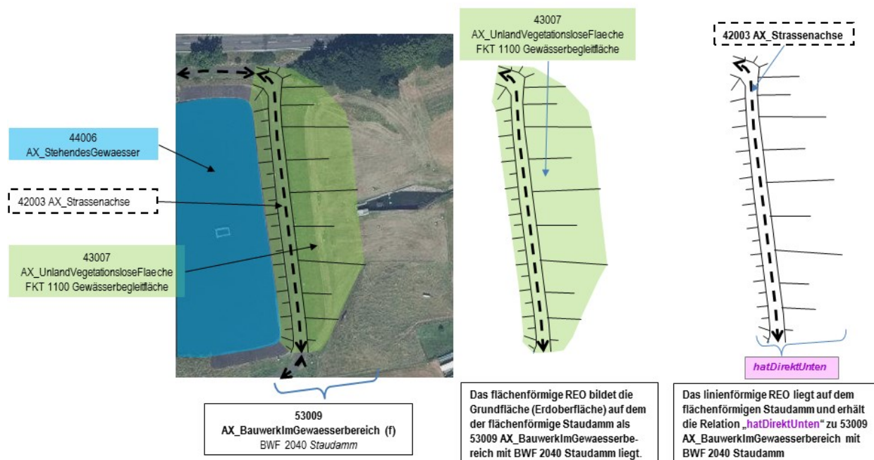
Abbildung 53: Modellierung eines REO Staudamm (flächenförmig) mit einer Straßenachse
