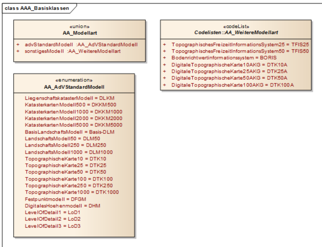
Abbildung 17: Modellarten im Basisschema
