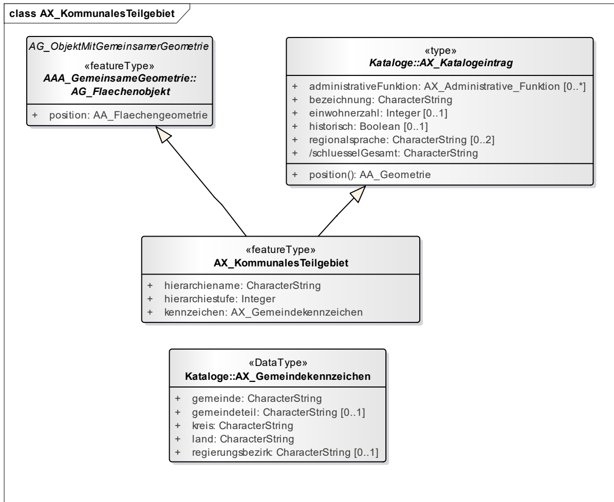
Abbildung 62: Klassendiagramm AX_KommunalesTeilgebiet
