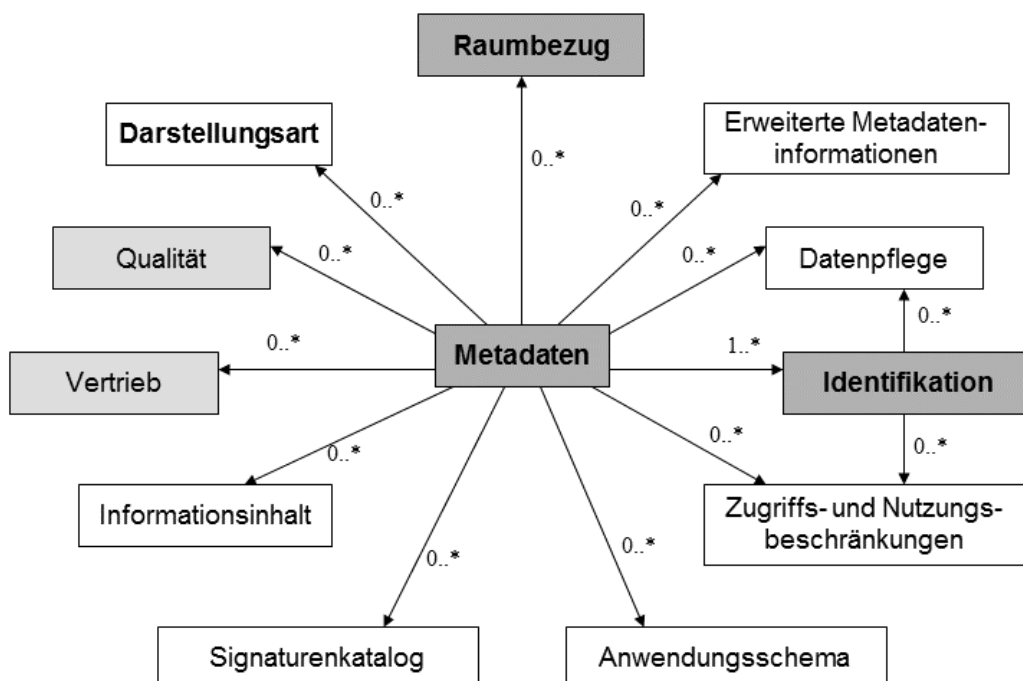
Abbildung 64: ISO-Hauptklassen
