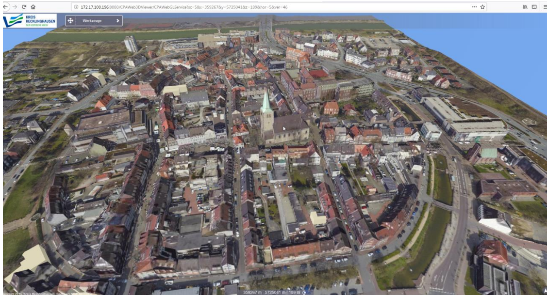
Ausschnitt aus Stadtmodell Kreis Recklinghausen volltexturiert automatisch erstellt aus Schrägluftbildern
