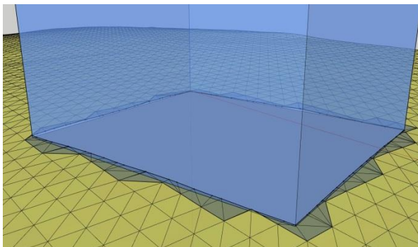
TerrainIntersectionCurve (TIC) auf der Basis des DGM1 gerechnet.
