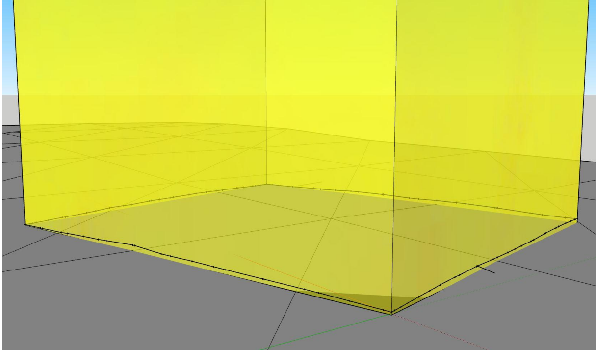
TerrainIntersectionCurve (TIC) aus DGM1 mit DGM10
